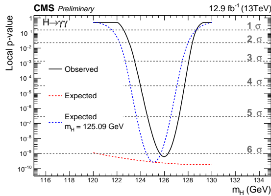
Figure 35: La signification observée (noir) est comparée à celle attendue dans l'intervalle 120-130 GeV, où on suppose que le boson de Higgs a une masse m_H = 125.09 GeV (bleu). La ligne rouge indique la signification statistique attendue pour chaque hypothèse de masse dans l'intervalle 120 \text{ GeV} < m_H < 130 \text{ GeV} .
