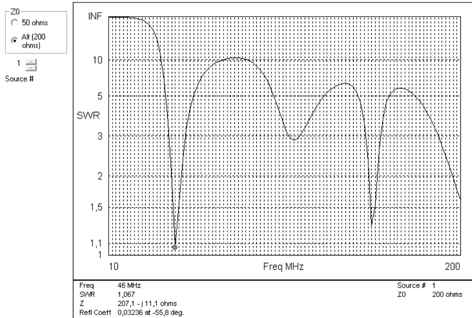
FIGURE 4.25 – Simulation EZNEC du SWR de l’antenne butterfly orientée E-W et positionnée au centre de la cuve, 1.5 m au dessus de l’eau, de fréquence de résonance 46 MHz et chargée sur une impédance de 200 \Omega [150].
