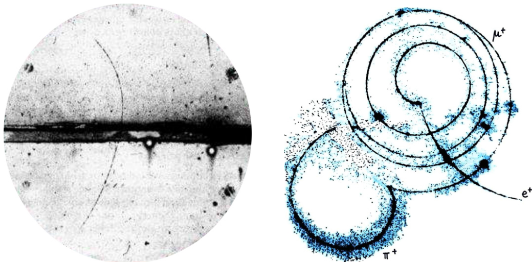
FIGURE 1.2 – Gauche : trace d'un positron traversant par le bas une chambre à brouillard (chambre de Wilson) plongée dans un fort champ magnétique. Droite : trace de la désintégration pion-muon-électron dans une chambre à brouillard [3].
