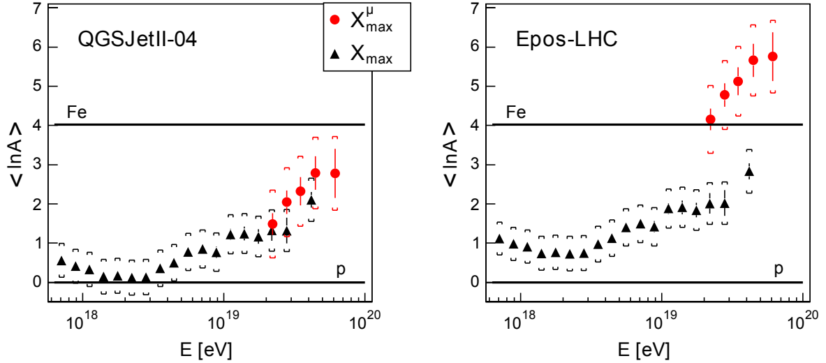
FIGURE 2.17 – Moyenne du logarithme du nombre de masse du primaire en fonction de son énergie, inférée à partir des valeurs expérimentales de X_{max} (noir) et X_{max}^{\mu} (rouge) associées au modèle QGSJetII-04 à gauche et au modèle Epos-LHC à droite [66].
