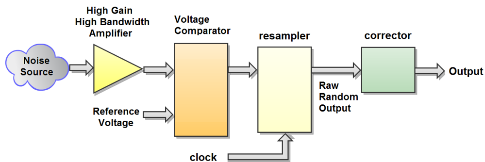
FIGURE 2.12 – TRNG basé sur l'amplification directe du bruit.
