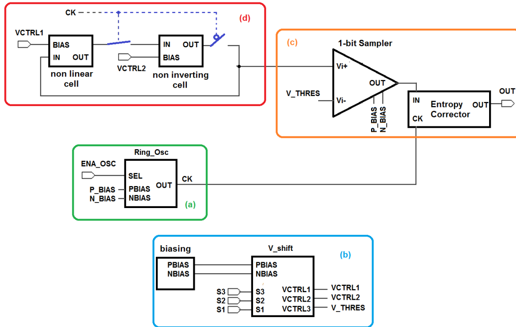
FIGURE 5.1 – Diagramme en blocs du TRNG proposé
