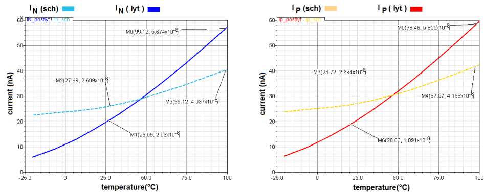
FIGURE 4.28 – Variation du courant avec la température (simulations pré-post Layout).
