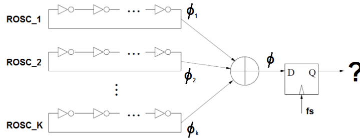
FIGURE 2.19 – schéma de fonctionnement d'un ROSCPUF.
