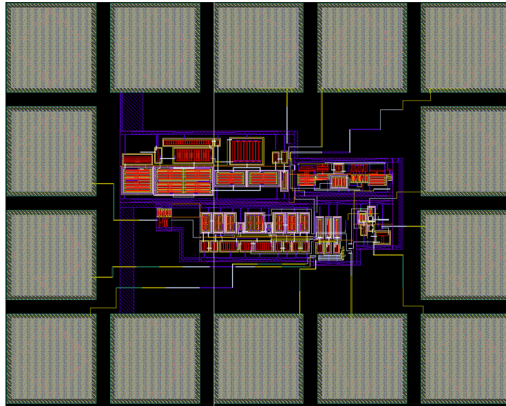
FIGURE 5.15 – Layout du sous-système.
