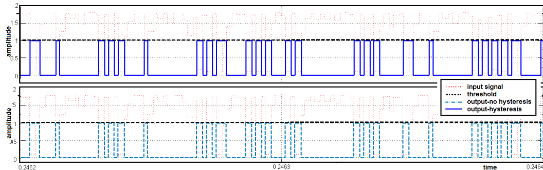
FIGURE 5.5 – Effet de l’hystérésis sur le modèle du comparateur.
