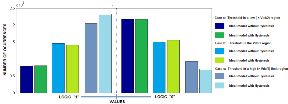
FIGURE 5.6 – L'effet de l'hystérésis dans trois placements du seuil.
