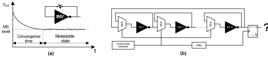
FIGURE 2.20 – PUF à métaoscillateur : (a) méta-inverseur (b) schéma équivalent du système .
