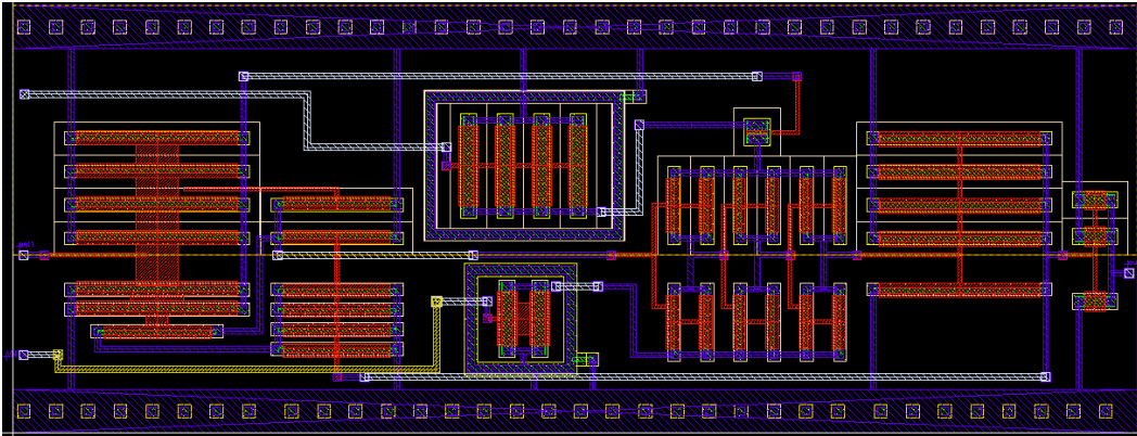
FIGURE 4.11 – Layout correspondant au bloc oscillateur.
