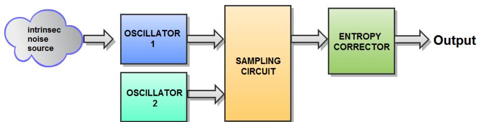
FIGURE 2.14 – TRNG basé sur l'échantillonnage d'horloges.
