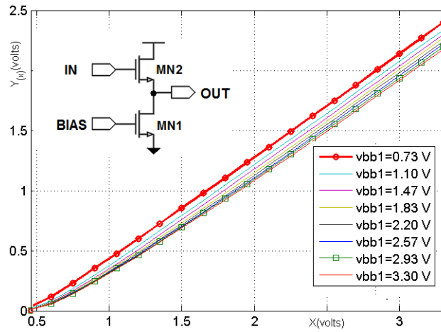
FIGURE 4.15 – Simulation paramétrique de l'étage non Inverseur.
