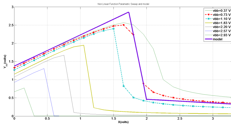
FIGURE 4.18 – Modèle simplifié de la fonction de transfert.
