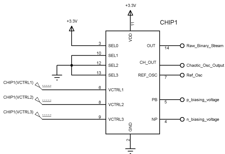
FIGURE 5.18 – Configuration de test sur le chiptest
