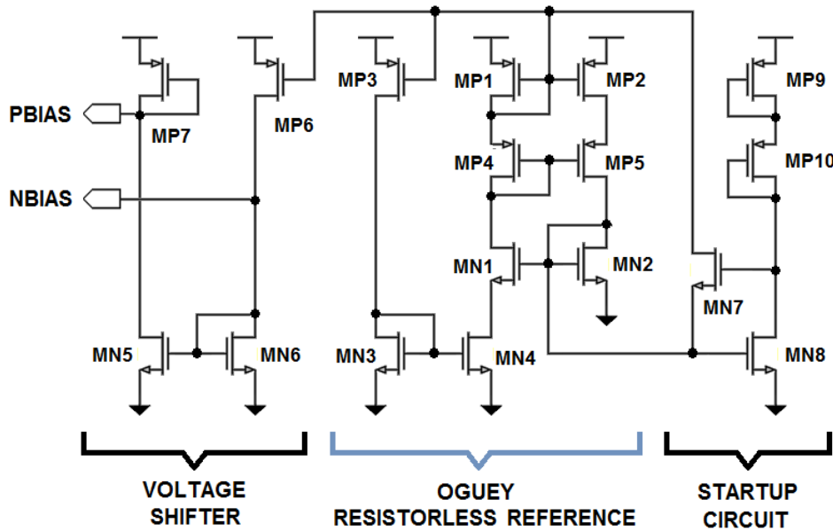
FIGURE 4.25 – Circuit de polarisation-démarrage
