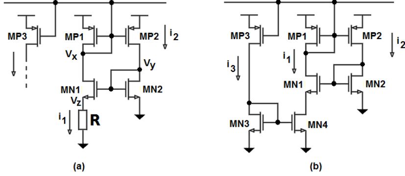
FIGURE 4.24 – (a) référence "classique" (b) référence Oguey.
