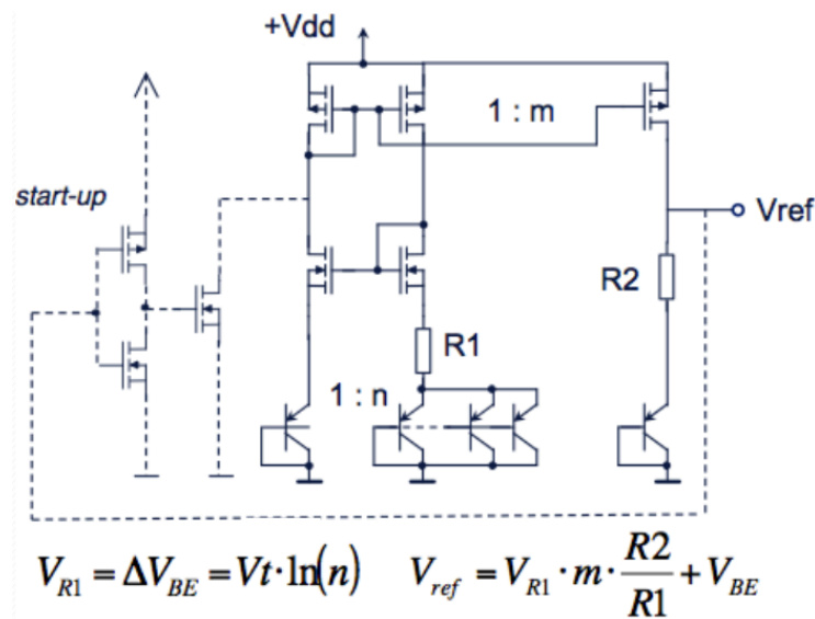
FIGURE 4.23 – Exemple classique de reference bandgap BiCMOS.
