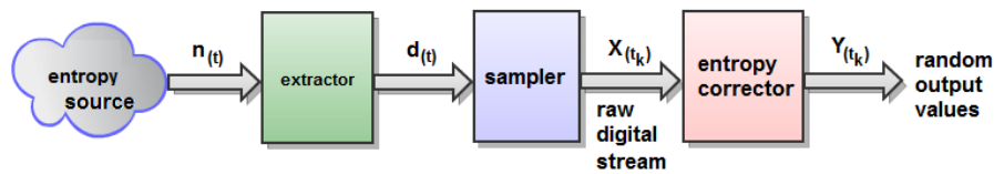
FIGURE 2.11 – Diagramme de blocs d'un TRNG.
