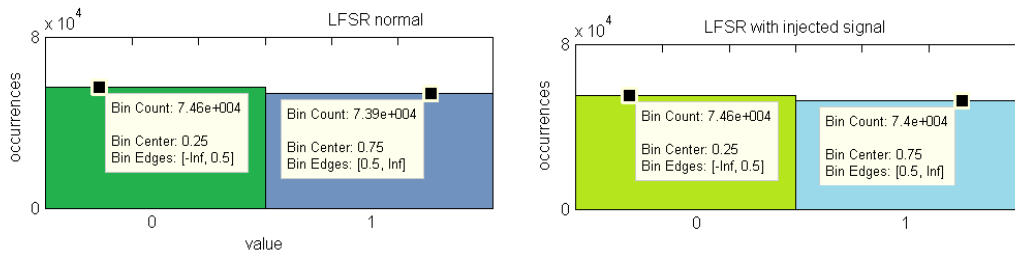
FIGURE 5.14 – Distribution binaire (a)LFSR solo (b) avec injection du signal biaisé.
