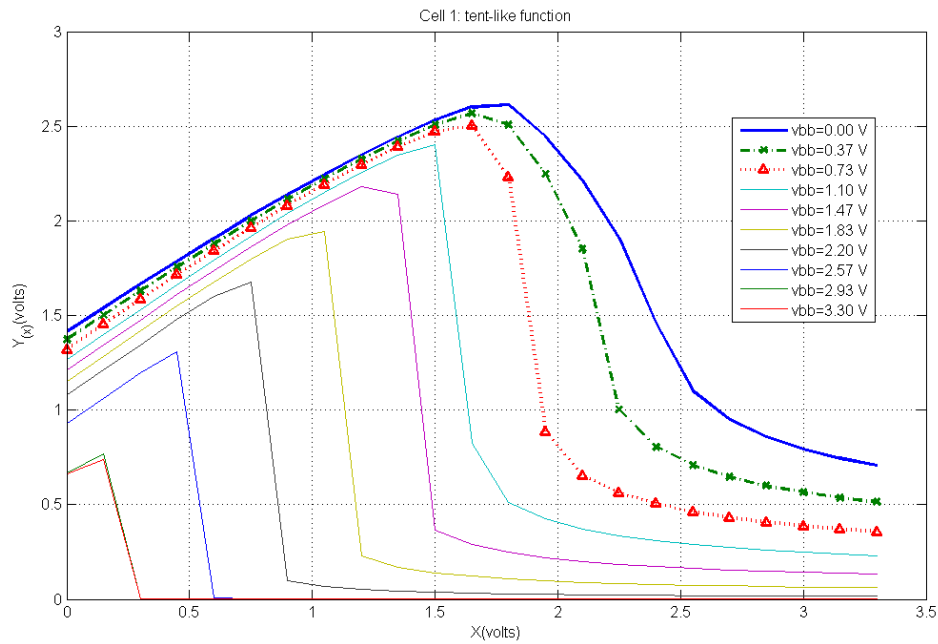
FIGURE 4.17 – Simulation paramétrique du circuit non linéaire type "tente"
