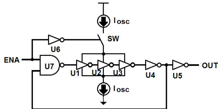
FIGURE 4.7 – Diagramme simplifié du générateur d'horloge.
