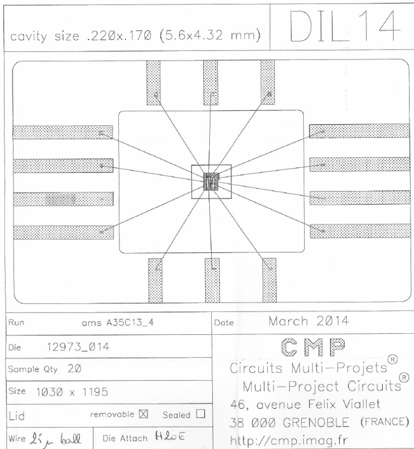
FIGURE 5.17 – Distribution des broches sur le chiptest
