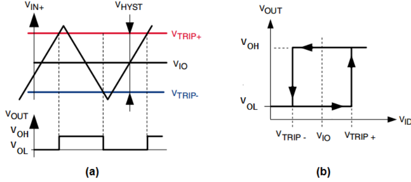
FIGURE 5.2 – Comparateur (a) Modèle (b) Caractéristique entrée V_{ID} -sortie V_{OUT}
