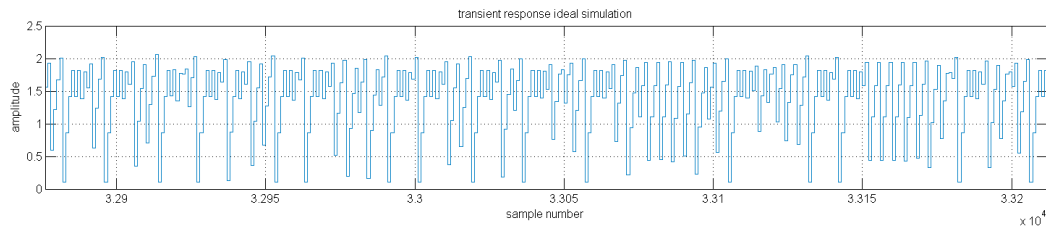
FIGURE 4.32 – Simulation transitoire du modèle idéal sous Matlab.
