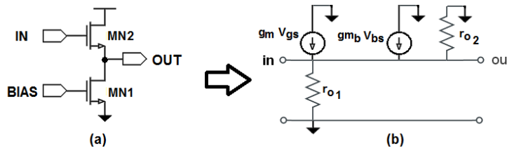
FIGURE 4.13 – NSF (a) schématique (b) schéma petit signal.
