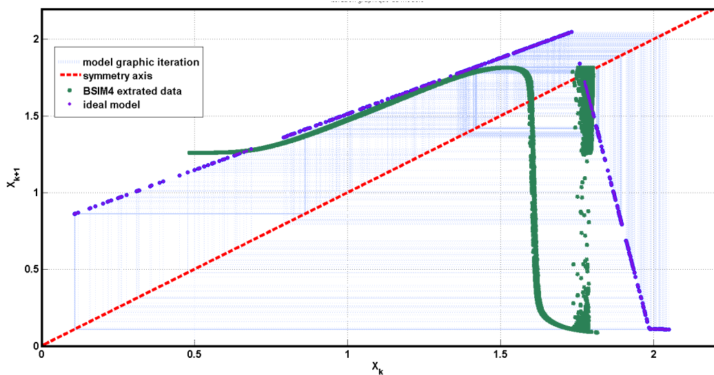
FIGURE 4.35 – comparaison des espaces générés par le modèle idéal et le modèle sous simulation.
