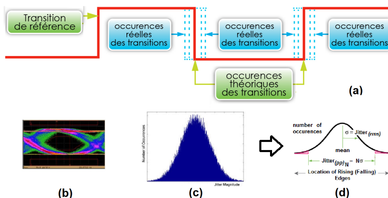
FIGURE 2.15 – (a)Le jitter (b) diagramme d'oeil (c) histogramme des variations de la période (d) analyse du jitter à partir de l'historgramme.
