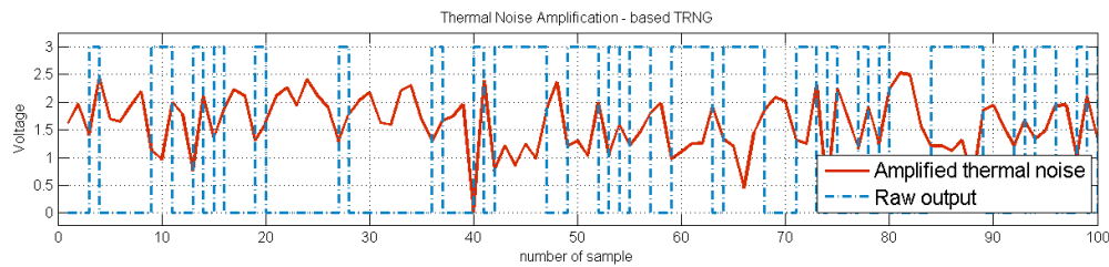
FIGURE 2.13 – Obtention de valeurs aléatoires à partir du seuillage de la sortie amplifié du bruit.
