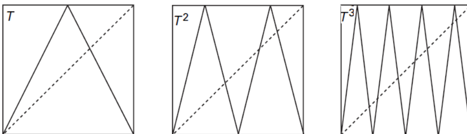
FIGURE 3.12 – Analyse des itérations de la fonction tente.
