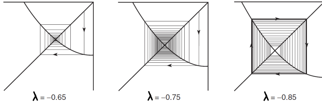
FIGURE 3.6 – Exemple de dédoublement de la période.
