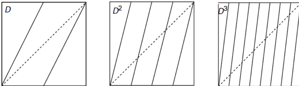
FIGURE 3.11 – Analyse des itérations de la fonction de doublement.
