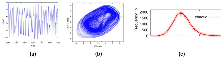
FIGURE 2.22 – Exemple d'un système chaotique : (a) sortie transitoire, (b) trajectoire chaotique, (c) histogramme du signal de sortie.
