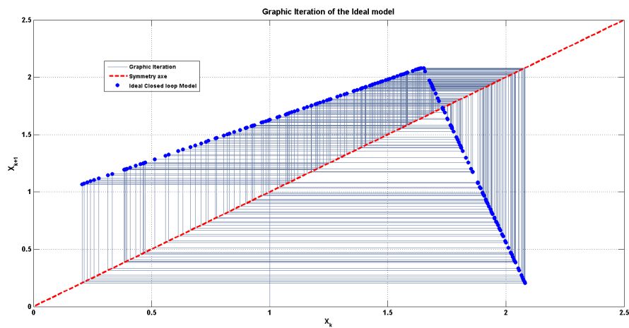
FIGURE 4.20 – Itération graphique du système idéal en boucle fermée.
