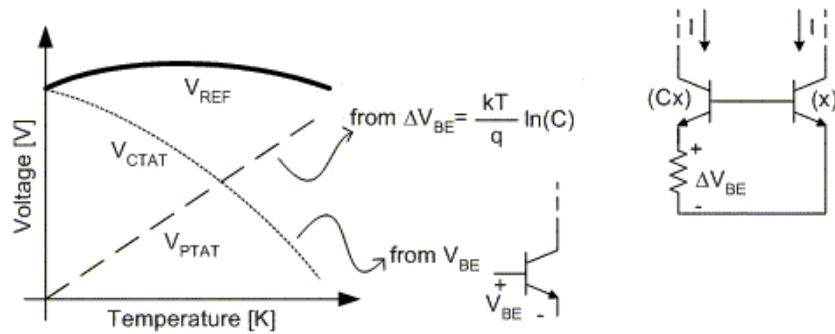
FIGURE 4.22 – Effet CTAT et PTAT et leur synthèse dans un système bandgap.
