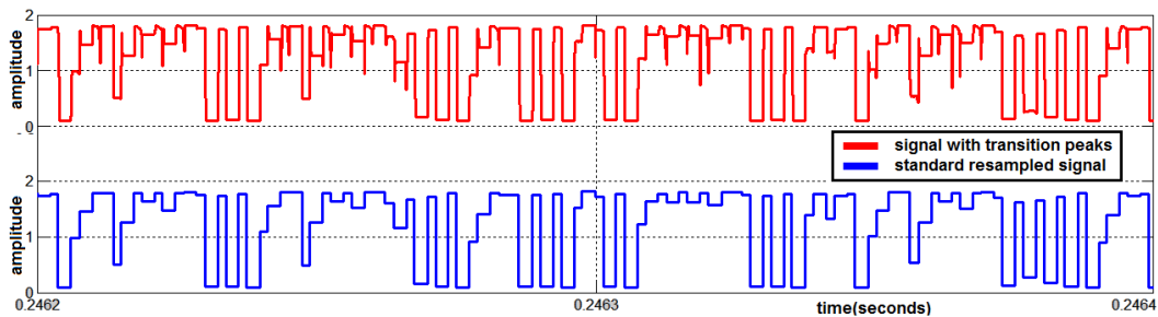
FIGURE 5.3 – Signal d'entrée du comparateur (en considérant ou pas les transitions de commutation).
