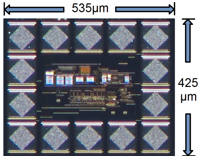
FIGURE 5.16 – Photographie du test chip réalisé.
