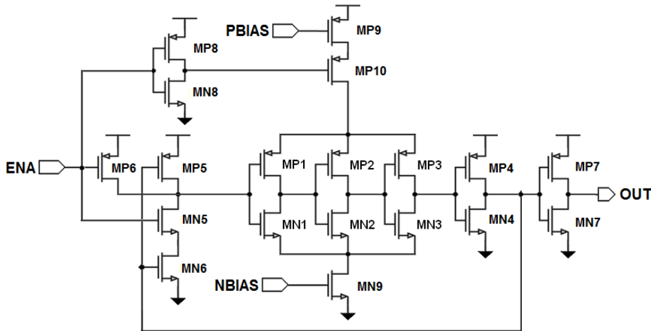
FIGURE 4.10 – Schématique du générateur d'horloge.
