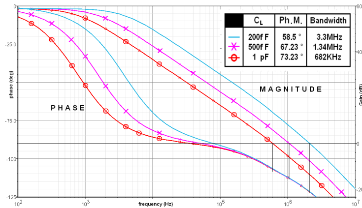
FIGURE 5.9 – Réponse en fréquence de l'OTA.
