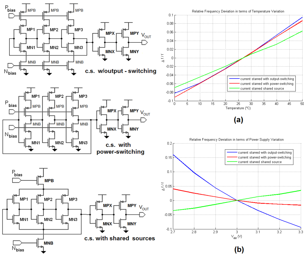
FIGURE 4.9 – Variantes de la topologie current starved et déviation relative de fréquences en fonction de : (a) la température (b) la tension d'alimentation.
