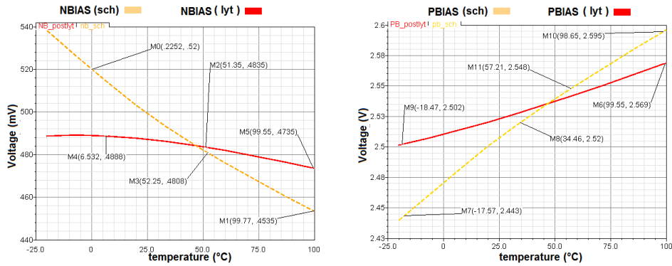
FIGURE 4.29 – Variation des tensions versus température (pré-post Layout).
