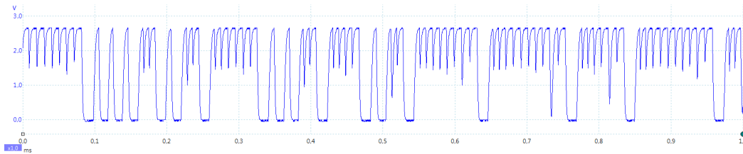
FIGURE 5.22 – détail de la sortie binaire sur le testchip.
