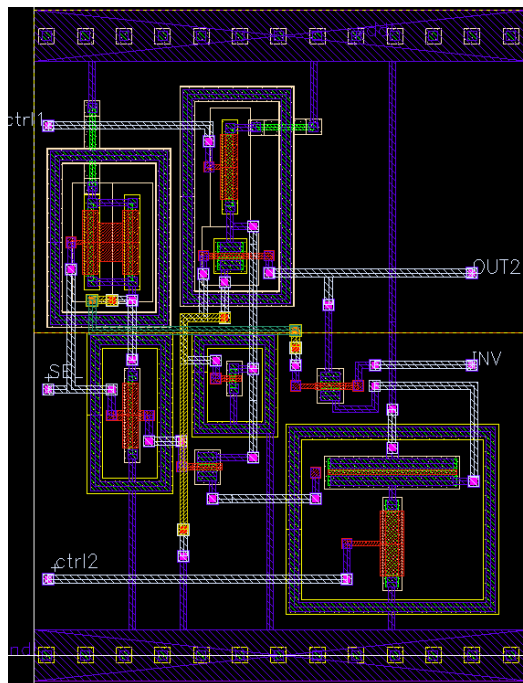
FIGURE 4.21 – Layout correspondant à l'oscillateur chaotique, incluant les interrupteurs, le suiveur et le bloc non linéaire.
