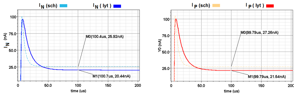
FIGURE 4.27 – Démarrage du circuit (simulations transitoires pre -post Layout).
