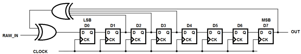
FIGURE 5.12 – Correcteur du type LFSR avec taps externes.
