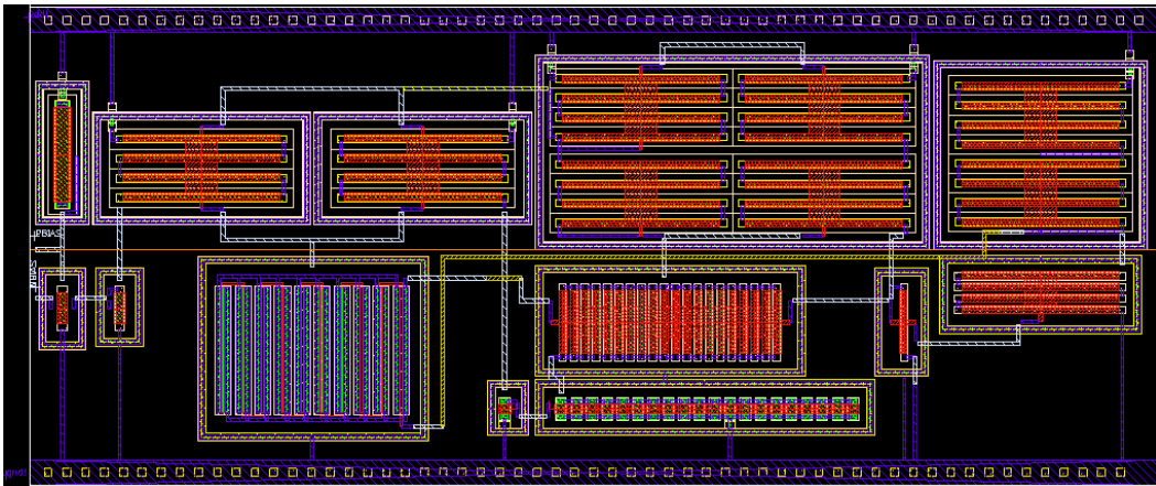
FIGURE 4.26 – Layout correspondant au circuit de polarisation-démarrage.
