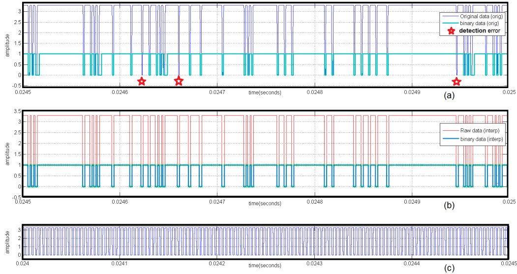
FIGURE 5.20 – Erreur de détection de données et correction par interpolation.
