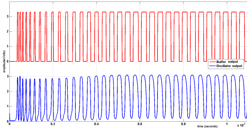
FIGURE 4.12 – Formes d’ondes générées par l’oscillateur.
