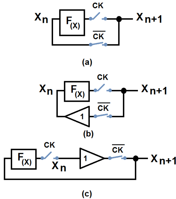
FIGURE 4.1 – Générateur chaotique en temps discret : (a) Schéma général (b) Équivalent avec étage non inverseur (c) Équivalent modifié.
