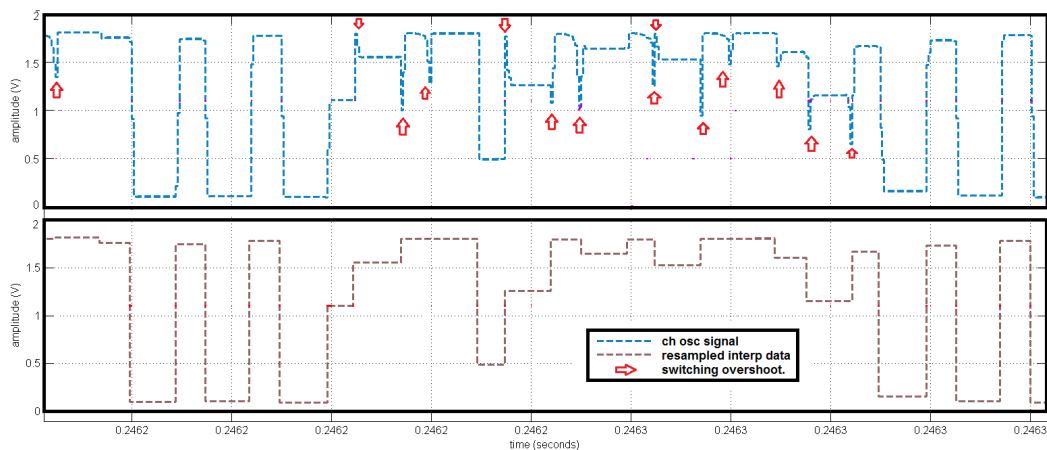
FIGURE 5.19 – Discrimination des surtensions de commutation lors de l'interpolation et re-échantillonnage du signal acquis.
