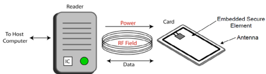
FIGURE 2.5 – Communication entre lecteur et carte RFID.
