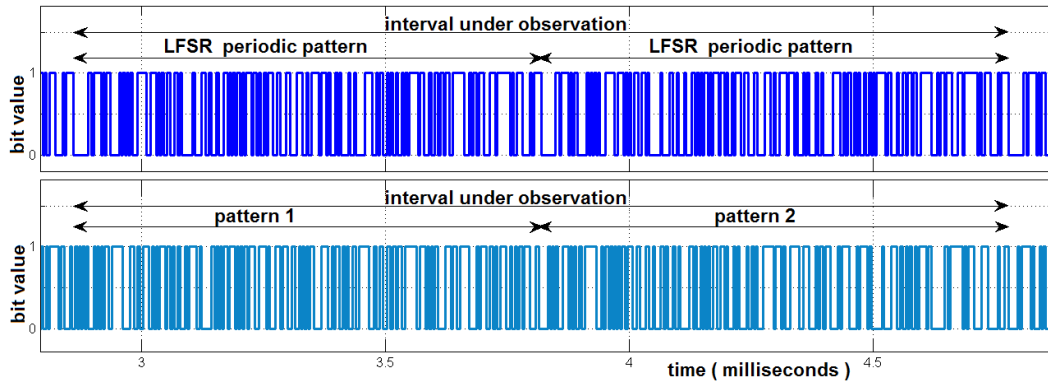
FIGURE 5.13 – LFSR (a)independant-PRNG (b)avec injection du signal biaisé.
