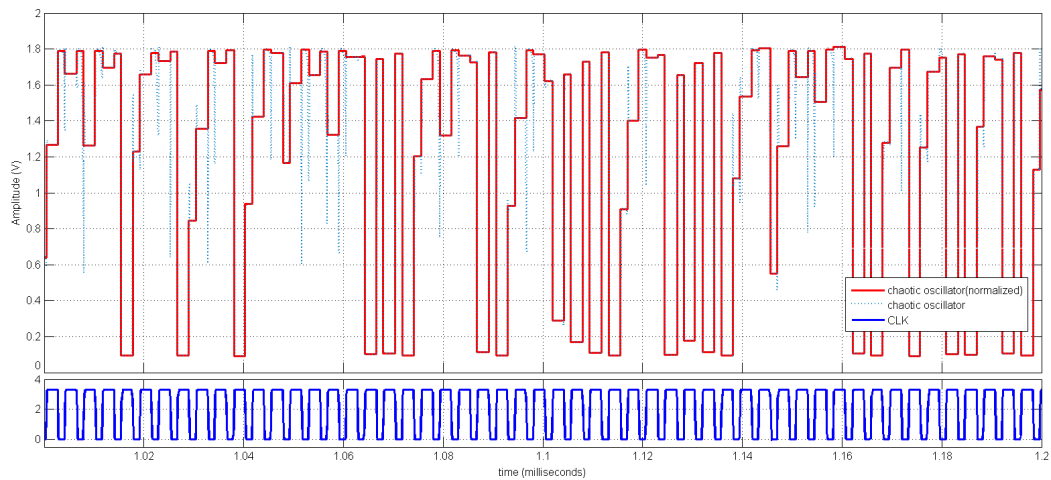
FIGURE 4.34 – Détail de la réponse transitoire indiquant les effets de commutation.
