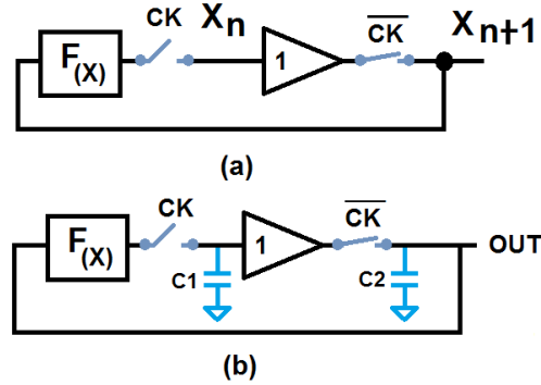
FIGURE 4.2 – (a) Modèle de l'oscillateur chaotique (b) avec représentation des éléments de mémoire capacitif.
