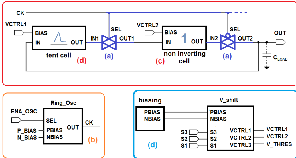
FIGURE 4.3 – Représentation en blocs de l'oscillateur chaotique.
