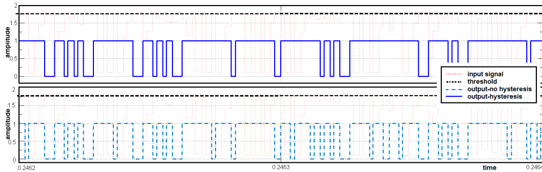
FIGURE 5.4 – Effet de l’hystérésis sur le modèle du comparateur ( V_{THRES} = 1,75V ).
