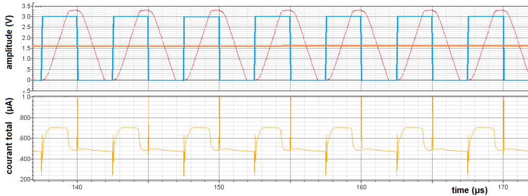
FIGURE 5.10 – Réponse transitoire du comparateur.
