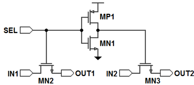
FIGURE 4.6 – Schématique des interrupteurs complémentaires.
