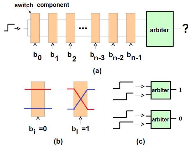
FIGURE 2.18 – APUF (a) schéma général ,(b) chemins de propagation,(c) opération de l'arbitre.
