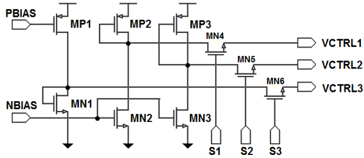
FIGURE 4.30 – Schématique du circuit de calibration.
