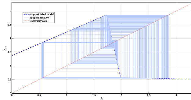
FIGURE 4.19 – Modèle linéarisé du comportement de la fonction discontinue avec itération graphique.
