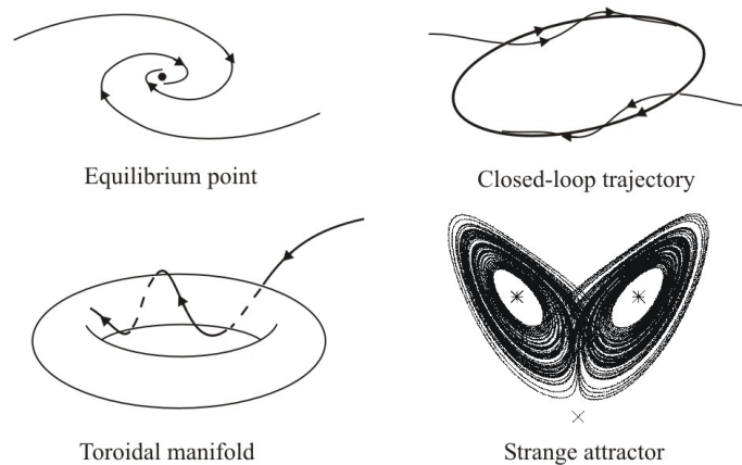
FIGURE 3.3 – Les différents types d'attracteurs
