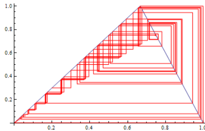
FIGURE 4.5 – Iteration graphique sur une fonction du type "tente".
