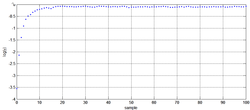
FIGURE 4.36 – Application de l'algorithme de Rosenstein.
