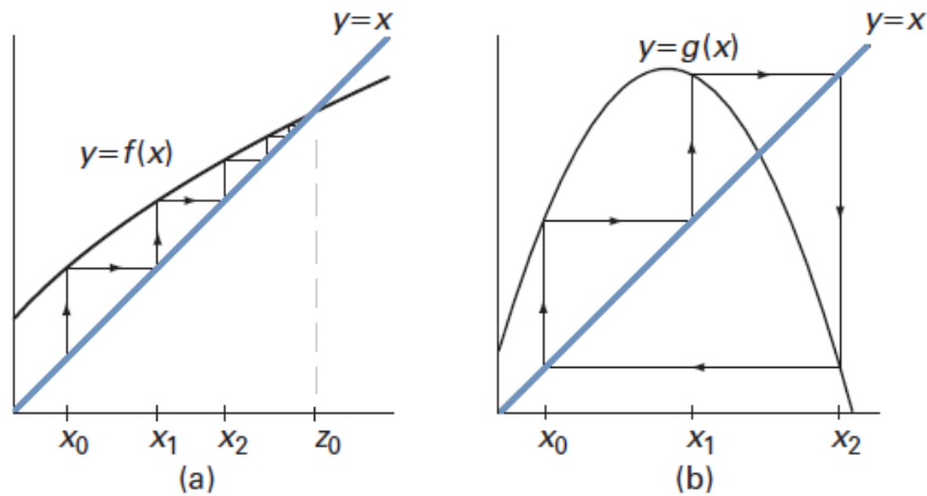
FIGURE 3.4 – Iteration graphique d'une trajectoire 1-D
