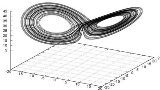
FIGURE 3.2 – L'attracteur de Lorenz ou "papillon".
