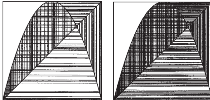
FIGURE 3.10 – Analyse des itérations de la fonction logistique.
