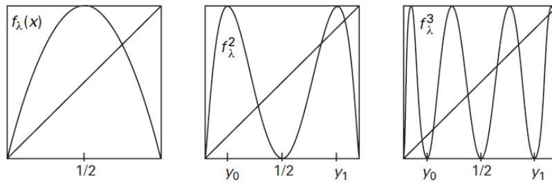
FIGURE 3.9 – Analyse des itérations de la fonction logistique.
