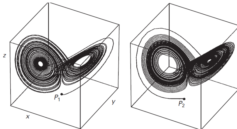
FIGURE 3.7 – Représentation 3D de l'attracteur de Lorenz avec deux conditions initiales différentes.
