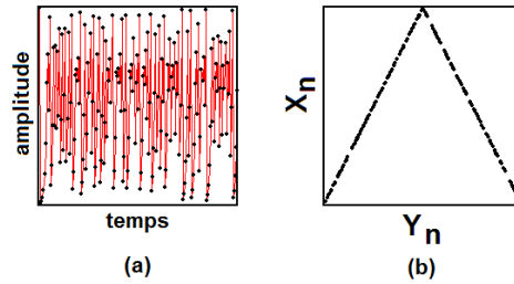
FIGURE 4.4 – "tent map" : (a) réponse transitoire (b) itération graphique.
