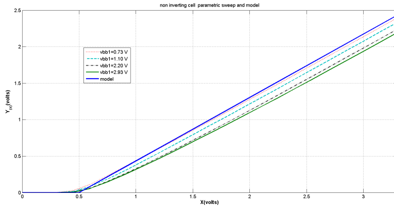
FIGURE 4.14 – Modèle utilisé versus simulation paramétrique de l'étage non inverseur.
