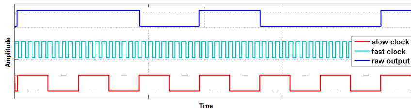
FIGURE 2.16 – Obtention de valeurs aléatoires à partir de l'échantillonnage d'horloges.
