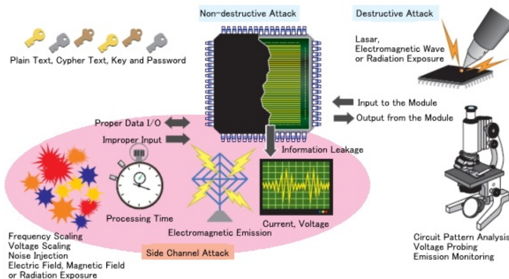
FIGURE 2.8 – Classification des techniques d'attaque sur les systèmes smartcard .
