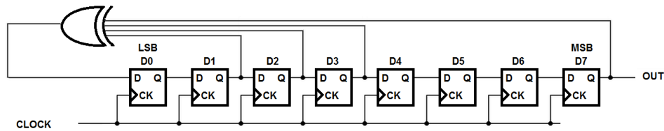
FIGURE 5.11 – Correcteur du type LFSR avec taps externes
