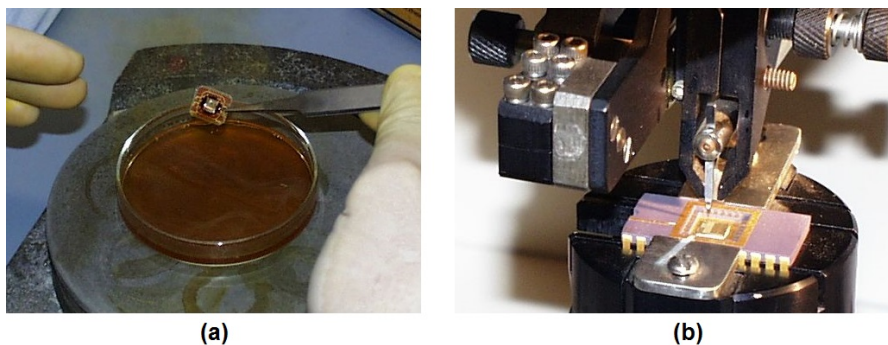
FIGURE 2.9 – Attaque invasif (a)corrosion du boitier. (b)insertion des sondes.
