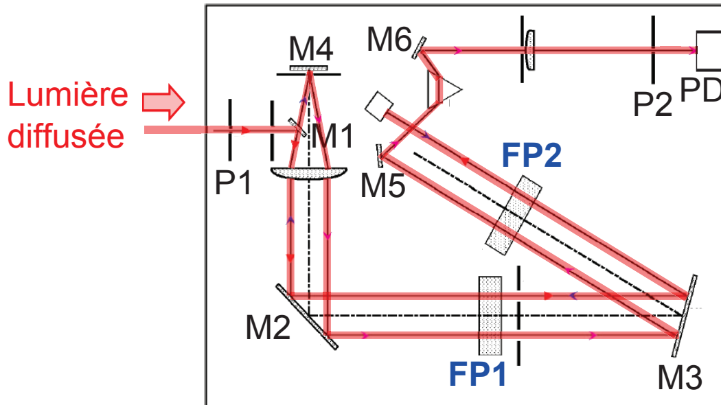
FIGURE B.3 – Schéma de principe du Tandem. Le trajet de la lumière est indiqué en rouge, les cavités FP en bleu et les éléments optiques principaux (miroir + trou d'entrée/sortie) en noir.
