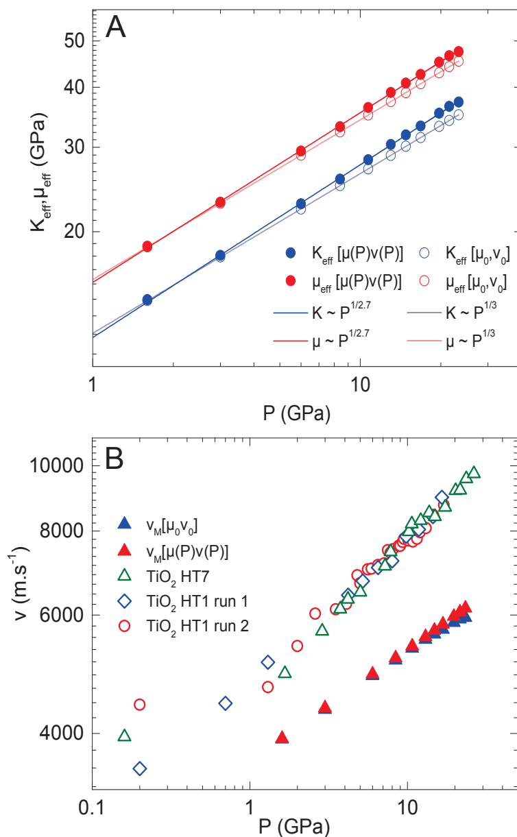
FIGURE 6.5 – A. Modules de compressibilité (bleu) et de cisaillement (rouge) effectifs de la poudre de \text{TiO}_2 HT1 calculés avec la théorie de Mindlin avec (cercles plein) et sans (cercles vides) la prise en compte de la dépendance en pression des constantes élastiques de \text{TiO}_2 . L'ajustement conduit à un coefficient \beta = 1/2.7 et \beta = 1/3 respectivement. B. Comparaison avec l'expérience des vitesses acoustiques calculées avec la théorie de Mindlin (équation 6.15) avec (triangles rouges) et sans (triangles bleus) la prise en compte de la dépendance en pression des constantes élastiques de \text{TiO}_2 .
