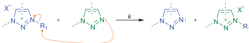
Schéma IV.13: Détails du mécanisme de l'hypothèse 1.
