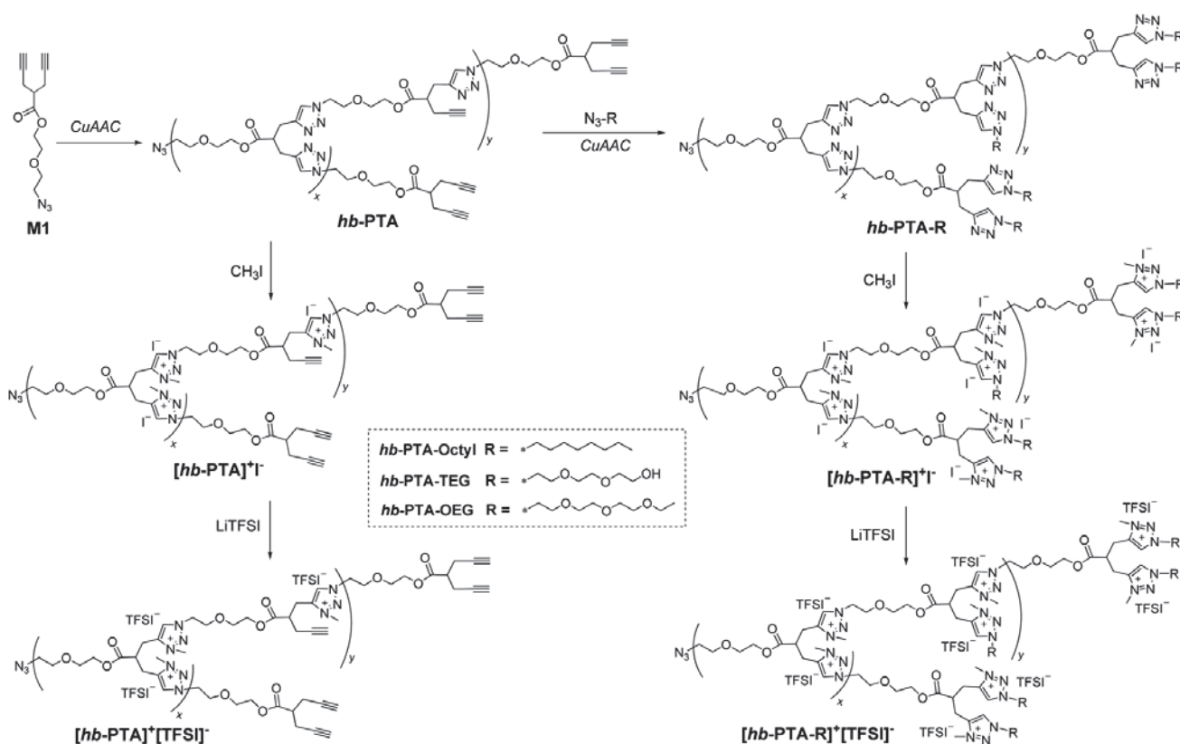
Schéma II.21: Synthèse de TPILs hyperbranchés. 83
