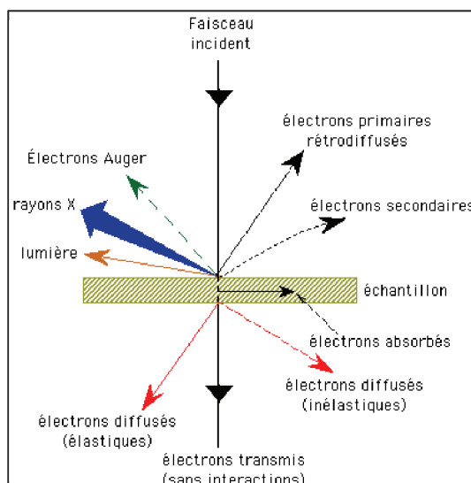
Figure 2.15: Ensemble des radiations pouvant être émises à partir de l'interaction entre le faisceau d'électrons et l'échantillon (source : http://www.mssmat.ecp.fr ).
