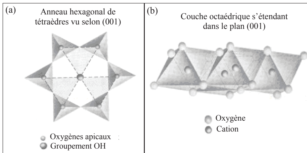
Figure 1.7: Structure de la serpentine. (a) représente les couches tétraédriques vue selon [001] et (b) représente les couches octaédriques constitutives des phyllosilicates dans le plan (001) (source : Klein et al., 1993).
