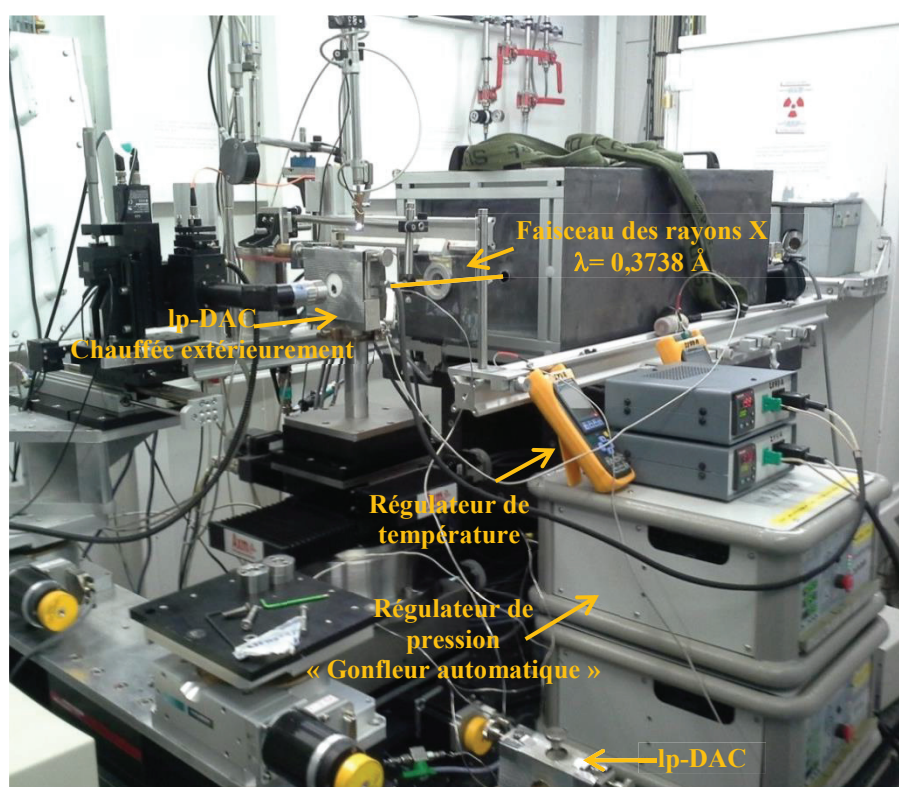
Figure 2.14: Montage expérimental de l'étude in situ de la réaction de serpentinisation sur la ligne ID-27 à l'ESRF (photo : Coll. avec H. Cardon, à l'ESRF, Grenoble).
