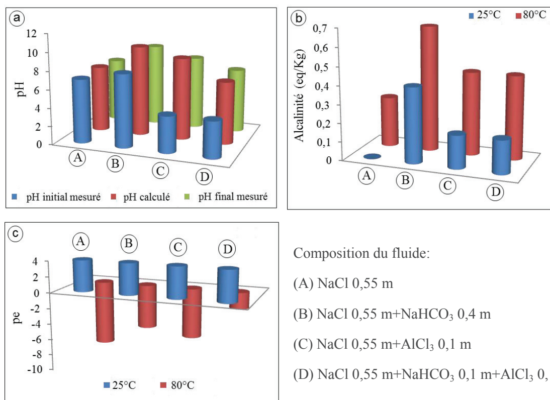
Figure 5.18: Valeurs du pH, de l'alcalinité et du pe obtenus avec la modélisation PHREEQC pour la réaction de serpentinisation avec différentes compositions de fluide à 80 °C et pression ambiante.
