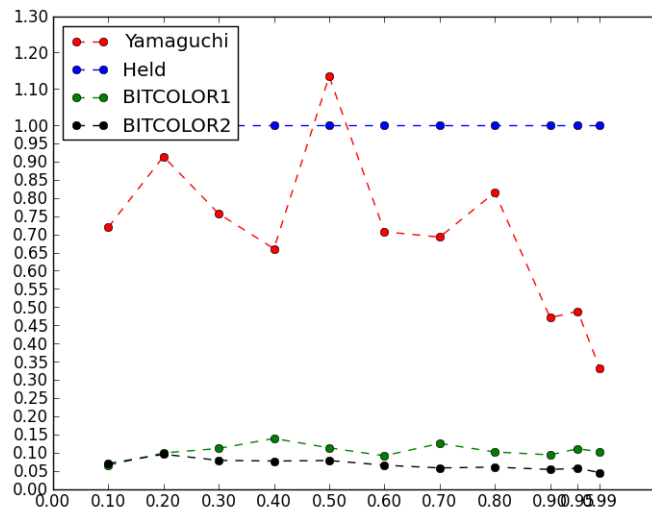
Figura 3.9: Razão entre a média dos tempos de execução de cada heurística e a média do tempo de execução de HCS, por densidade, para instâncias com 300 vértices
