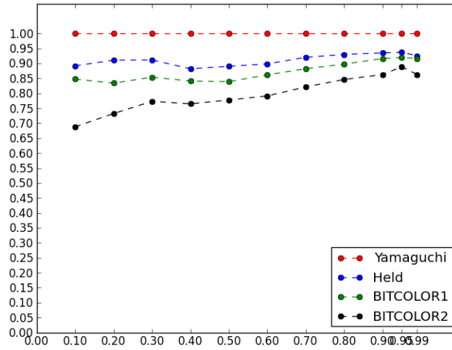
Figura 3.7: Razão entre a média dos limites superiores de cada heurística e a média do limite superior de YM, por densidade, para instâncias com 300 vértices
