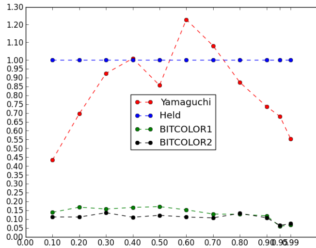
Figura 3.8: Razão entre a média dos tempos de execução de cada heurística e a média do tempo de execução de HCS, por densidade, para instâncias com 200 vértices
