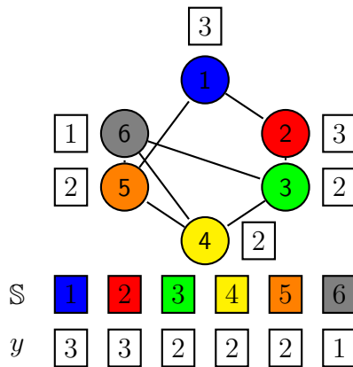
Figura 2.4: Coloração ponderada trivial: o peso da coloração ponderada trivial de G é 13. A clique máxima ponderada de G é 6.
