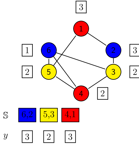
Figura 2.5: A coloração ponderada particionada de G mostrada na figura tem peso 8 e a clique máxima ponderada de G é 6.
