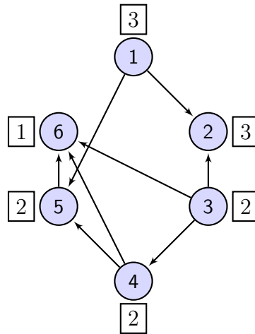
Figura 3.3: Grafo ponderado direcionado \vec{G}_\rho , onde \rho = (1, 3, 4, 2, 5, 6)
