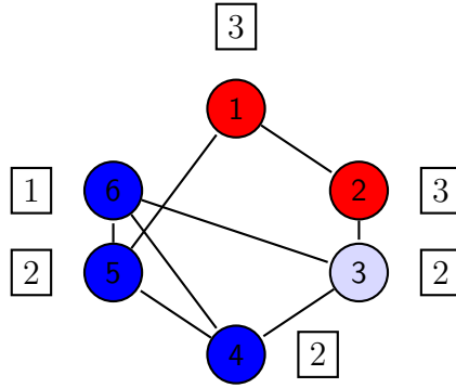
Figura 2.2: Relação entre o problema CLIQUE e CLIQUE PONDERADA: o conjunto de vértices \{4,5,6\} é uma clique máxima de G , mas não é a clique máxima de ponderada de G , que é definida por \{1,2\} .
