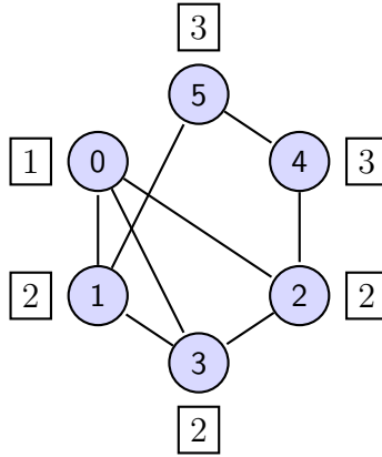
Figura 6.1: Grafo ponderado com os vértices ordenados seguindo a ordem do menor peso primeiro .
