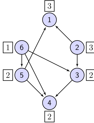
Figura 3.2: Grafo ponderado direcionado \vec{G}_\rho , onde \rho = (6, 2, 5, 3, 4, 1)
