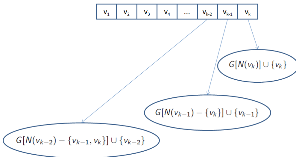
Figura 3.10: Esquema de ramificação de Balas-Yu
