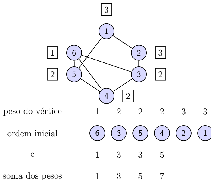
Figura 5.1: Limites superiores dados pela soma dos pesos dos vértices e pelos valores de c[i] para cada G_i , para i = 1, \dots, 4 .
