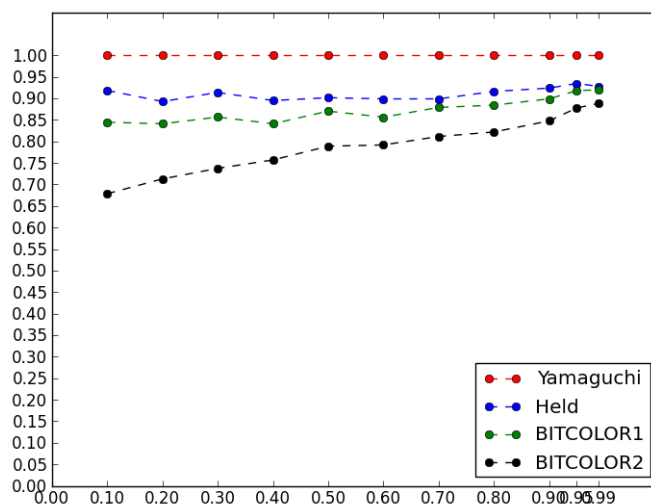
Figura 3.6: Razão entre a média dos limites superiores de cada heurística e a média do limite superior de YM, por densidade, para instâncias com 200 vértices
