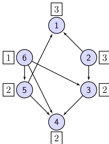
Figura 3.4: Grafo ponderado direcionado \vec{G}_\rho , onde \rho = (2, 6, 5, 1, 3, 4)
