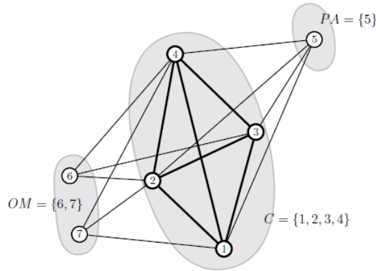
Figura 4.1: Relação entre uma clique C e os subconjuntos de vértices PA e OM . Fonte: [Wu, Hao e Glover 2012]
