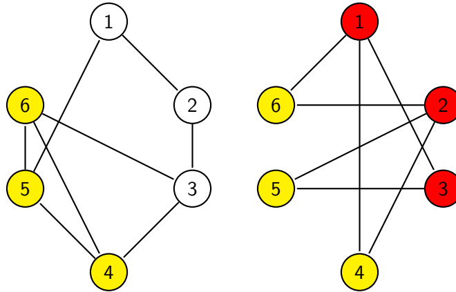
Figura 2.1: A relação entre a clique máxima, conjunto independente máximo e cobertura mínima de vértices. O grafo da direita, denotado por \overline{G} , é o complemento do grafo da esquerda denotado por G . O conjunto de vértices \{4,5,6\} define a clique máxima de G e o conjunto independente máximo de \overline{G} . O conjunto de vértices \{1,2,3\} representa a cobertura mínima de \overline{G} .
