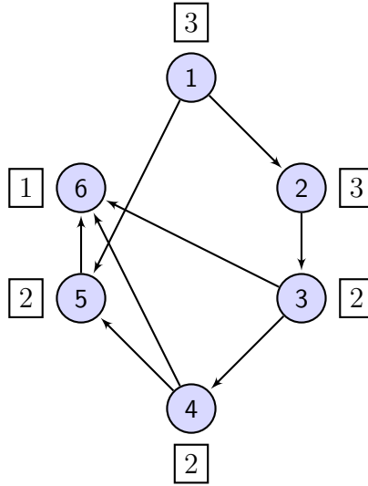
Figura 3.1: Grafo ponderado direcionado \vec{G}_\rho , onde \rho = (1, 2, 3, 4, 5, 6)
