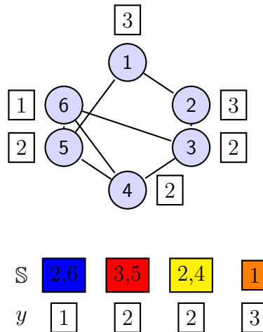
Figura 2.6: O peso da coloração ponderada inteira de G é 8. A clique máxima ponderada para G é 6.
