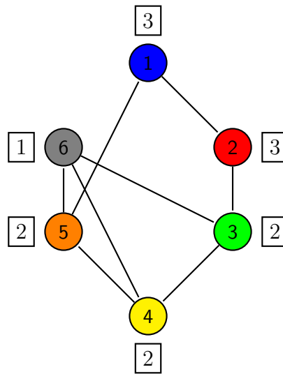
Figura 3.5: Grafo Ponderado
