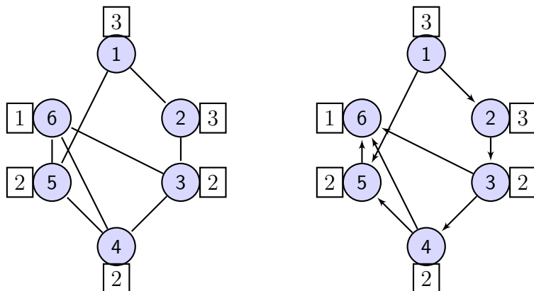
Figura 2.3: O grafo da esquerda é um grafo ponderado utilizado para obter o grafo direcionado acíclico induzido pela sequência (1,2,3,4,5,6) (grafo da direita).
