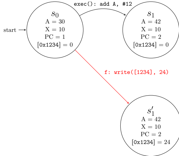
FIGURE 5.3. – Graphe d'exécution fauté
