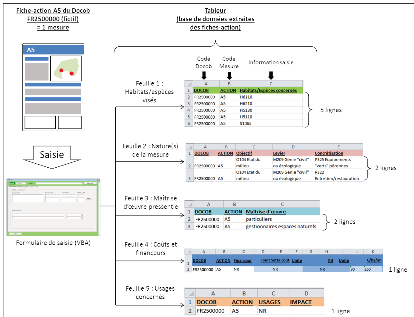
Figure 33 : Représentation schématique de la constitution d'une base de données (codage) à partir des fiches-actions des Docob
