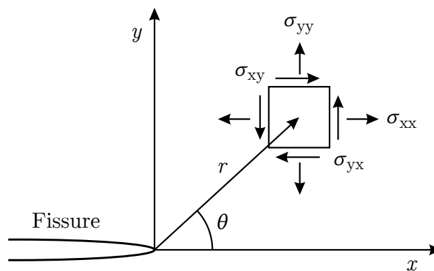
Figure 6.2 – Diagramme de contraintes sur un point à une distance r et angle \theta par rapport à la pointe de la fissure (Irwin, 1958 ; Hertzberg, 1996 ; Miyaura, 2012).
