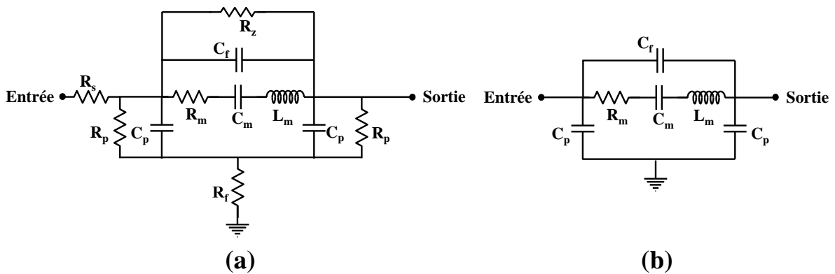
Figure 5-2 : (a) Schéma électrique équivalent tenant compte des pertes dans la couche de ZnO et dans la membrane suspendue de silicium et (b) modèle simplifié dans lequel toutes ces pertes ont été négligées pour faciliter la conception des filtres
