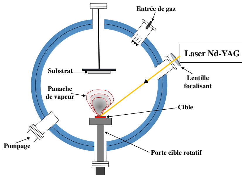
Figure 2-11 : Schéma représentant le principe d'un système de dépôt par PLD
