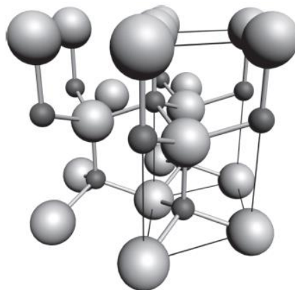
Figure 2-10 : La structure Wurtzite hexagonale de ZnO. Les atomes O sont représentés par de grandes sphères blanches tandis que les atomes de Zn sont les petites sphères grises foncées
