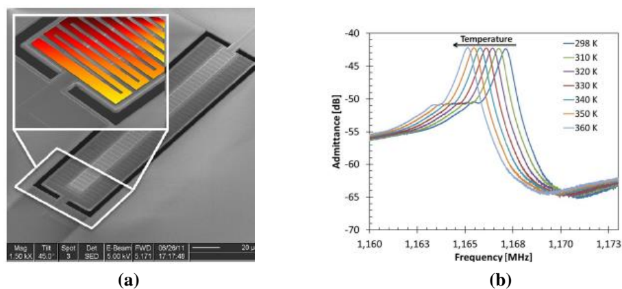
Figure 1-28 : (a) Images MEB du micro-résonateur AlN, l'électrode en rouge représente l'électrode à serpents de chauffage. (b) Mesure de l'admittance Y_{11} à différentes températures pour le résonateur 1,1 GHz [96]
