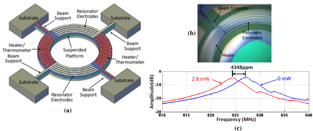
Figure 1-29 : (a) Un schéma du micro-résonateur AlN accordable intégrant un système de chauffage. (b) Image microscopique d'un coin du dispositif fabriqué. Les électrodes du micro-résonateur font 4µm de largeur. (c) La réponse fréquentielle mesurée du micro-résonateur avant et après chauffage (2,8 mW) [97]
