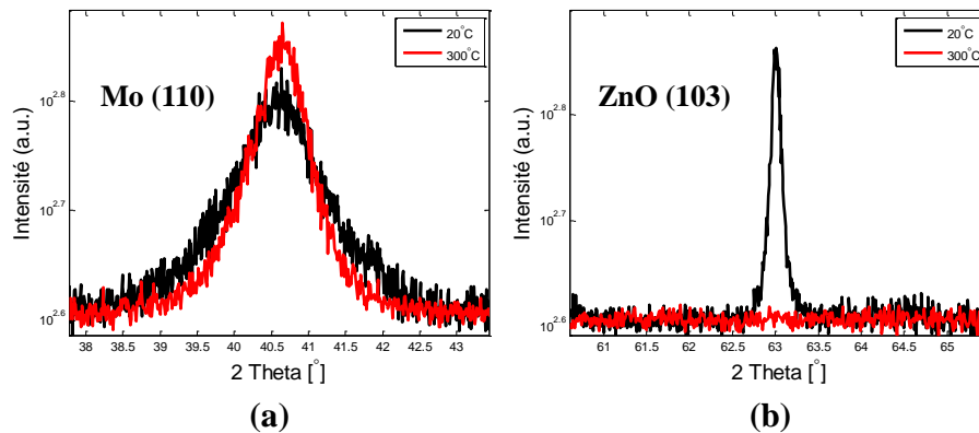
Figure 2-24 : (a) Amélioration de la qualité cristalline du Molybdène déposé à 300°C (pic de Mo (110) plus étroit) et (b) disparition de l'orientation secondaire du ZnO (103) quand il est déposé sur du molybdène obtenu à 300°C
