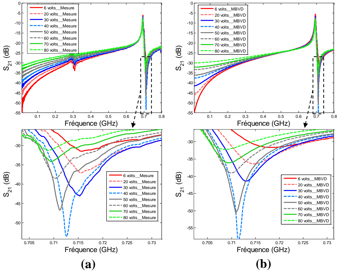
Figure 3-45 : Réponse en transmission S_{21} d'un micro-résonateur ( L= 140 \mu\text{m} & n=40 IDTs) avec une tension de polarisation balayée entre 6 et 80 V : (a) en mesure et (b) en simulation avec le modèle de MBVD et les valeurs du tableau 3-8
