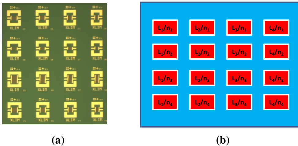
Figure 3-19 : (a) Photo MEB des circuits réalisés et (b) représentation de la position des circuits en fonction de la variation de la longueur ( L_n ) et du nombre ( n ) de peignes IDTs
