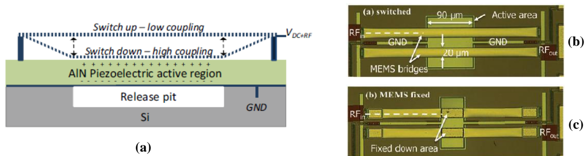
Figure 1-30 : (a) Vue schématique du dispositif de commutation piézo-électrique. Lorsque l'électrode de commutation supérieure est séparée de la région piézo-électrique, le couplage est faible et le résonateur est éteint. Lorsqu'une tension de polarisation est appliquée, l'électrode est amenée en contact par attraction électrostatique, et le résonateur fonctionne. (b) et (c) représentent des images du dispositif réalisé, (a) à l'état off et (b) à l'état ON [99]
