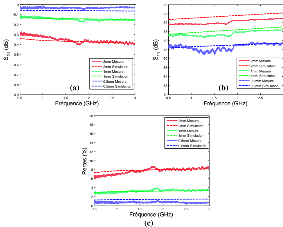
Figure 3-6 : (a) et (b) Paramètres [S], en mesures et en simulations, de lignes coplanaires réalisées sur un substrat désoxydé de Si HR et (c) représente les pertes calculées à partir de ces mesures
