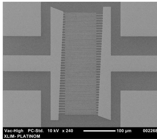
Figure 3-3 : Image MEB d'une capacité en forme de peignes IDTs possédants 80 peignes de longueur de 100 \mu\text{m}
