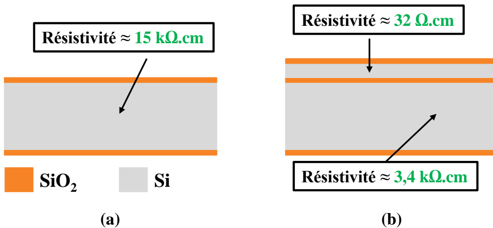
Figure 3-2 : Valeurs de résistivité du substrat en silicium sur lequel les micro-résonateurs sont réalisés dans le cas d'un wafer Silicium HR (a) et celui d'un wafer type SOI (b)
