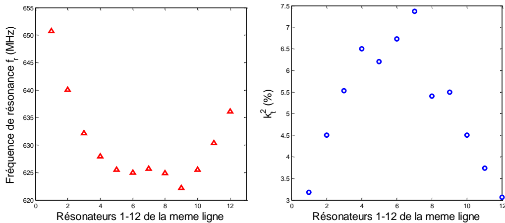
Figure 2-33 : Dispersion de la fréquence centrale de résonance f_r et du coefficient de couplage électromécanique k_t^2 selon la position des résonateurs qui sont distribués sur une même ligne sur le substrat d'accueil
