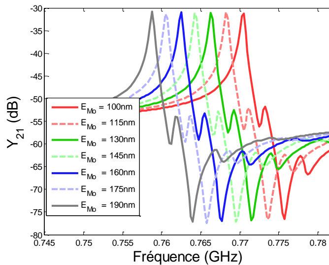
Figure 5-6 : Réponse Y_{21} de plusieurs micro-résonateurs intégrant une couche de ZnO de 200 nm et différentes épaisseurs de l'électrode inférieure en molybdène
