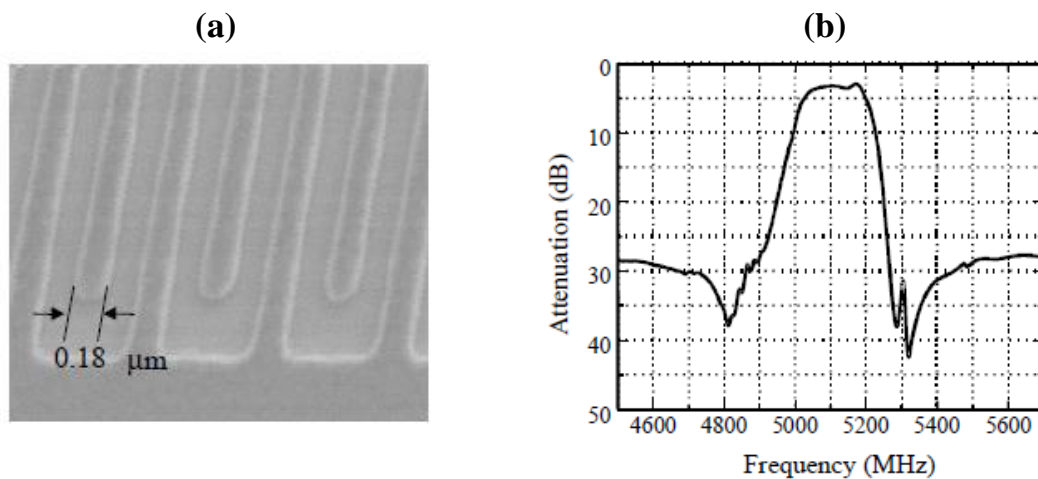
Figure 1-12 : Exemple de filtre SAW fonctionnant au-delà de 5GHz [64] : (a) Résolution lithographique de 0.18\mu\text{m} des électrodes inter-digitées (SAW) et (b) la réponse en transmission du dispositif
