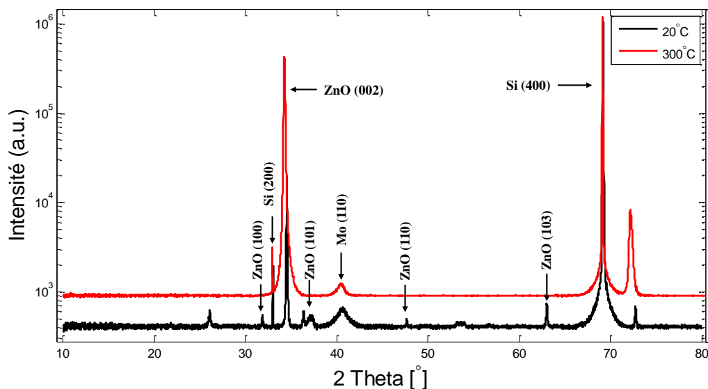
Figure 2-23 : Diagrammes de diffraction des rayons X de couches minces de ZnO déposées sur du molybdène obtenues à température ambiante et à 300°C
