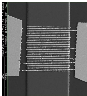
Figure 4-23 : Image par microscopie électronique à balayage MEB qui montre le décolllement des électrodes IDTs à l'extérieur de la région structurée Mo+AlN
