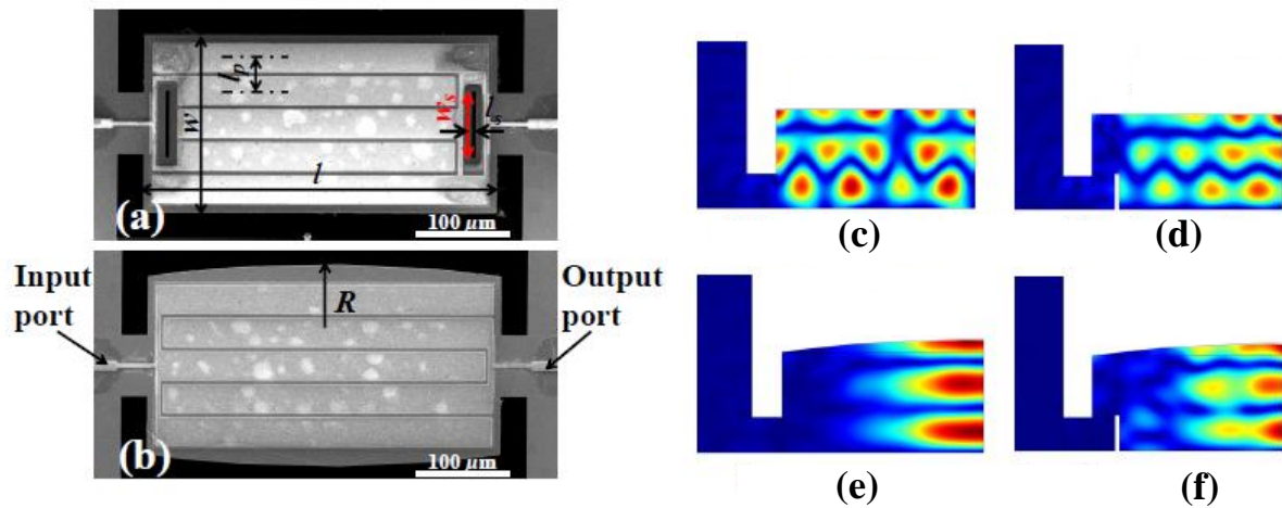
Figure 2-1 : Image MEB de micro-résonateurs possédant une membrane suspendue en Si (a) avec des fentes et (b) en forme biconvexe. Les résultats des simulations FEM montrant la dispersion des ondes acoustiques dans la membrane de Silicium d'un (c) dispositif normal, (d) prévu avec des fentes usinés dans l'épaisseur de la membrane, (e) de forme biconvexe et (f) biconvexe avec fente [4]
