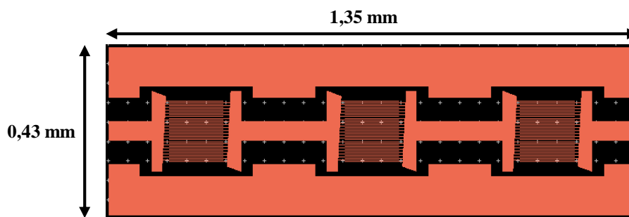
Figure 5-4 : Dessin d'un filtre trois pôles conçu à partir d'un micro-résonateur possédant 40 électrodes IDTs de longueurs de 100 \mu m (vue de dessus)
