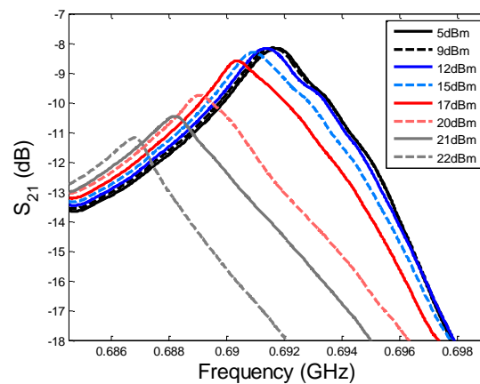
Figure 3-33 : Réponse en transmission S_{21} d'un micro-résonateur possédant 40 IDTs de longueur 100 \mu m pour différents niveaux de puissance d'entrée
