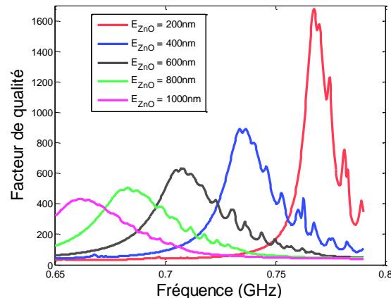
Figure 3-17 : Facteurs de qualité des micro-résonateurs intégrant des couches de ZnO avec différentes épaisseurs obtenus en simulation FEM
