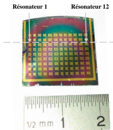
Figure 2-31 : Image du substrat d'accueil avec les résonateurs réalisés et mesurés. La zone active occupe 1.9cm×1.5cm et la couche de ZnO réparti sur toute cette zone possède une variation de l'épaisseur (vu la formation de plusieurs anneaux de couleurs différentes)
