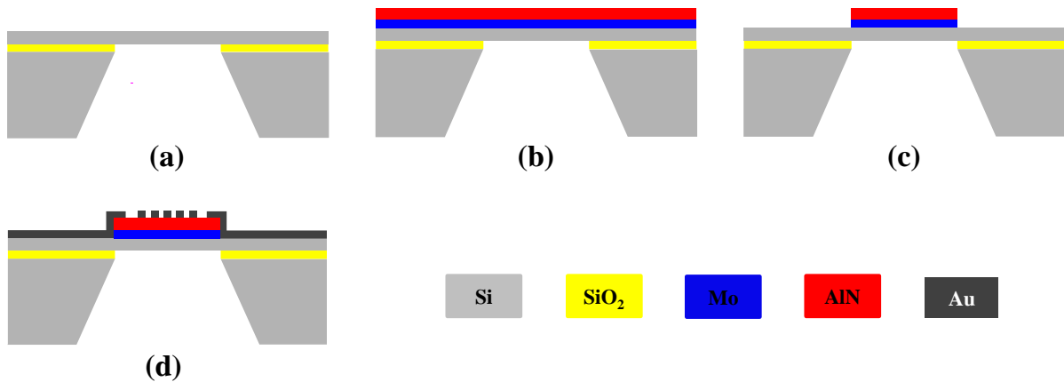
Figure 4-21 : Vue schématique des différentes étapes de réalisation des micro-résonateurs suivant le nouveau procédé. (a) Libération de la membrane de silicium, (b) dépôt du molybdène et de l'AlN sans remise à l'air entre les deux, (c) gravure de l'AlN et du molybdène en utilisant le même masque (celui de l'électrode inférieure) et (d) réalisation des électrodes supérieures IDTs en lift-off
