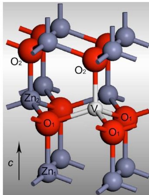
Figure 5-8 : Structure d'un ZnO dopé au vanadium
