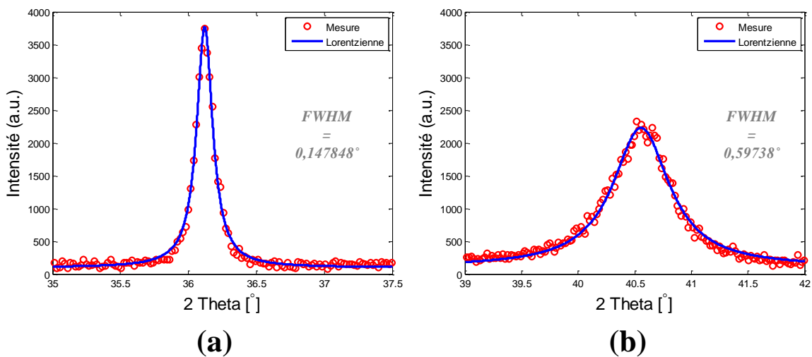
Figure 4-6 : Simulation par une fonction Lorentzienne des pics : (a) de l'AlN (002) et (b) du Mo (110), dans le cas d'un molybdène déposé à 300°C suivi d'un AlN déposé à température ambiante
