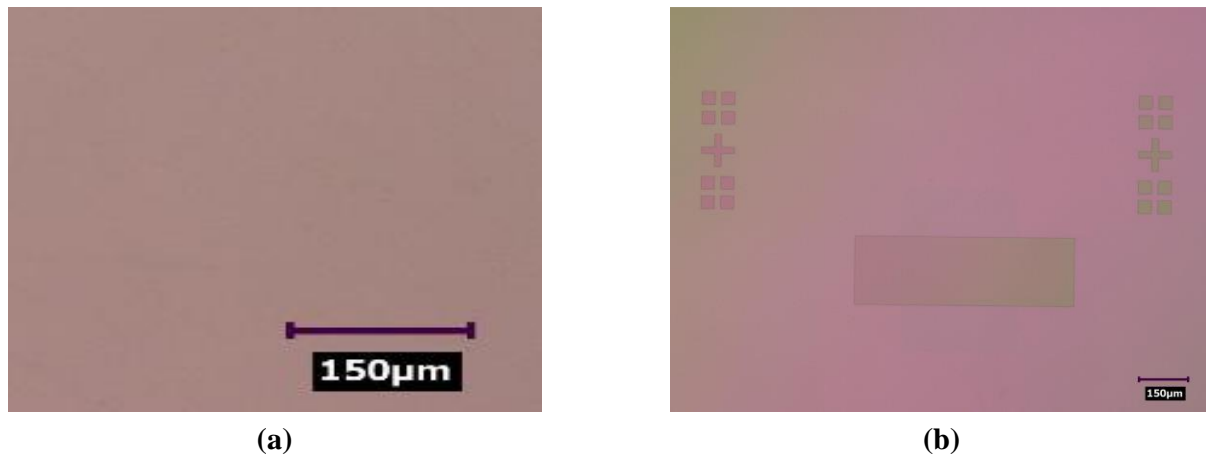
Figure 2-15 : Disparition totale des microfissures dans la couche de ZnO suite à l'optimisation du procédé de refroidissement à température ambiante après dépôt. (a) Un substrat en silicium et (b) un substrat SOI avec des membranes de silicium suspendues en très bon état
