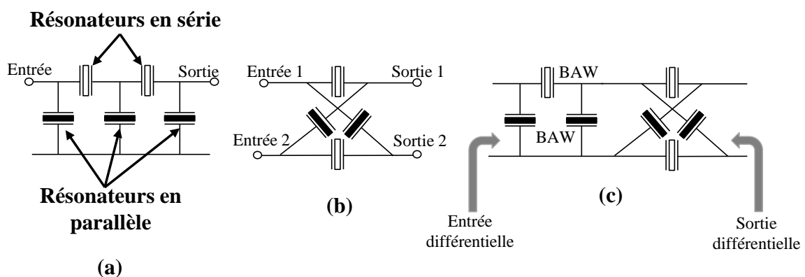
Figure 1-26 : Architecture de filtres à résonateurs BAW en : (a) échelle, (b) treillis et (c) échelle-treillis
