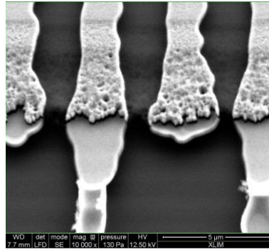
Figure 4-24 : Image par microscopie électronique à balayage MEB prise au niveau du bord de la région du Mo+AlN et qui montre la discontinuité structurale des électrodes IDT
