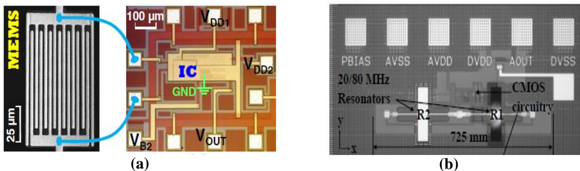
Figure 1-25 : (a) Image d'un micro-résonateur lié (par bonding) à un circuit intégré CMOS pour former un oscillateur fonctionnant à 1,5\text{GHz} [87]. (b) Image d'un oscillateur conçu à base d'un micro-résonateur intégré avec les composants CMOS. La zone active de l'oscillateur est égale à 0,23\text{mm}^2 [88]
