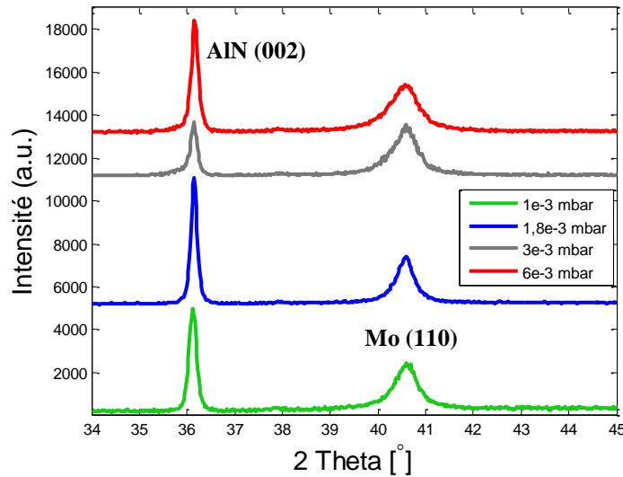
Figure 4-11 : Diagrammes de diffraction des rayons X de couches minces d'AlN déposées sur du molybdène. La pression globale des dépôts a été variée entre 6.10^{-3} mbar et 1.10^{-3} mbar
