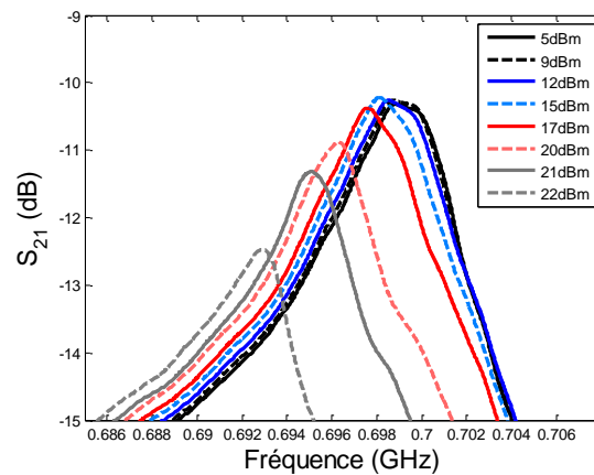
Figure 3-32 Réponse en transmission S_{21} d'un micro-résonateur possédant 40 IDTs et de longueur 140 \mu m pour différents niveaux de puissance d'entrée
