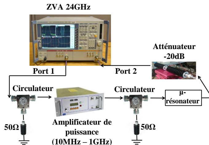
Figure 3-30 : Montage utilisé pour la caractérisation des micro-résonateurs en variant la puissance RF d'entrée
