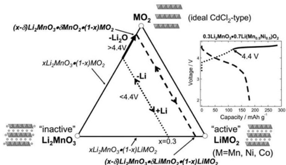
Figure 21 : Diagramme ternaire représentant les domaines d’activité électrochimique des phases x\text{Li}_2\text{MnO}_3 \cdot (1-x)\text{LiMO}_2 , d’après Thackeray et al. 167
