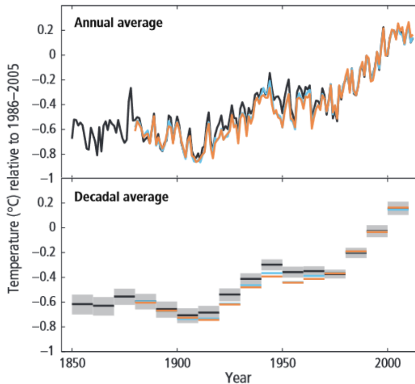
Figure 2 : Evolution de la température surfacique océanique et terrestre entre 1850 et 2012 v
