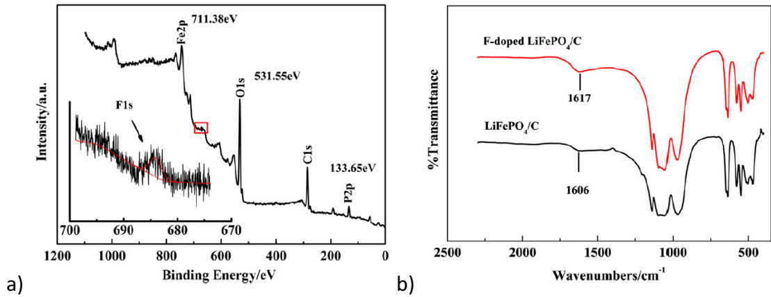
Figure 5 : (a) Analyse XPS de \text{LiFePO}_4 dopé au fluor et (b) analyses FTIR de \text{LiFePO}_4 dopé (rouge) et non dopé (noir) au fluor, d'après Lu et al. 9
