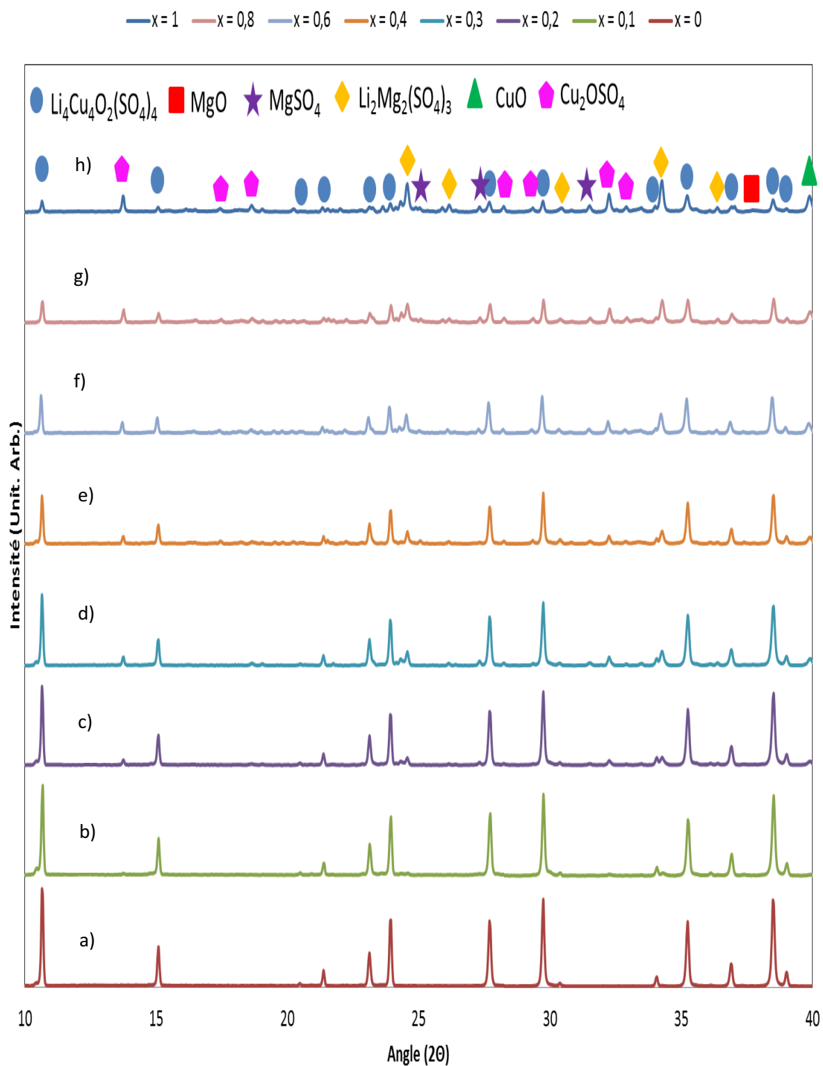
Figure 18 : Diffractogrammes des poudres correspondant aux différentes compositions théoriques \text{Li}_{4-2x}\text{Mg}_x\text{Cu}_4\text{O}_2(\text{SO}_4)_4 \text{Li}_{4-x}\text{Cu}_4\text{O}_{2-x}(\text{SO}_4)_4\text{F}_x , avec x=0 (a) ; 0,1 (b) ; 0,2 (c) ; 0,3 (d) ; 0,4 (e) ; 0,6 (f), 0,8 (g) et 1 (h)
