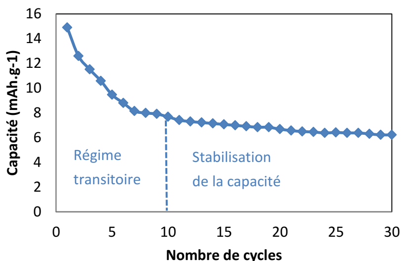
Figure 33 : Cyclage galvanostatique avec limitation en potentiel (GCPL) de \text{Li}_4\text{Cu}_4\text{O}_2(\text{SO}_4)_4 préparé par voie nitrates à 550°C (2x24h) – C/10 – \text{LiPF}_6 1M dans EC/DEC 1:1 (v:v)
