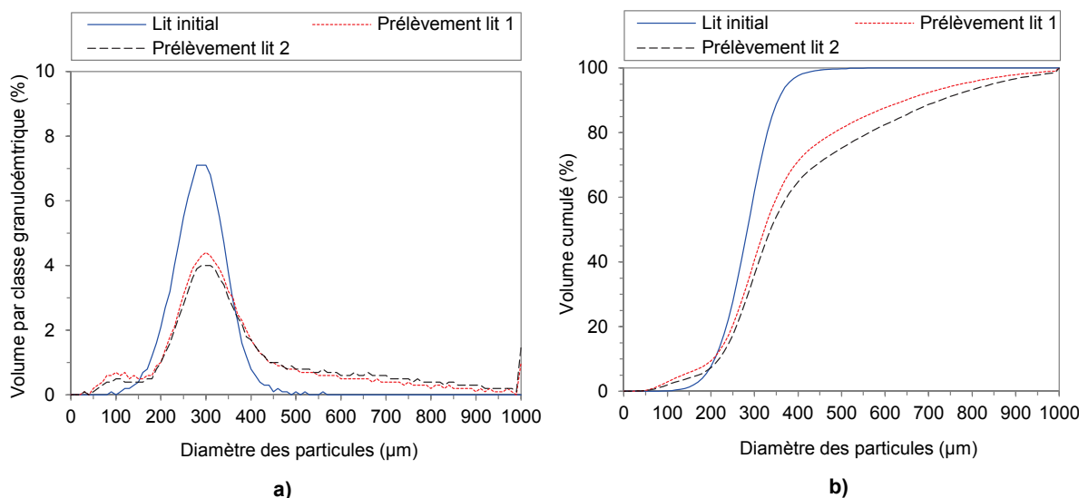
Figure 81. Comparaison de la distribution granulométrique des prélèvements de lit après l'essai de gazéification de paille de blé à échelle pilote par rapport à la granulométrie initiale du lit : a) Répartition en volume par classe granulométrique, b) Répartition en volume cumulé.
