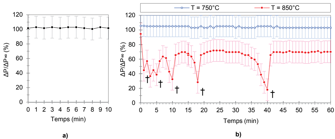
Figure 57. Evolution de la perte de charge du lit fluidisé au cours du temps : a) sans cendres à 850^\circ\text{C} , b) avec cendres (0,4 % massique de lit) à 750^\circ\text{C} et 850^\circ\text{C} († : mélange manuel du lit à l'aide d'une tige métallique, cette opération est réalisée lorsque la défluidisation complète du lit est visuellement observée)
