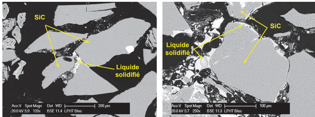
Figure 74. Coupes transversales d'agglomérats observés par MEB et provenant de l'essai de gazéification de paille de blé à échelle pilote dans un lit de SiC (observations réalisées en contraste de phase chimique).
