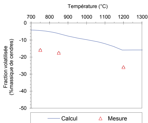
Figure 33. Evolution de la perte de masse des cendres en température : comparaison des valeurs mesurées et calculées à l'équilibre thermodynamique (en % massique de cendres)
