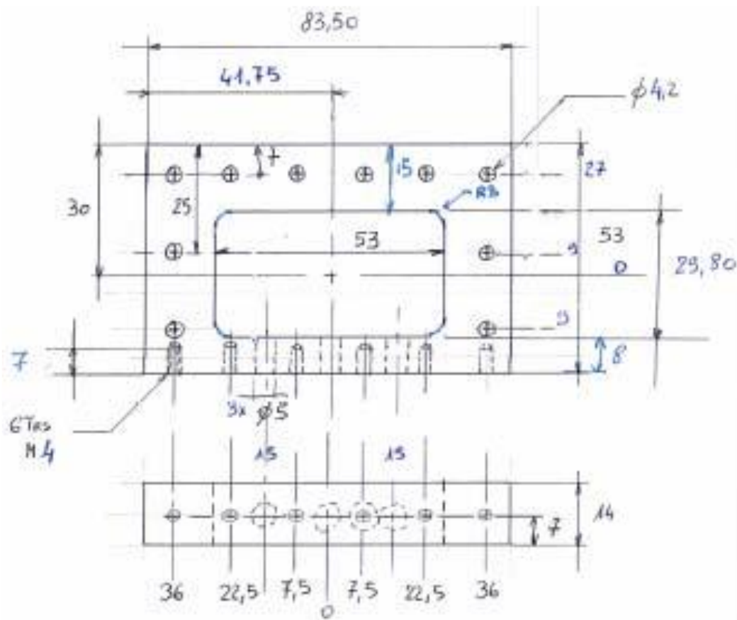
Figure A 3 : Schéma du cadre de double confinement avec sa tranche permettant une entrée latérale du faisceau. Dimensions en mm
