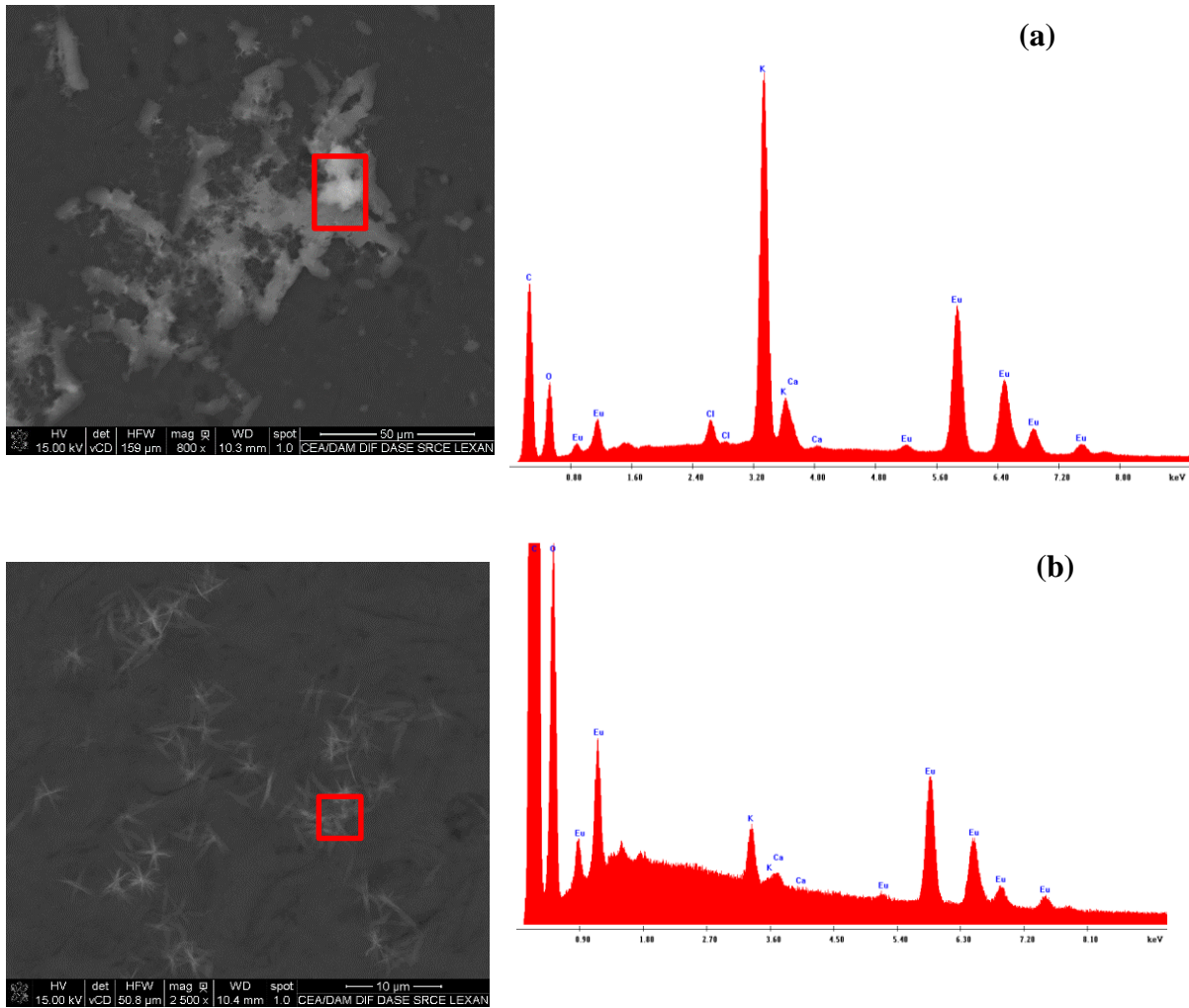
Figure 32 : Analyses MEB/EDX de la solution d'eau milliQ en présence de K^2CO_3 à 2,2 \cdot 10^{-3} M dopée en europium à 5 \cdot 10^{-5} M pH=7,8.
