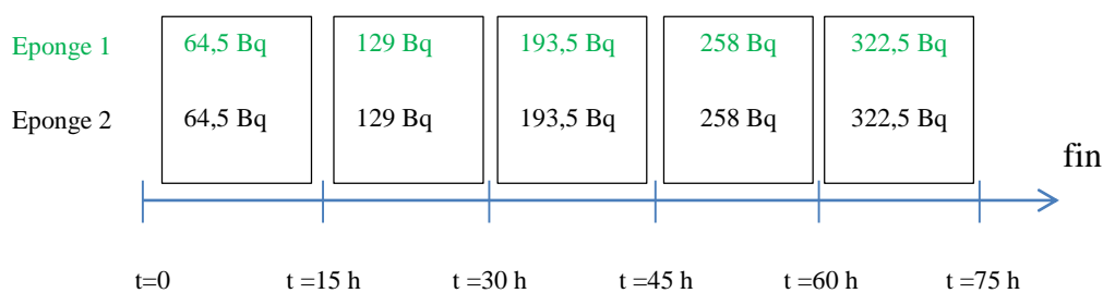
Figure 41: Schéma de l'expérience de contamination en aquarium des 2 éponges en américium avec les quantités cumulées introduites pour les deux éponges.
