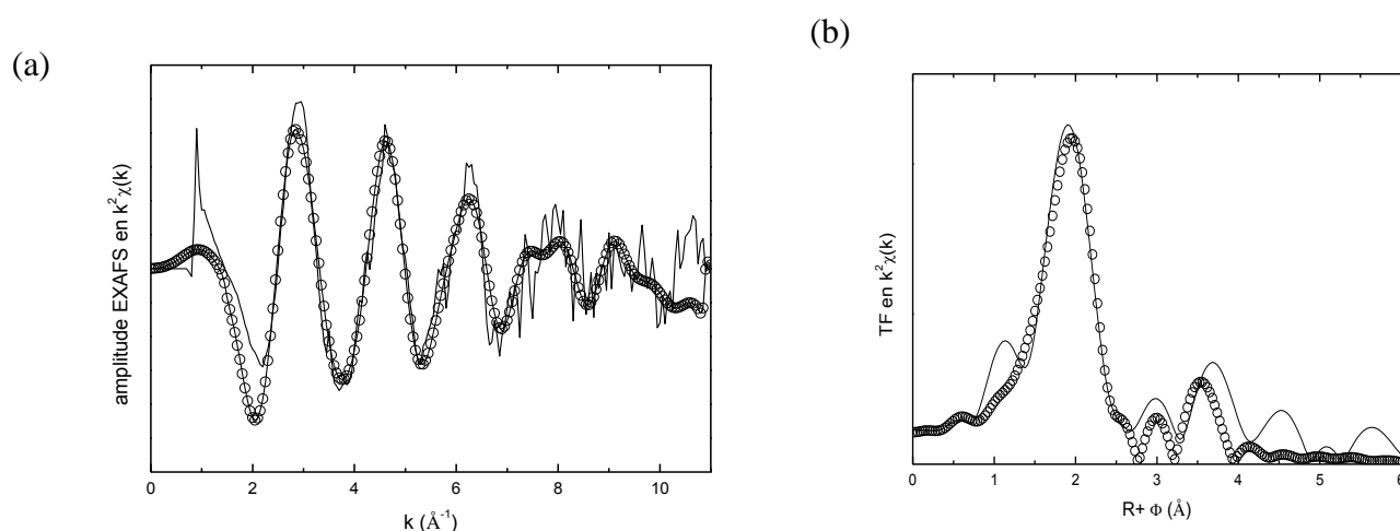
Figure 35 : Spectre EXAFS (a) et transformée de Fourier (b) correspondant au seuil L_{III} de l'euprium de la solution d'eau de mer dopée à 5.10^{-5} M. Spectre expérimental en traits pleins et ajustement en pointillés.
