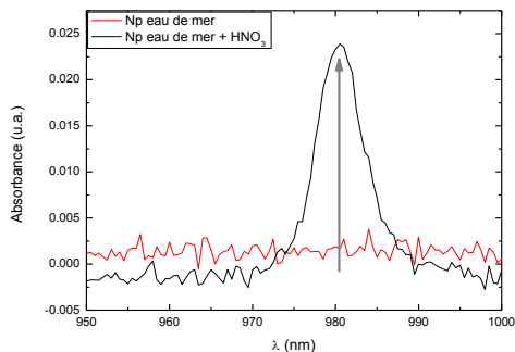
Figure 73 : Spectres UV-visible de la solution d'eau de mer dopée en neptunium à 5.10^{-5} M avec ajout d'acide concentré.
