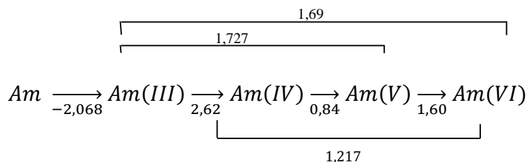
Figure 6 : Potentiels standard des couples de l'américium en milieu acide perchlorique 1M d'après [4]
