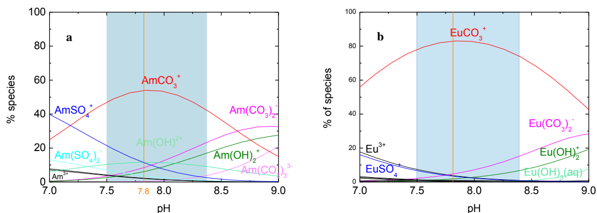
Figure 28 : Diagrammes de spéciation de l'américium (a) et de l'euprium (b) dans l'eau de mer à 5.10^{-5} M
