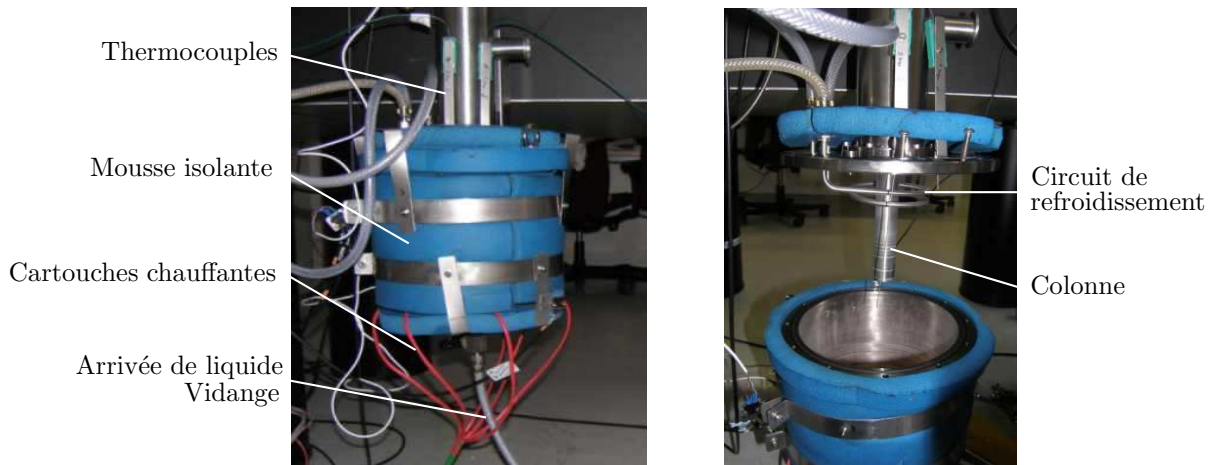
FIGURE 2.2. – Réservoir.
