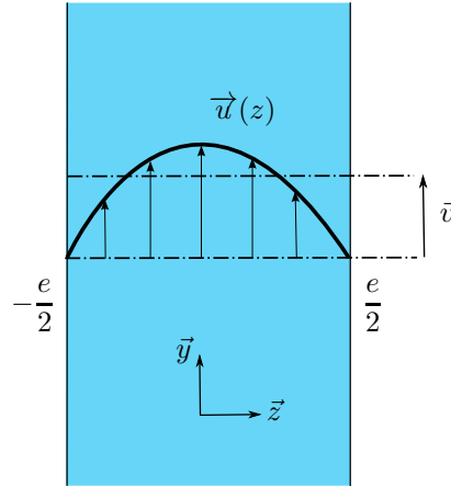
FIGURE 4.2. – Profil de vitesse laminaire dans le canal, selon l'orientation des axes définie au paragraphe précédent, pour un ménisque ascendant.
