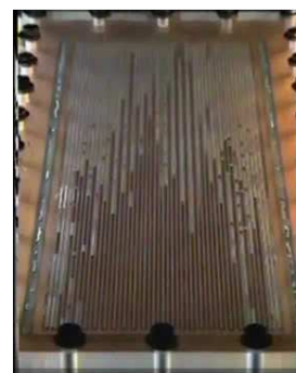
(c) PHP plat, extrait de [85]. Les bouchons de liquide apparaissent en noir.
