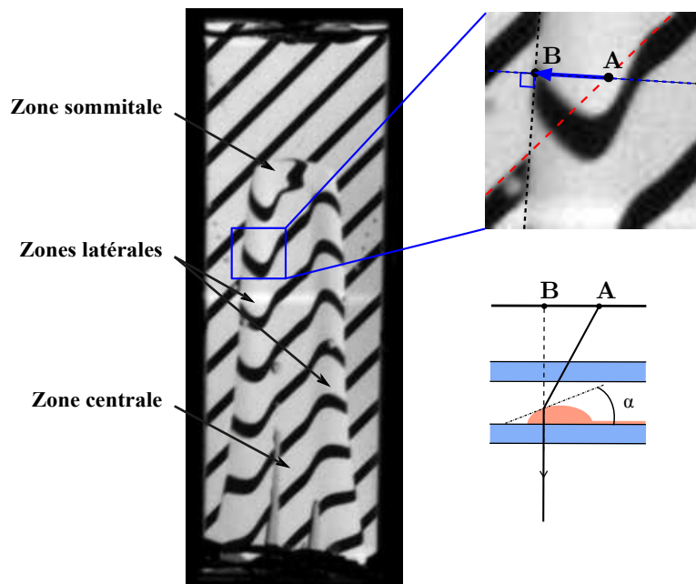
FIGURE 3.3. – Repérage des différentes zones caractéristiques du film sur une image issue de la caméra. Droite : exemple d'un point objet et de son image décalée.
