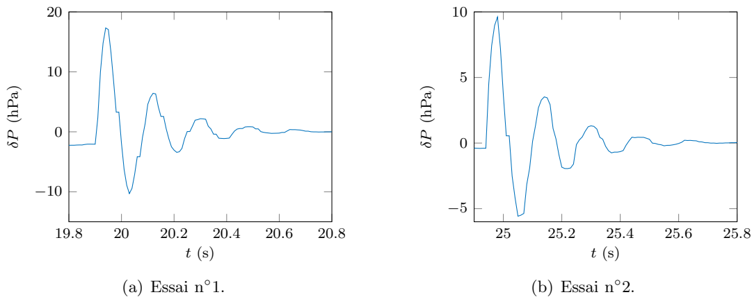
FIGURE 4.7. – Oscillations amorties de la pression dans la bulle, pour les deux essais.
