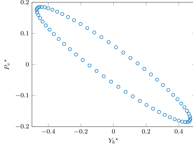
FIGURE D.5. – Diagramme de Clapeyron des fondamentales de P_v^* et Y_b^* .
