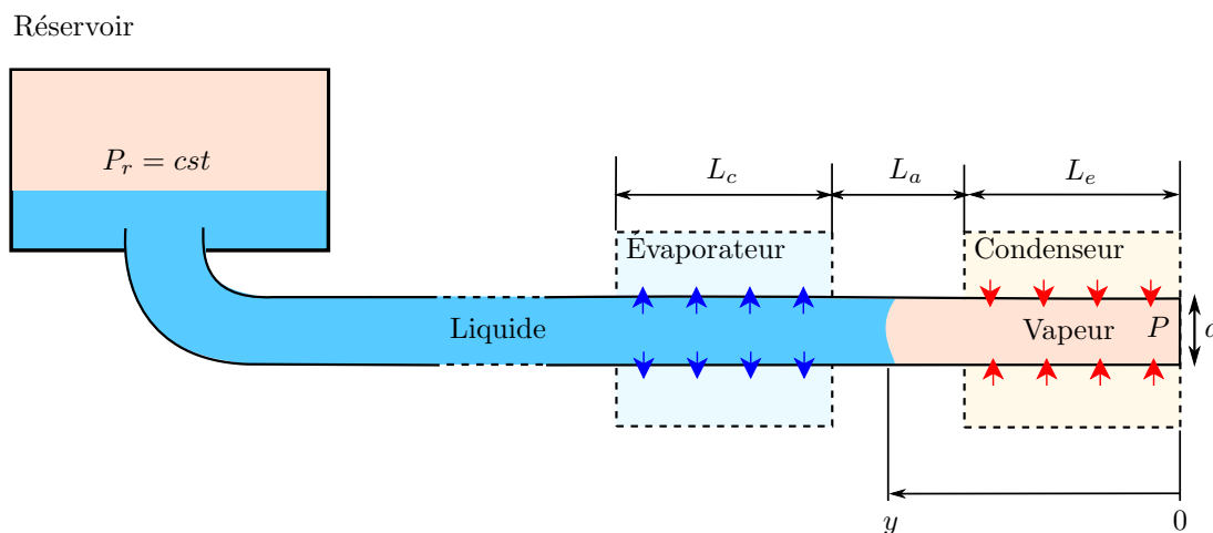
FIGURE 1.10. – Schéma d'un dispositif de PHP monobranche, destiné à l'étude des phénomènes physiques gouvernant le fonctionnement global du PHP.
