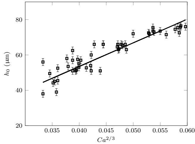
FIGURE 5.4. – Épaisseur du film liquide juste après son dépôt par le ménisque, en conditions d'oscillation auto-entretenue, en fonction du nombre capillaire Ca . Le trait noir plein représente l'équation (5.6), calculée avec \sigma = 22,3 \cdot 10^{-3} \text{ N} \cdot \text{m}^{-1} , \mu = 7,9 \cdot 10^{-4} \text{ Pa} \cdot \text{s} .
