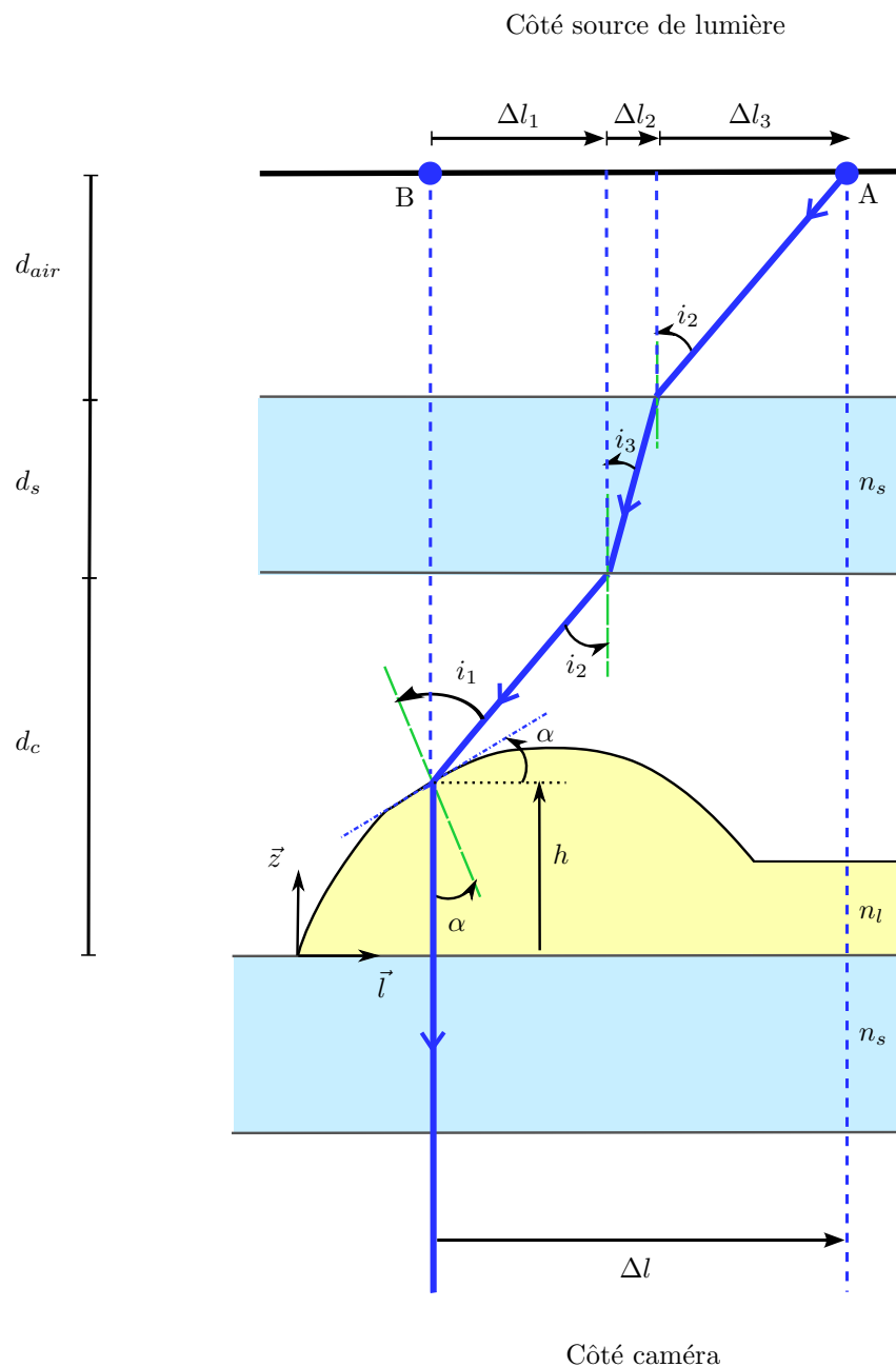
FIGURE 3.4. – Chemin du rayon lumineux dans le plan (\vec{l}, \vec{z}) orthogonal à la ligne triple. Le schéma n'est pas à l'échelle : en réalité, la distance d_{air} est très grande devant d_s et d_c .
