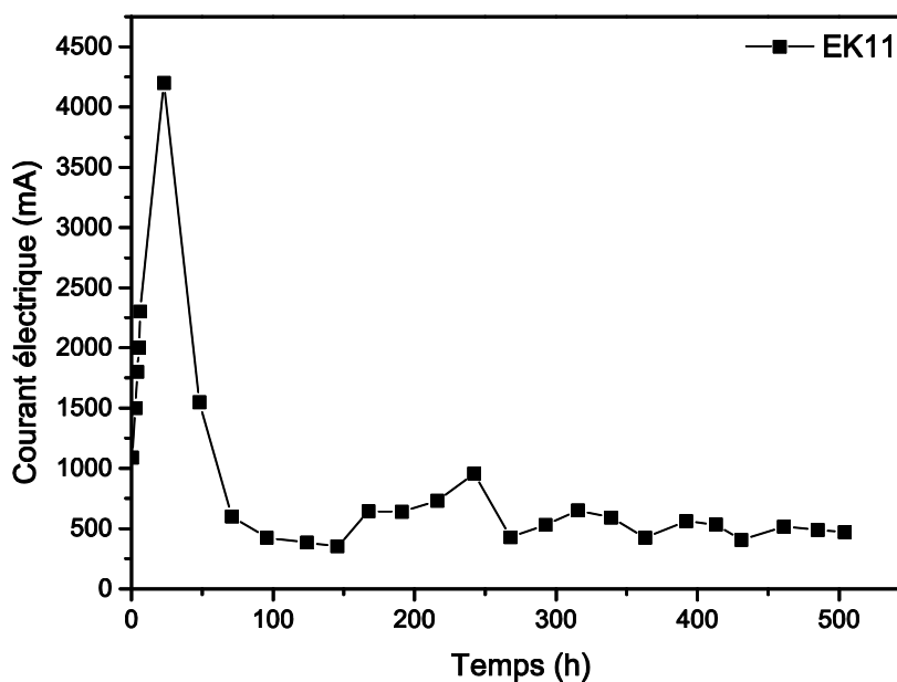
Figure III-31 : Évolution de l'intensité du courant électrique en fonction du temps pour EK11
