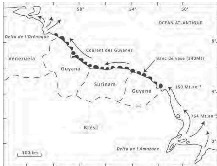
Figure 15: Décharge sédimentaire sur les 1500 km de côte des Guyanes de l'estuaire de l'Amazone à celui de l'Orénoque. Les sédiments déversés par l'Amazone sont en partie accolés à la côte sous forme de bancs de vase migrants vers le nord-ouest poussés par les courants côtiers. Inspiré de Froidefond et al. (1988).
