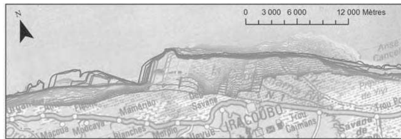
Figure 29: Cartes des fluctuations du trait de côte à mangrove dans la région d'Iracoubo. L'enveloppe de fluctuation maximale est d'environ 6000 m. Même légende que la Figure 17.
