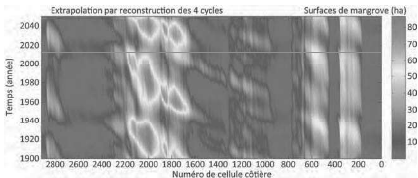
Figure 42: Extrapolation dans le passé et le futur des surfaces de mangrove à partir d'une reconstruction fondée sur les 4 cycles présentés en Figure 41. La ligne rouge indique la situation actuelle en 2014.
