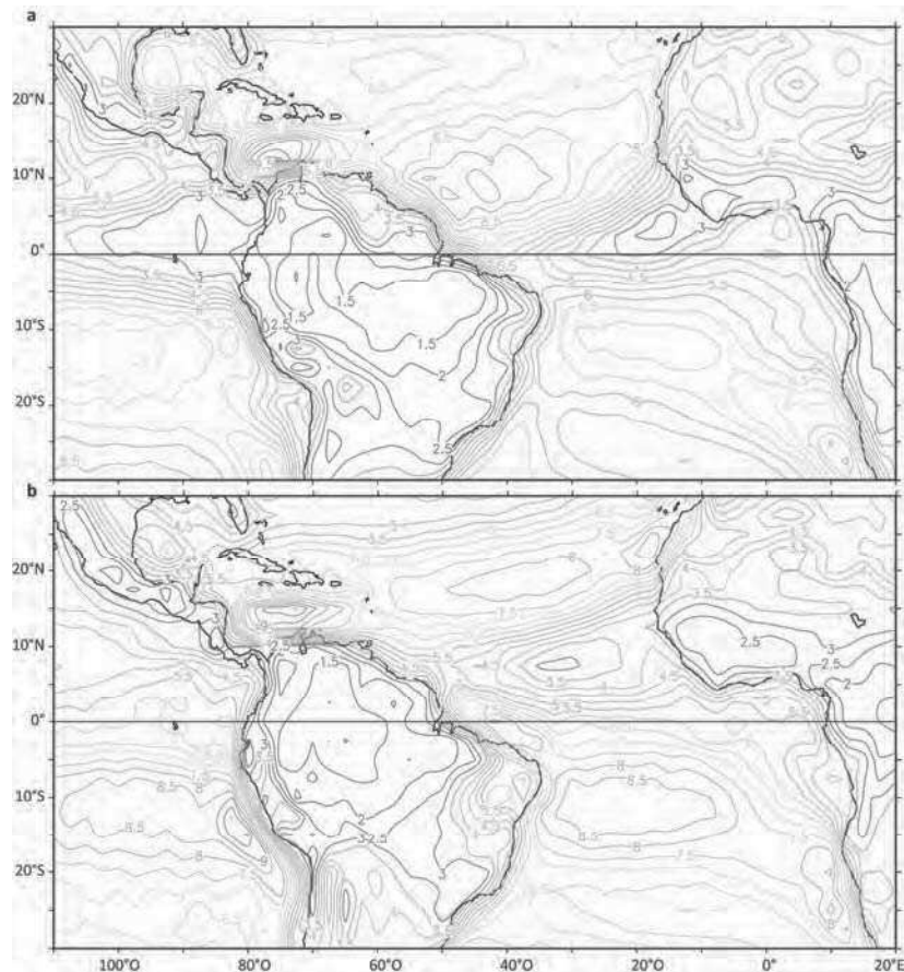
Figure 11: Carte des vents de surface exprimée en mètre par seconde (m.s) sur la période 1968-1996. a) Moyenne d'hivers (J-F-M). b) Moyenne d'été (J-A-S). Données obtenues sur http://www.esrl.noaa.gov/psd/data/gridded .
