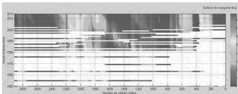
Figure 24: Diagramme de Hovmöller des surfaces de mangrove avant interpolation. Les données manquantes sont affichées en blanc.
