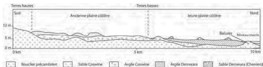
Figure 8: Coupe des strates lithologiques de la plaine côtière de Guyane. D'après Prost (1989).
