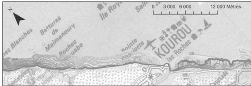
Figure 31: Carte de la fluctuation du trait de côte à mangrove dans la région de Kourou. Le trait de côte n'a fluctué que dans les années 1980-1990 (jaune-orange). Sur la rive droite du Kourou, le trait de côte a recommencé à fluctuer dans les années 2000-2010 (rouge). L'enveloppe de fluctuation maximale est d'environ 2500 m. Même légende que la Figure 17.
