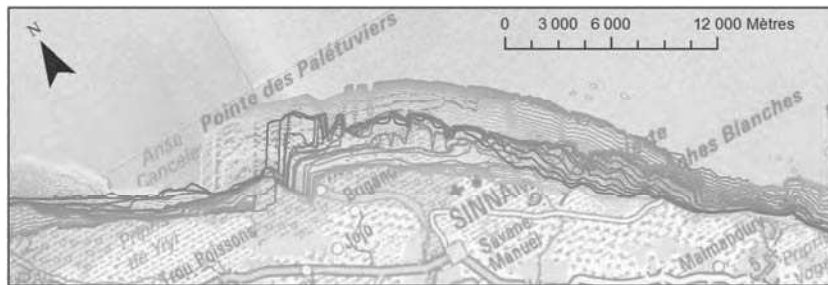
Figure 30: Carte de la fluctuation du trait de côte à mangrove dans la région de Sinnamary. L'enveloppe de fluctuation maximale est d'environ 4000 m sur la rive droite. Même légende que la Figure 17.
