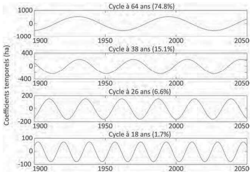
Figure 41: Projection sur la période 1900-2050 des 4 cycles côtiers détectés par la décomposition en fonction empiriques orthogonales complexes (CEOF). Le cycle à 64 ans, 38 ans, 26 ans et 18 ans correspondent respectivement au mode 1 ( R^2 = 0,93 ), mode 2 ( R^2 = 0,86 ), mode 3 ( R^2 = 0,97 ) et mode 4 ( R^2 = 0,84 ). Ils représentent respectivement 74,8%, 15,1%, 6,6% et 1,7% de la variabilité totale du jeu de données, soit environ 98%.
