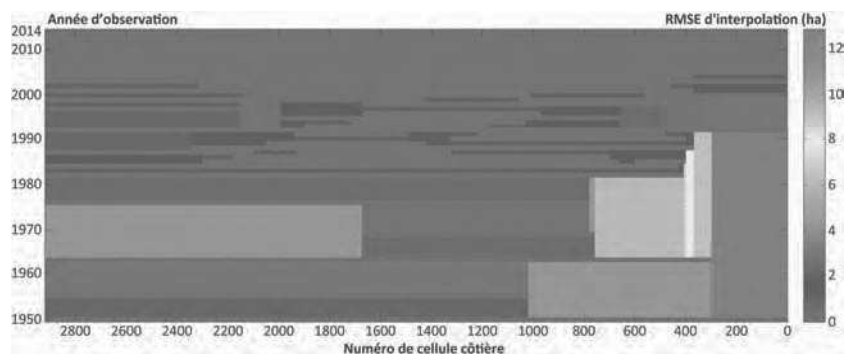
Figure 26: Erreurs quadratiques moyennes (RMSE) liées à l'interpolation temporelle des données de surfaces de mangrove manquantes.
