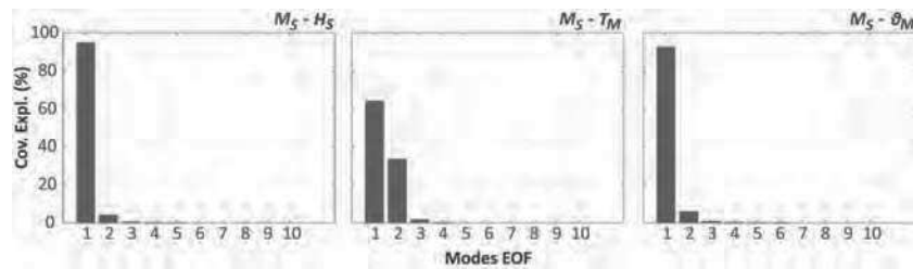
Figure 52: Taux de covariance expliquée par les modes SVD sur les couples surfaces de mangroves ( M_S ) et hauteurs significatives ( H_S ), surfaces de mangroves ( M_S ) et périodes moyennes ( T_M ) et surfaces de mangroves ( M_S ) et directions moyennes ( \theta_M ) des vagues d'hiver en Atlantique Nord.
