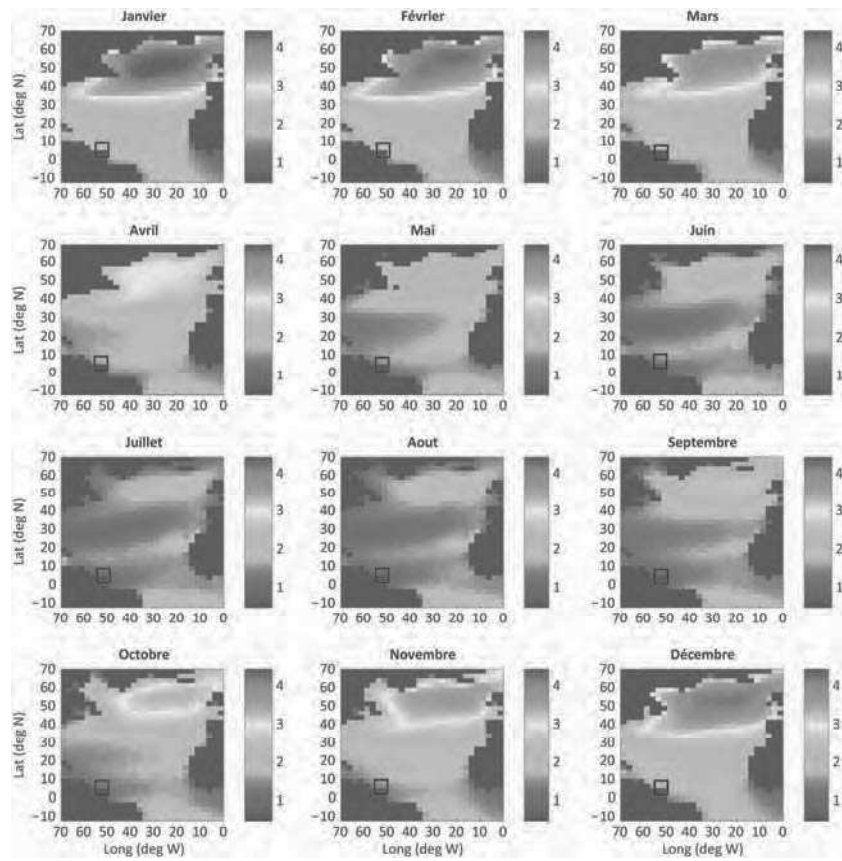
Figure 44: Climatologie mensuelle des hauteurs significatives de vagues ( H_s ) exprimées en mètres dans l'Atlantique Nord sur la période 1958-2002. Le carré noir indique la position de la Guyane.
