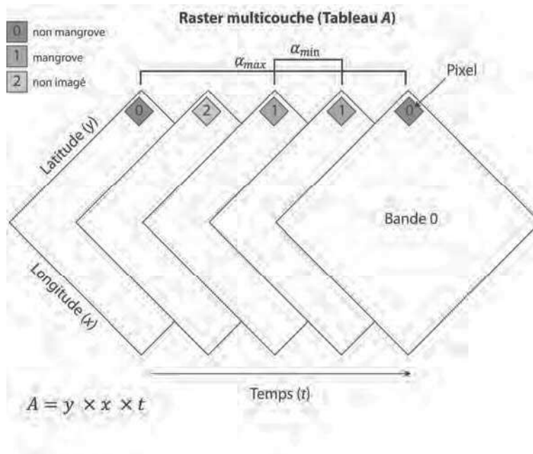
Figure 62: Schématisation de l'algorithme de détermination de l'âge de mangrove théorique à partir d'un raster multicouche. Le raster est importé sous la forme du tableau A. Les âges théoriques minimum ( \alpha_{min} ) et maximum ( \alpha_{max} ) sont calculés en comptant le nombre de cellules dans la dimension temporelle ( t ).
