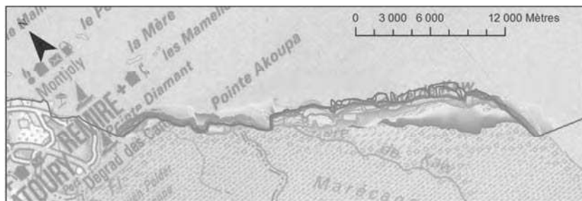
Figure 33: Carte de la fluctuation du trait de côte à mangrove dans la région de Kaw. L'enveloppe de fluctuation maximale est d'environ 4500 m sur la rive gauche de l'estuaire de l'Approuague. Même légende que la Figure 17.
