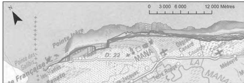
Figure 28: Carte des fluctuations côtières dans la région de Mana. L'enveloppe de fluctuation maximale est d'environ 3500 m. La zone a subi une forte tendance à l'érosion depuis 1950 mais progresse de nouveau en face de Mana depuis les années 2000-2010 (orange-rouge). Même légende que la Figure 17.
