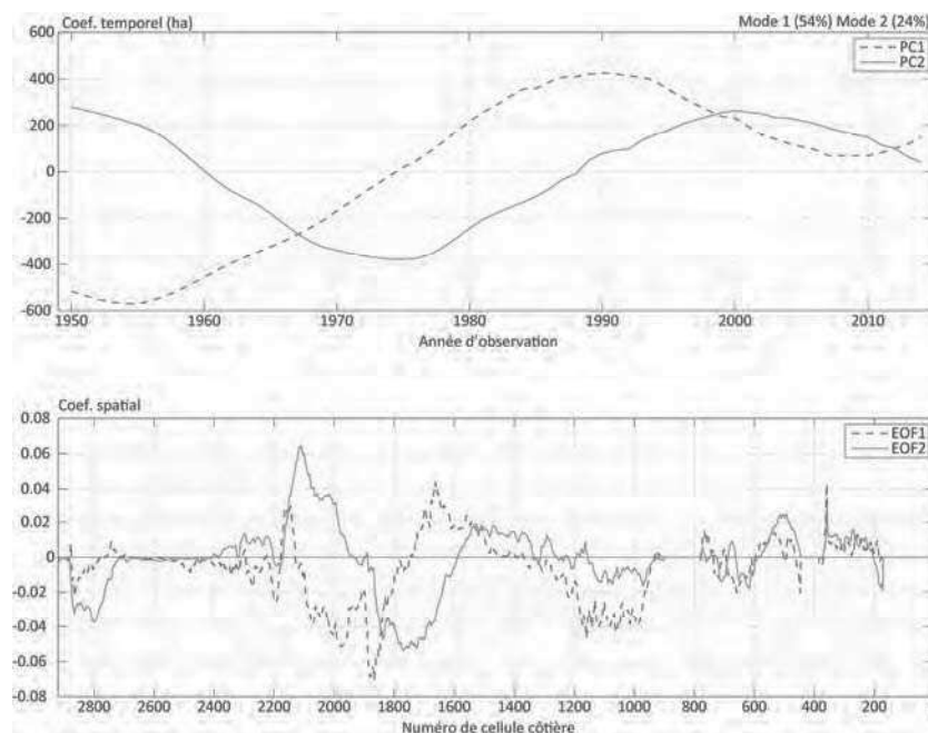
Figure 36: Les 2 premiers modes résultant de la décomposition en Fonctions Empiriques Orthogonales (EOF) du diagramme de Hovmöller des surfaces de mangrove. Pour retrouver la vraie valeur de surface du diagramme, il faut multiplier le coefficient temporel d'une année donnée (haut) par le coefficient de co-variation spatial d'une cellule côtière donnée (dessous) et par le taux de variabilité totale expliquée par le mode (mode 1 = 0,54 et mode 2 = 0,24) et ajouter la moyenne temporelle de cette cellule.
