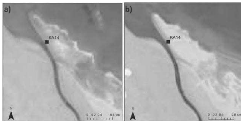
Figure 63: Datation du site d'inventaire forestier KA14 inventorié en 2004. a) Quicklook de l'image satellite Landsat de 1999 (LE72270571999286EDC00) montrant l'absence de végétation sur la parcelle. b) Quicklook de l'image satellite Landsat de 2000 (LE72270572000209EDC00) montrant la présence de végétation sur la parcelle. On déduit que l'installation de la mangrove sur la parcelle inventoriée en 2014 n'avait pas moins de 4 ans et pas plus de 5 ans.
