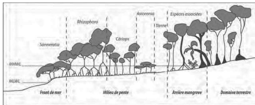
Figure 2: Exemple de zonation des espèces sur un gradient terre-mer. Coupe schématique des faciès de mangroves dans le fond de la baie de Bouéni, Mayotte. Le niveau moyen des plus basses mers (MLWL) et le niveau moyen des plus hautes mers (MHWL) sont indiqués. Le gradient de salinité du sol augmente en remontant la pente.
