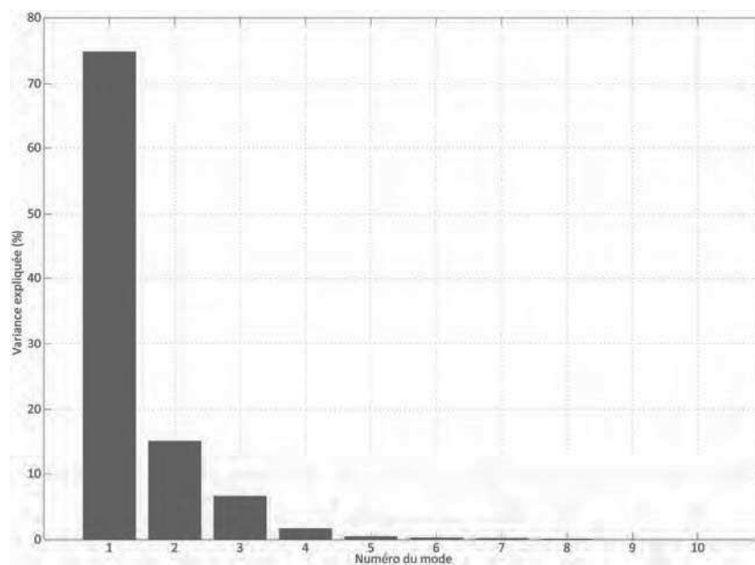
Figure 37: Part de la variance expliquée (%) par chacun des modes issues de la décomposition en Fonctions Empiriques Orthogonales Complexes (CEOF).
