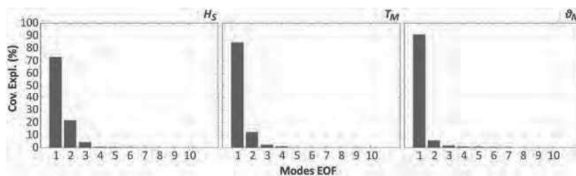
Figure 48: Taux de covariance expliquée par les modes EOF sur les hauteurs significatives ( H_S ), les périodes moyennes ( T_M ) et les directions moyennes ( \theta_M ) des vagues d'hiver en Atlantique Nord.
