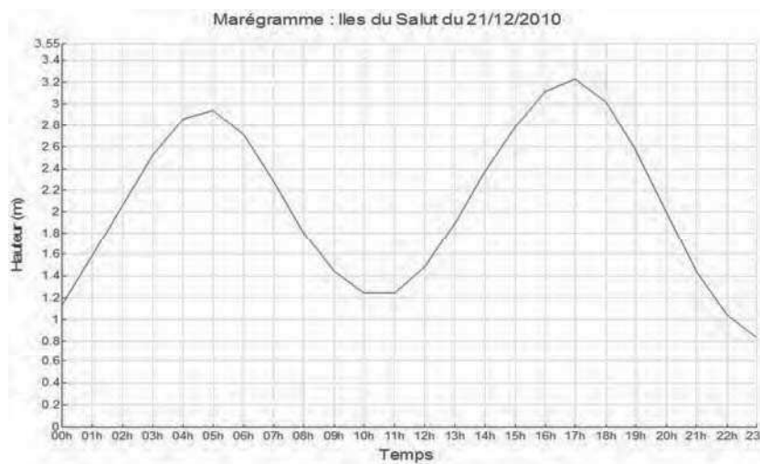
Figure 13: Marégramme du solstice d'hiver 2010 à la station Iles du Salut, Guyane. Données de prédiction issues du Service Hydrographique et Océanographique de la Marine nationale (SHOM).
