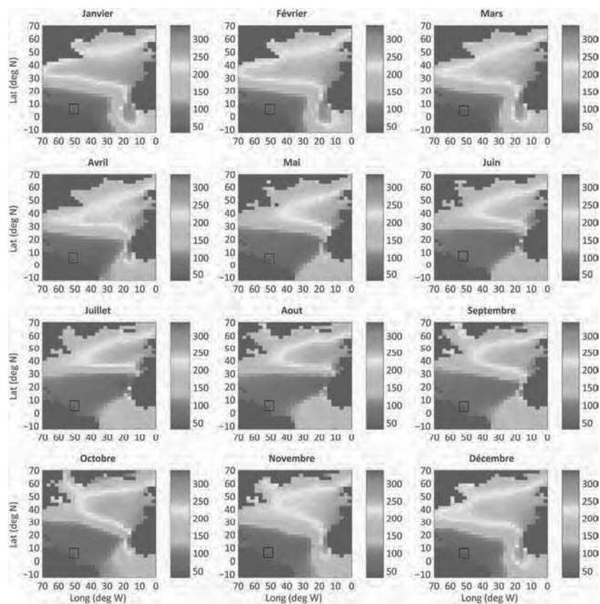
Figure 46: Climatologie mensuelle dans l'Atlantique Nord sur la période 1958-2002 des directions moyennes des vagues ( \theta_M ) exprimées en degrés suivant la convention météorologique, c.à.d. 0^\circ indique « provenant du nord » et 90^\circ « provenant de l'est ». Le carré noir indique la position de la Guyane.
