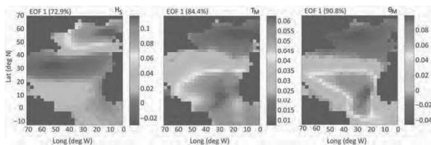
Figure 50: Coefficients spatiaux (EOF) du premier mode de la décomposition en EOF des hauteurs significatives ( H_s ), périodes moyennes ( T_M ) et directions moyennes ( \theta_M ) des vagues d'hiver en Atlantique Nord.
