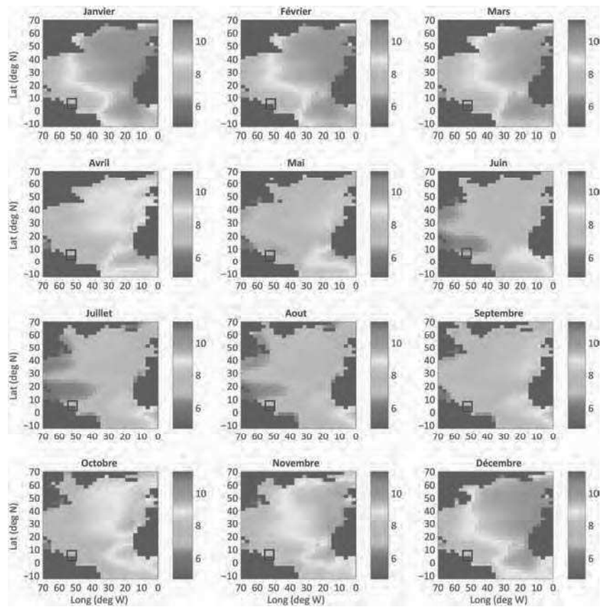
Figure 45: Climatologie mensuelle des périodes moyennes de vagues ( T_M ) exprimées en secondes dans l'Atlantique Nord sur la période 1958-2002. Le carré noir indique la position de la Guyane.
