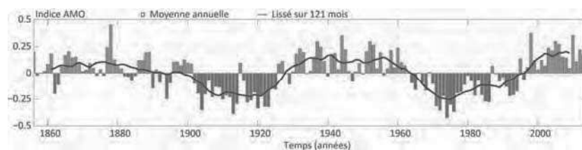
Figure 58: Indice de l'Oscillation Multi-décennale Atlantique (AMO en anglais). Moyennes annuelles de l'indice mensuel (barres) et lissage sur 121 mois. Données fournies par le Earth System Research Laboratory, Physical Science Division de la National Oceanic and Atmospheric Administration (USA).
