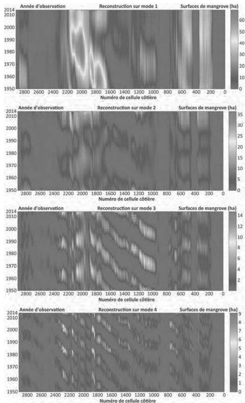
Figure 40: Reconstruction de la matrice à partir chaque mode individuel. Les mode 1, 2, 3 et 4 correspondent respectivement à des cycles de 64, 38, 26 et 18 ans et représentent respectivement 74,6%, 15,1%, 6,6% et 1,7% de la variabilité totale.
