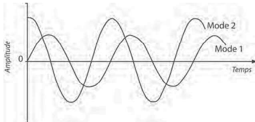
Figure 23: Schematisation d'une quadrature temporelle entre deux modes.
