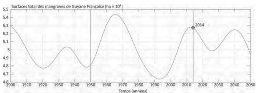
Figure 43: Extrapolation dans le passé et le futur de la superficie totale des mangroves de Guyane à partir d'une reconstruction fondée sur les 4 cycles présentés en Figure 41.
