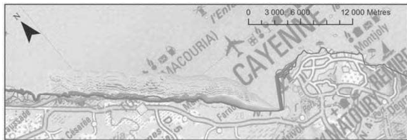
Figure 32: Carte de la fluctuation du trait de côte à mangrove dans la région Tonate-Macouria. L'enveloppe de fluctuation maximale est d'environ 3500 m à l'estuaire de la crique Macouria (la Césarée). En face de Cayenne, le trait de côte à fluctué dans les années 1955, 1985, et 2005 avec une enveloppe maximale de 1000m. Même légende que la Figure 17.
