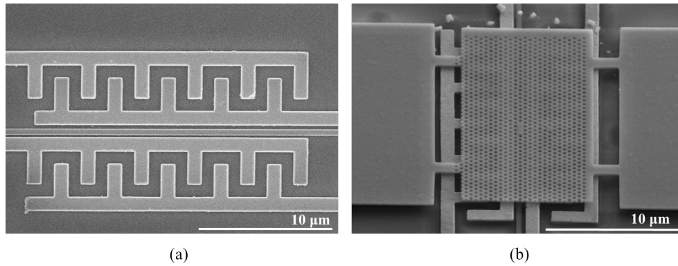
Figure E.6: (a) Électrodes 'interdigitated' avec guide d'ondes sur la même puce (b) le système avec la membrane cristaux photonique suspendu sur électrodes intégrées et guide d'ondes. La membrane contient une cavité L3.
