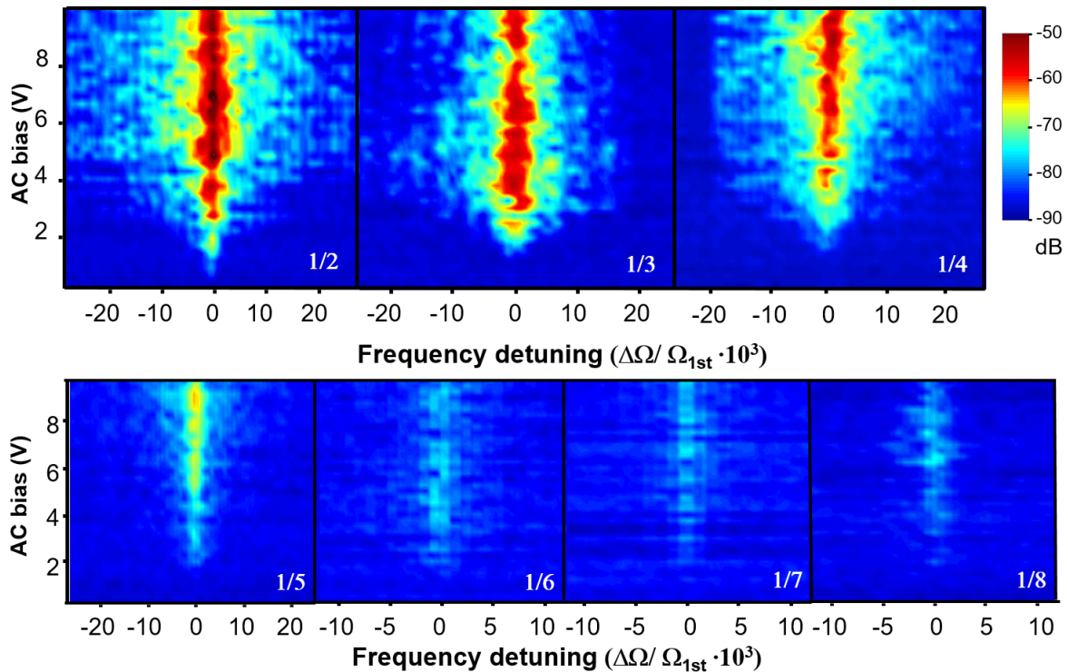
Figure E.4: Super-harmonique réponse générée jusqu'à huitième ordre, il y a des réponses comme 'tongue' qui sont observées avec une tension d'actionnement.
