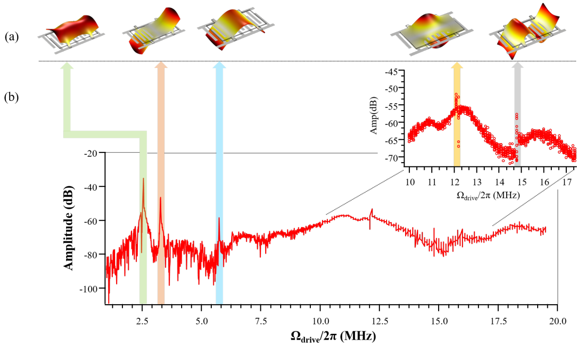
Figure E.2: (a) Simulation MEF de mode mécanique (b) mode mécanique observées avec balayage de fréquence, la tension d'actionnement est maintenue constante.
