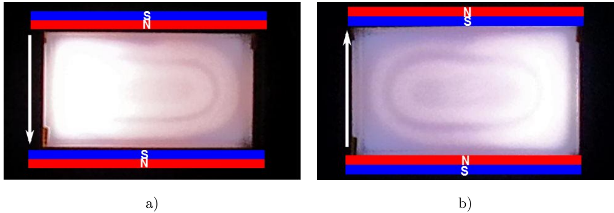
FIGURE 4.30 – Photographies en vue de face de la cavité de PEGASES en SF_6 en configuration a) NS et b) SN (200 W, 10 sccm et 190 G).
