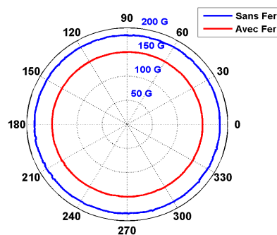
FIGURE 5.6 – Simulation de B en fonction de \theta avec et sans fer pur à r = 30 mm.
