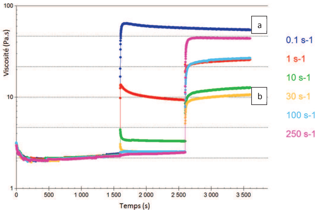
Figure 68 : influence de l'histoire de cisaillement sur la viscosité. Le taux de cisaillement du 2 ème palier est indiqué dans la légende. Teneur en \text{CaCO}_3 : 41% vol.
