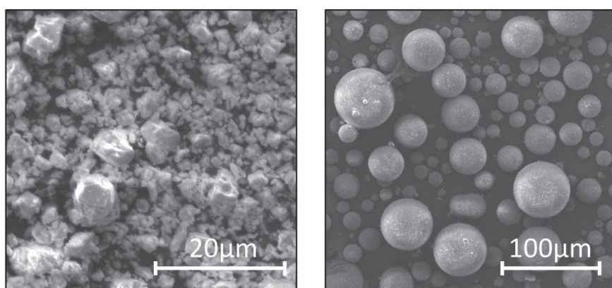
Figure 4 : micrographies MEB de \text{CaCO}_3 (a) et de billes de verre (b) [1]
