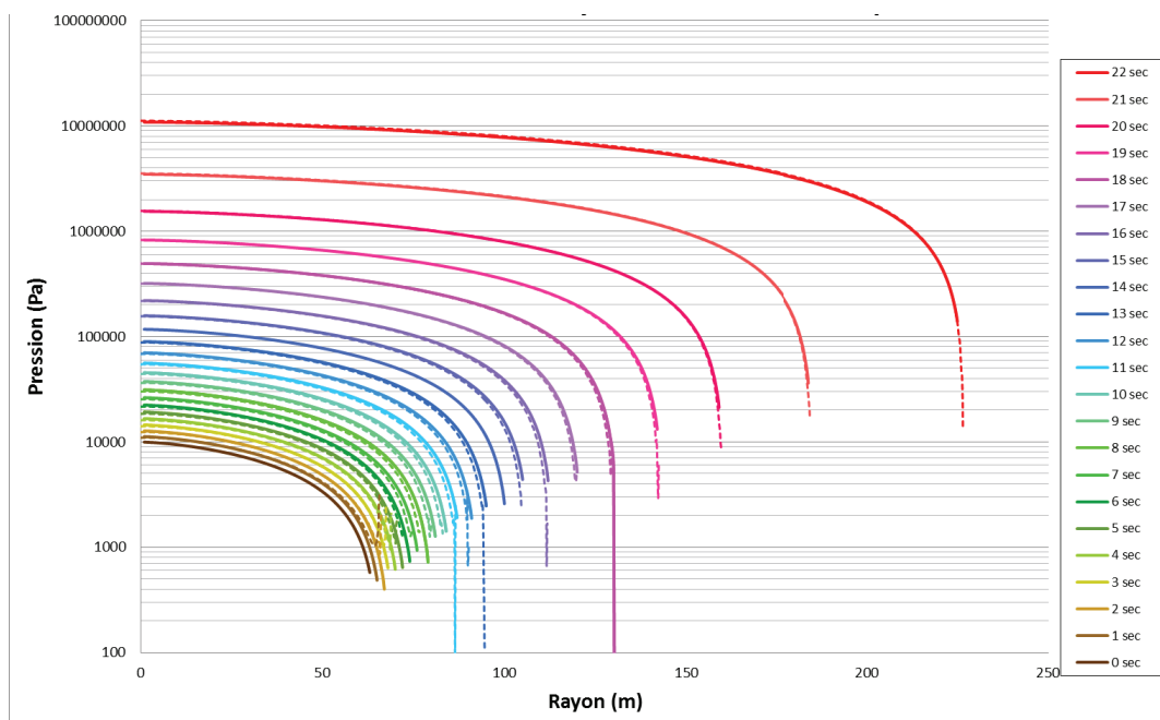
Figure 47 : comparaison calcul analytique/simulation numérique. Pression en fonction du rayon. Les pointillés représentent les résultats de simulation numérique. Les lignes pleines sont ceux obtenus avec Excel.
