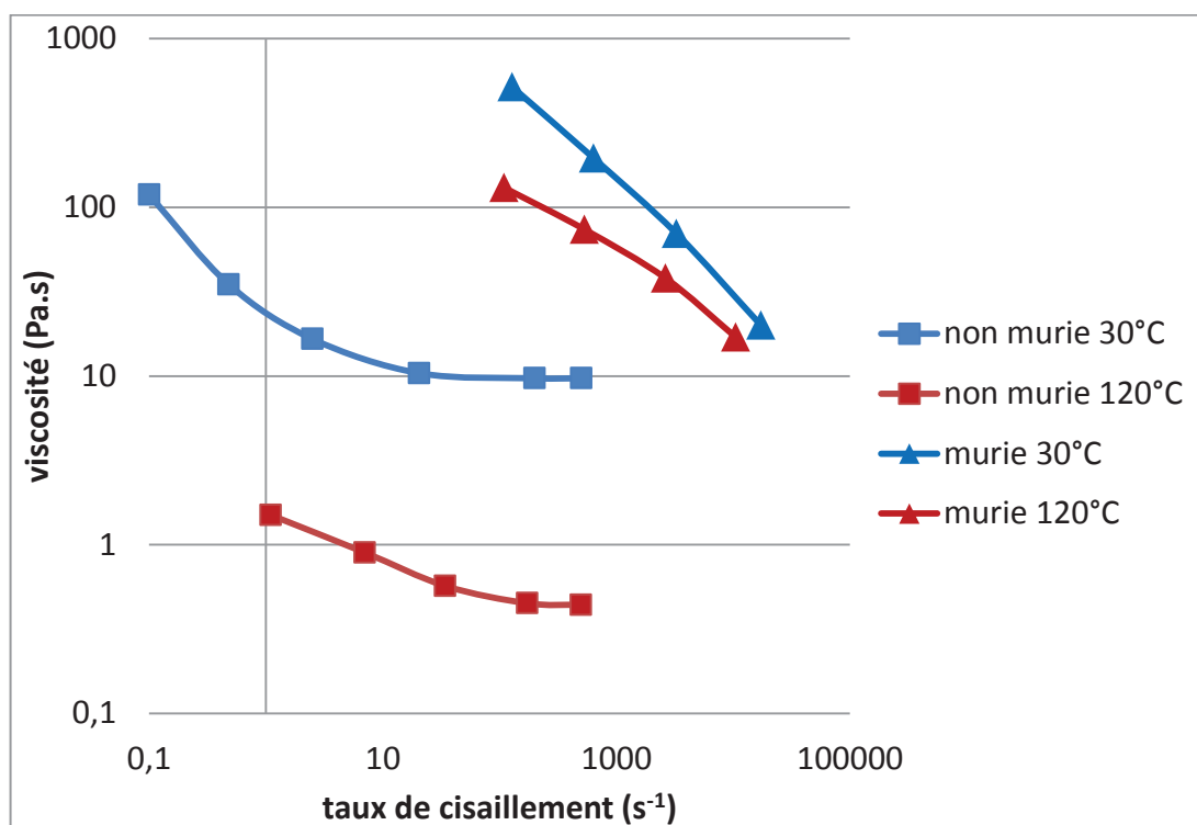
Figure 23 : comparaison des viscosités des pâtes mûries et des pâtes non mûries.
