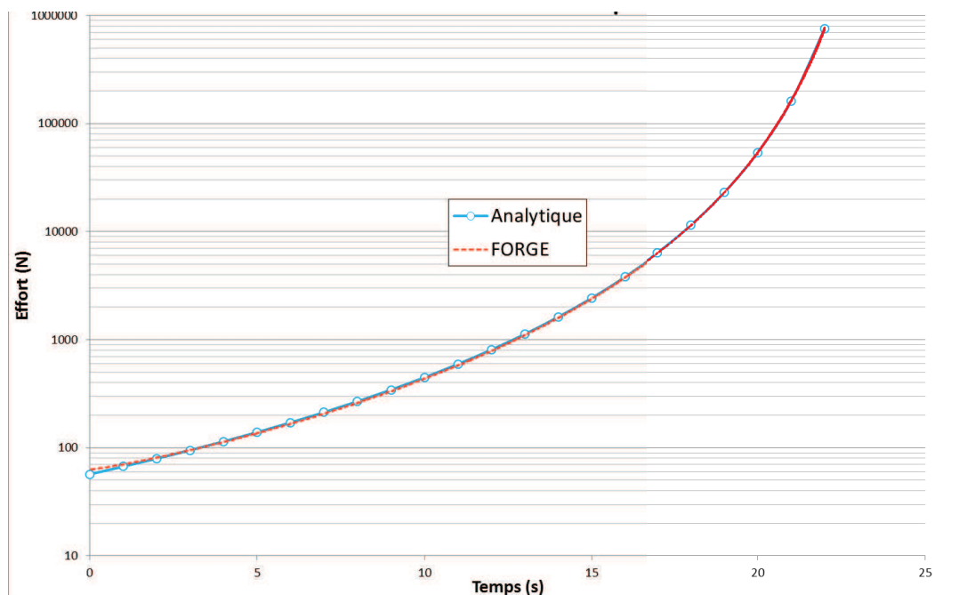
Figure 49 : comparaison calcul analytique/simulation numérique. Force totale en fonction du temps.
