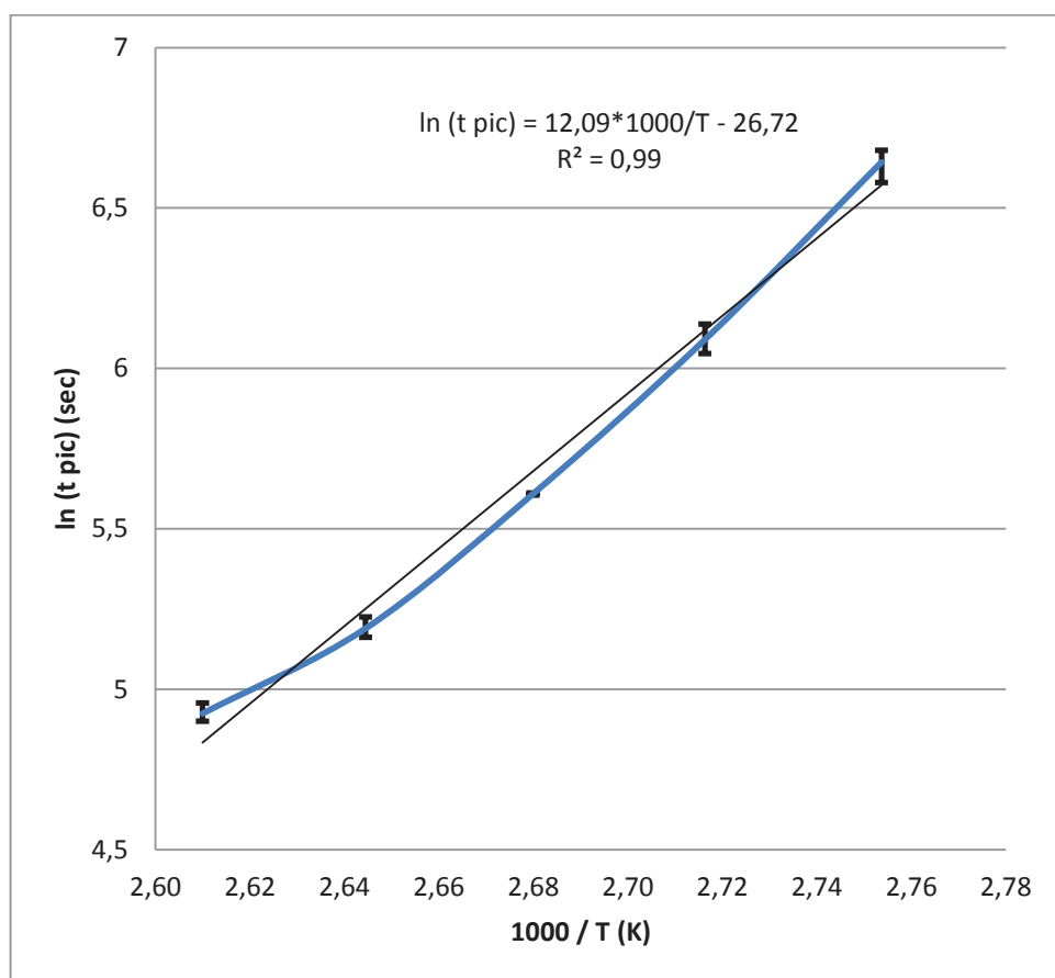
Figure 35 : comportement de type Arrhenius du temps d'apparition du pic exothermique
