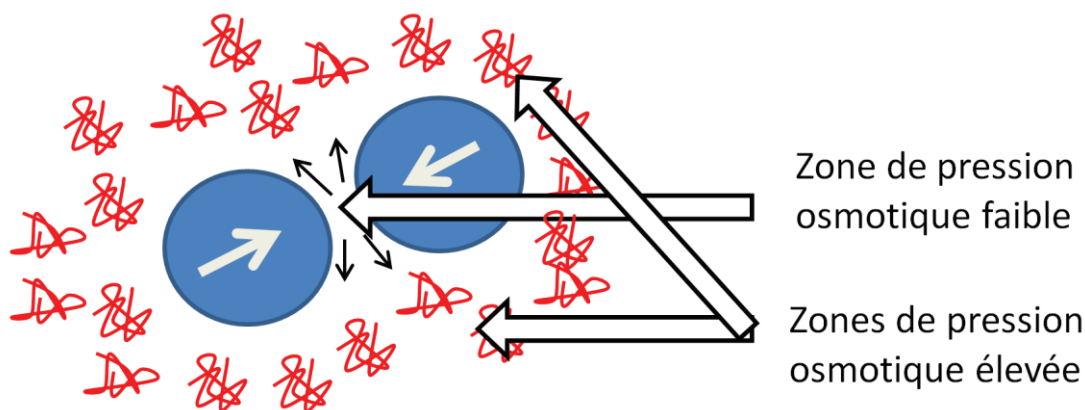
Figure 63 : Flocculation par déplétion. Les chaînes de polymères sont représentées en rouge, les particules sont représentées en bleu.
