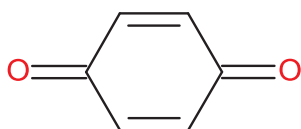
Figure 67 : Para Benzo Quinone (PBQ)
