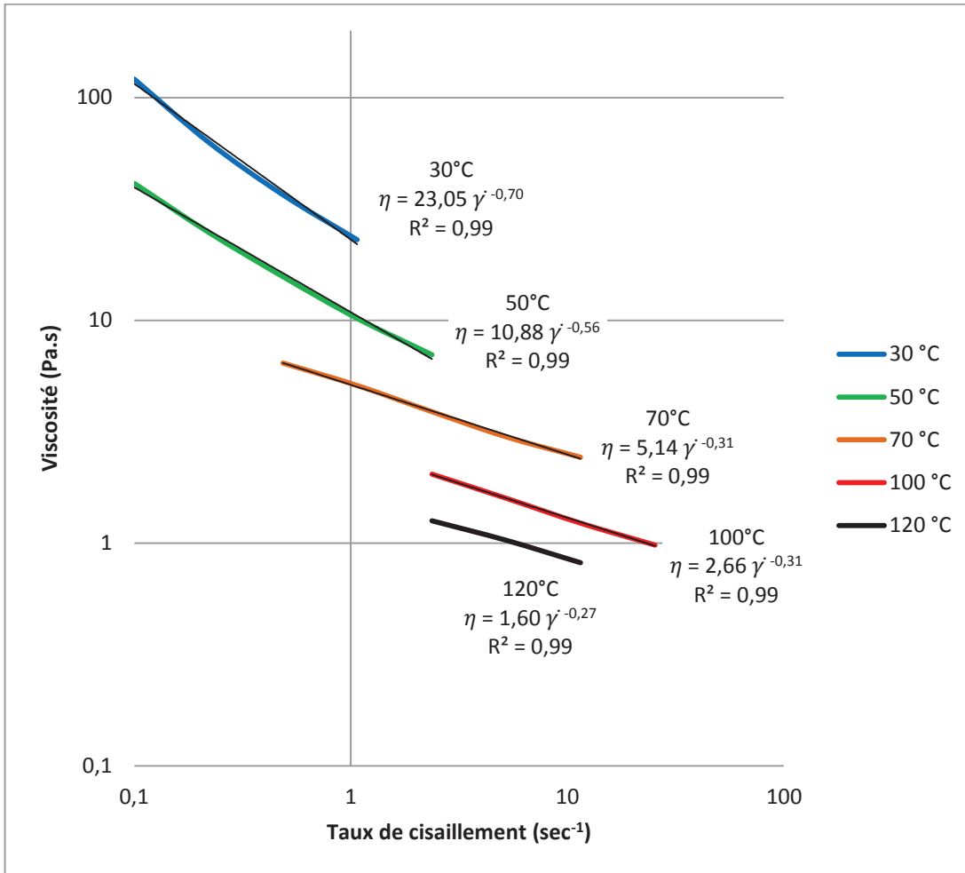
Figure 27 : viscosité dans le domaine rhéo-fluidifiant
