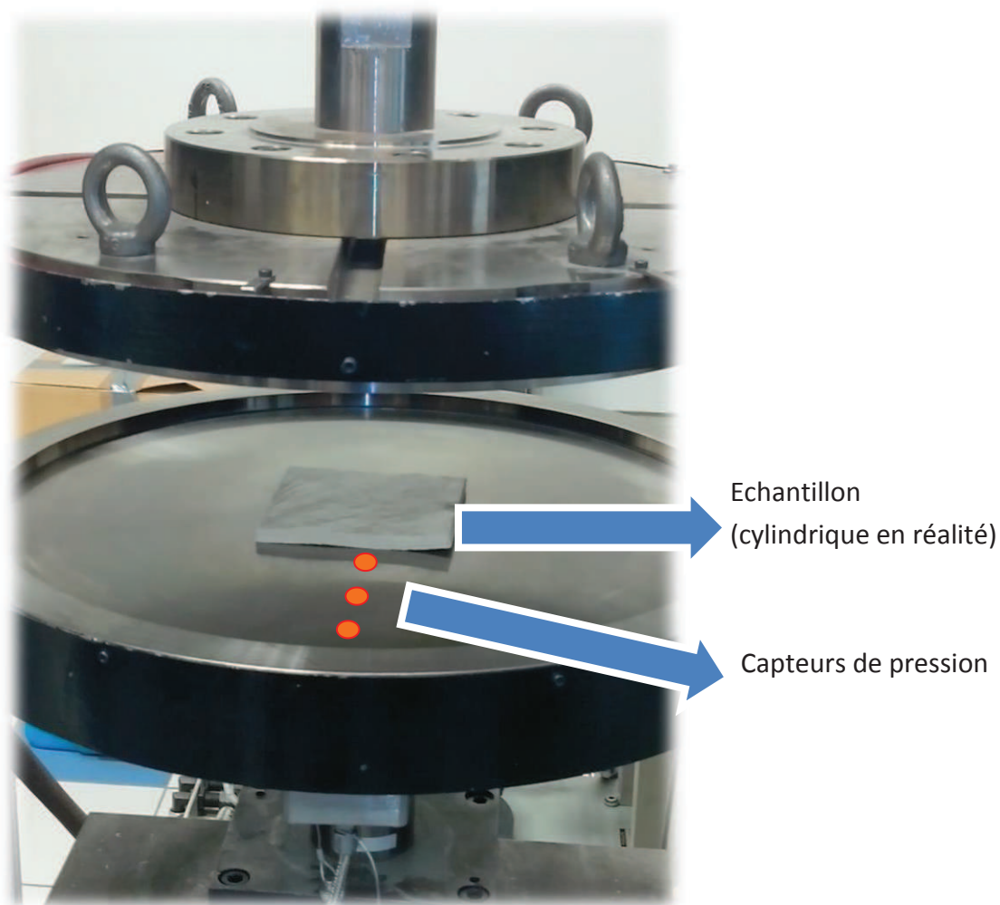
Figure 52 : dynamomètre instrumenté
