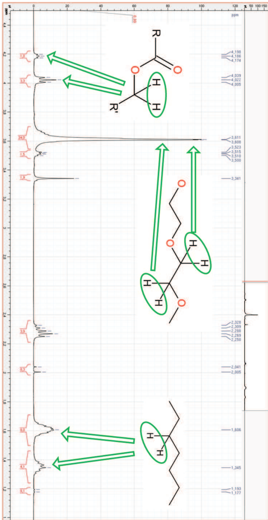
Figure 88 : RMN du proton du BYK W996. Vue détaillée. Solvant : CDCl 3 . 400 MHz.
