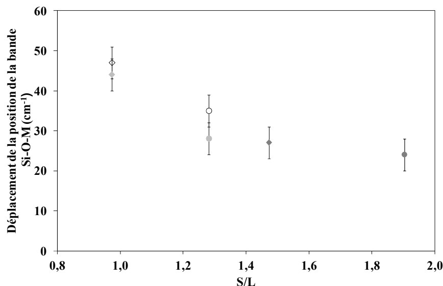
Figure 17 : valeur de déplacement de la position de la bande Si-O-M en fonction du rapport solide / liquide (S/L) pour les échantillons (◇) S_K1M1 , (◆) S_K1M1_{0,8}G_{0,2} , (◆) S_K1M1_{1,0}G_{0,2} , (○) S_K3M1 , (●) S_K3M1_{0,8}G_{0,2} et (●) S_K1M1_{1,0}G_{0,2} .
