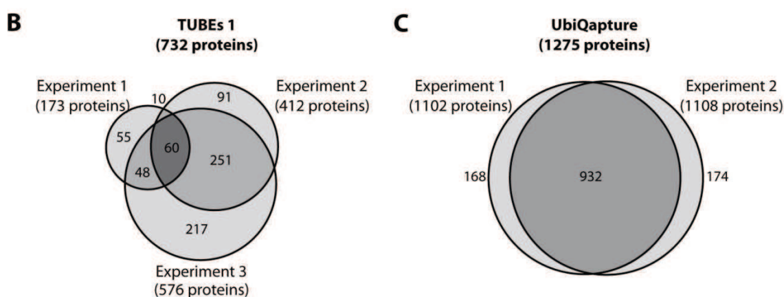
Figure 3: 1641 protéines ubiquitylées sont identifiées par spectrométrie de masse dans le foie de souris avec une grande reproductibilité entre les expériences
