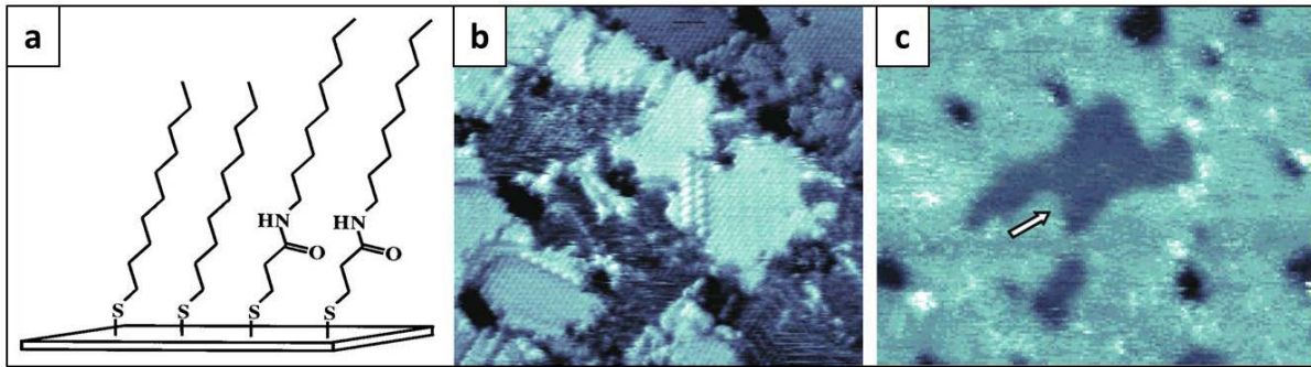
Figure 2. (a) Représentation schématique des SAMs étudiées contenant le décane-1-thiol et la 3-mercaptopropyl-N-nonylpropionamide. (b) Cliché STM (300 x 300 Å) d'une SAM obtenue par coadsorption d'une solution équimolaire de HS(CH 2 ) 9 CH 3 et de HS(CH 2 ) 2 CONH(CH 2 ) 8 CH 3 . (c) Cliché STM (515 x 475 Å) d'une SAM obtenue par coadsorption d'une solution 1:3. D'après [Smith, 2001].
