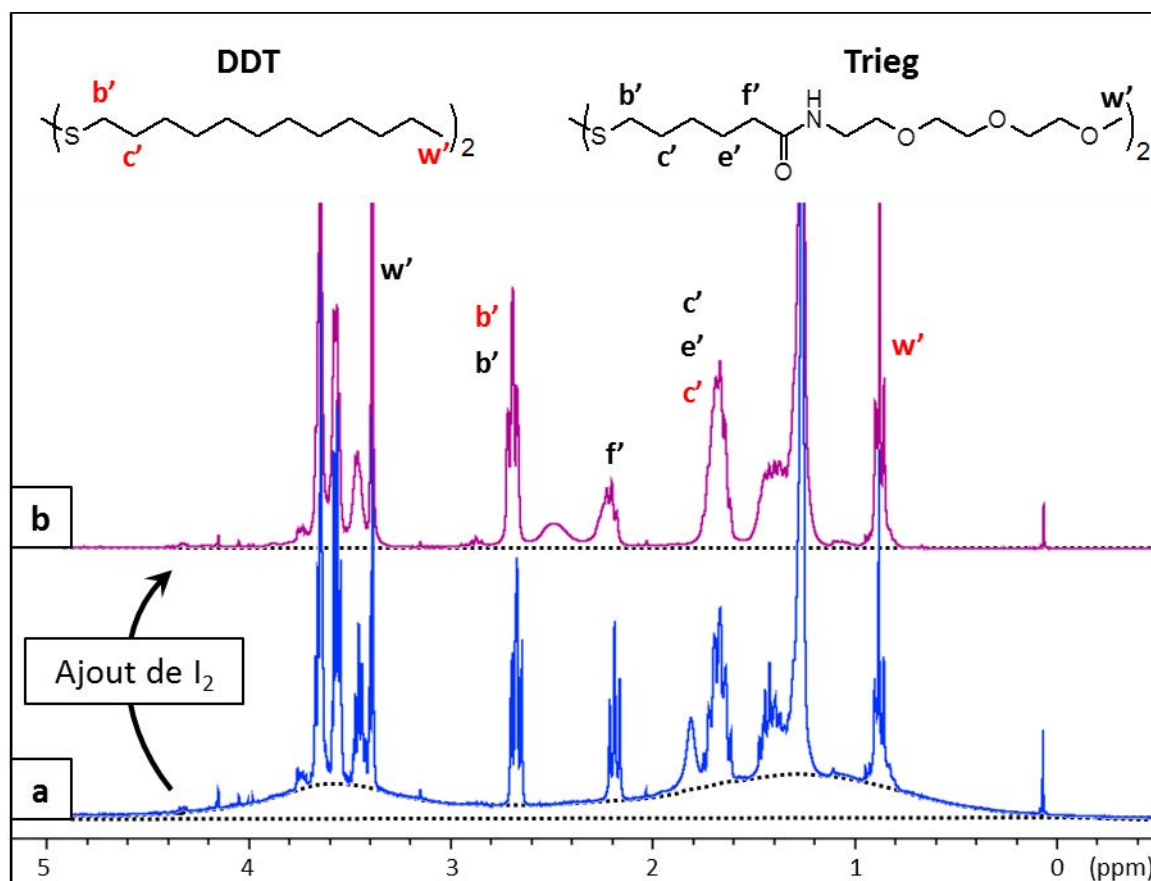
Figure 9. Spectres RMN ^1\text{H} dans \text{CDCl}_3 d'une suspension de nanoparticules en fin d'échange du DDT par le Trieg (a) et de la même suspension après ajout de diiode (b). Le diiode oxyde les thiolates greffés en surface des nanoparticules. Toutes les espèces liées représentées par des signaux très élargis en (a) sont alors libérées en solution, retrouvant ainsi leur mobilité : les pics correspondants s'affinent.
