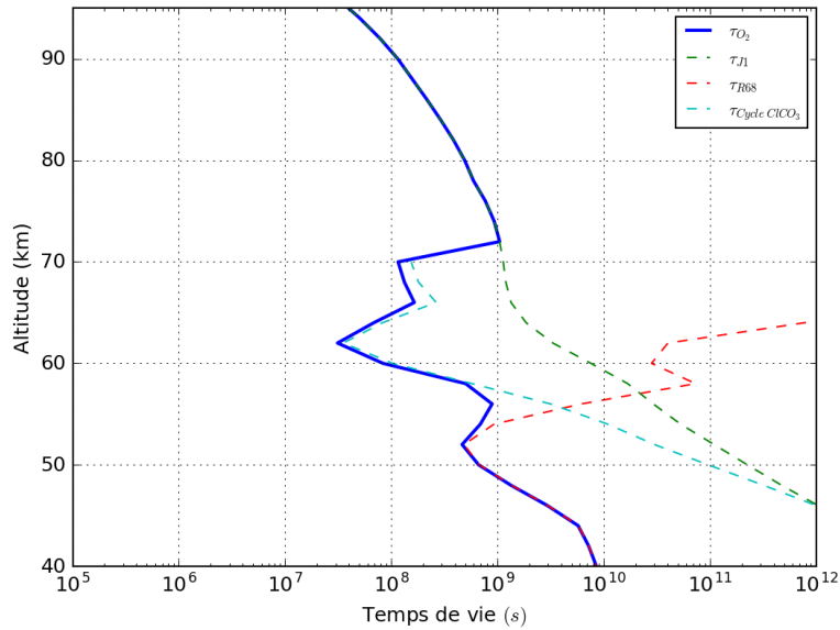
FIGURE 8.19 – Durée de vie de O 2 calculée par notre modèle avec SO 2 initialisé à 10 ppmv dans l'atmosphère profonde et après 100 jours vénusiens simulés. Seules les réactions principales dans la perte de O 2 sont affichées.
