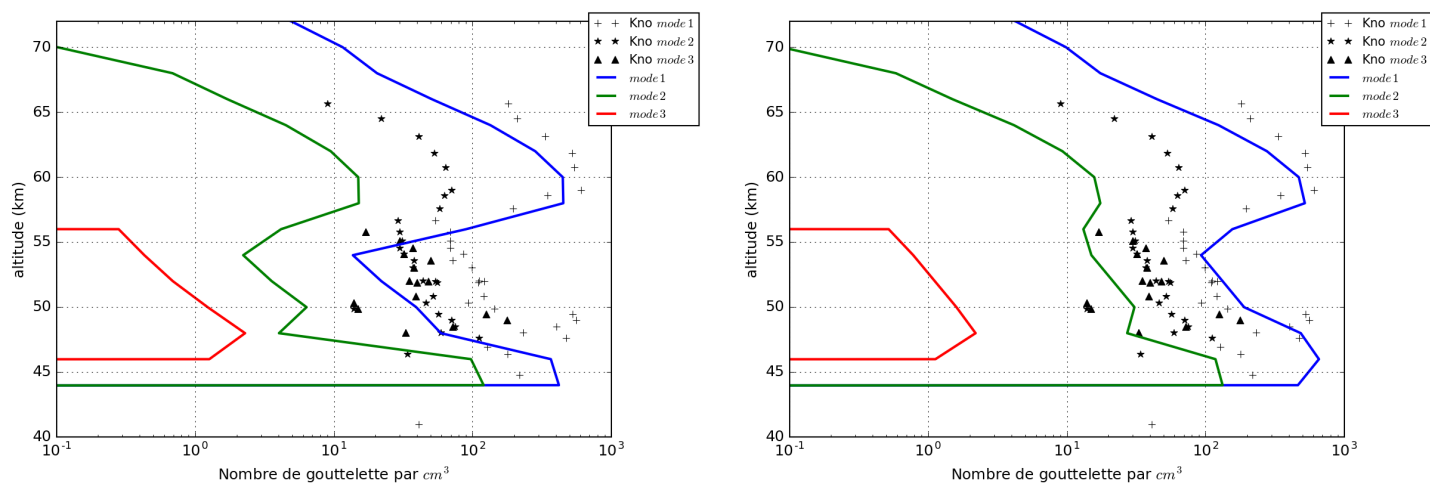
(a) Simulation initialisée avec un mode 3 , constitué de gouttelettes d'acide sulfurique.
