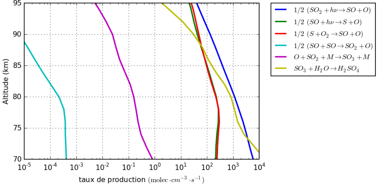
FIGURE 3.3 – Les vitesses de réaction des cycles catalytiques décrits dans Winick and Stewart (1980) sont celles utilisées par les auteurs. Excepté pour la photodissociation de SO 2 , calculé par le code de transfert de rayonnement de notre modèle chimique. Afin de tracer les taux de production, j'ai également utilisé la moyenne globale des concentrations de chaque espèce chimique que nous fournit notre modèle, le GCM 3D de Vénus.
