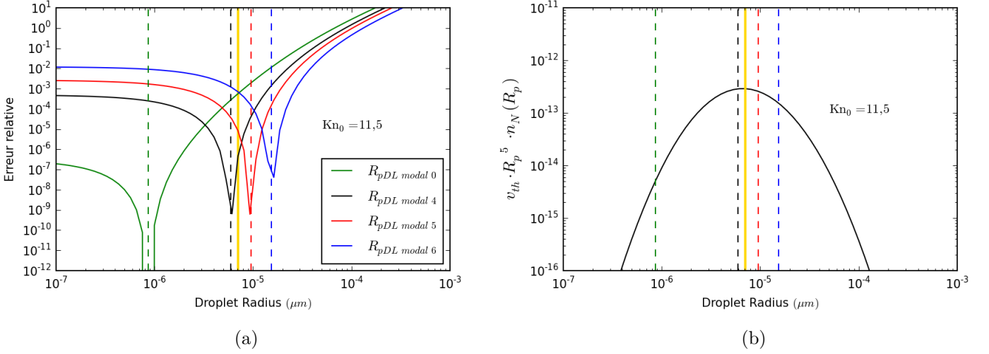
FIGURE B.3 – Détermination de R_{p^*} pour une distribution à Knudsen caractéristique de 11,54. (a) représente l'erreur relative entre le calcul de l'intégrande théorique et celui issu du développement limité en R_{pDL\ mode\ X} . Les traits pleins sont l'erreur relative et les pointillés verticaux marquent la valeur du R_{pDL\ mode\ X} choisie. (b) représente la valeur de l'intégrande selon le rayon. La ligne verticale pleine et dorée représente la valeur du rayon pour lequel l'intégrande est maximale.
