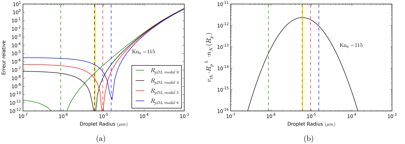
FIGURE B.4 – Détermination de R_{p^*} pour une distribution à Knudsen caractéristique de 115,4. (a) représente l'erreur relative entre le calcul de l'intégrande théorique et celui issu du développement limité en R_{pDL\ mode\ X} . Les traits pleins sont l'erreur relative et les pointillés verticaux marquent la valeur du R_{pDL\ mode\ X} choisie. (b) représente la valeur de l'intégrande selon le rayon. La ligne verticale pleine et dorée représente la valeur du rayon pour lequel l'intégrande est maximale.
