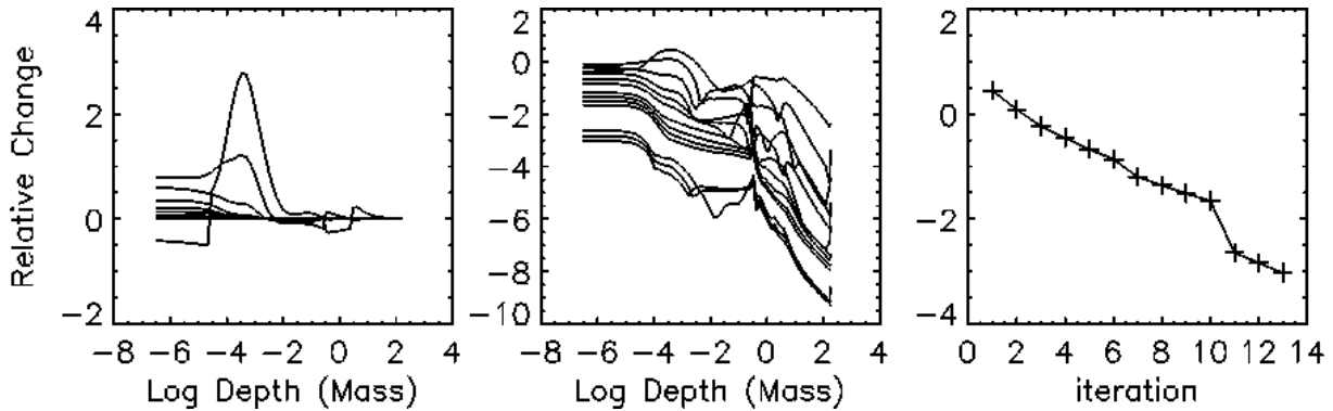
FIG. A.1 : Exemple de test de convergence à partir des variations relatives de tous les paramètres d'état (Eq. 2.21) à chaque point en profondeur calculé : (\Delta k^n \equiv (k^n - k^{(n-1)}) / k^n ; où i est l'indice de l'itération CL et k est le paramètre considéré. Cet exemple correspond à T_{\text{eff}} = 25000 K, \log g = 4.0 , abondance solaire, modèle hors-ETL avec H et He. Gauche : \Delta k^n versus \log(m) pour chaque paramètre. Centre : \log(|\Delta k^n|) versus \log(m) . Droite : Logarithme de la variation relative maximale pour tous les paramètres et profondeurs \log(|\Delta k_{\text{max}}^n|) en fonction de l'itération. Noter que les itérations s'arrêtent quand \log(|\Delta k_{\text{max}}^n|) \leq la valeur limite ( = 10^{-3} dans ce cas). Pour la convergence de ce modèle il a fallu 13 itérations de la méthode CL.
