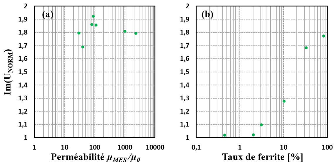
Figure 2.33 : Partie imaginaire de la tension normalisée en fonction de \mu_{MES}/\mu_0 et du taux de ferrite à 0,5 Hz
