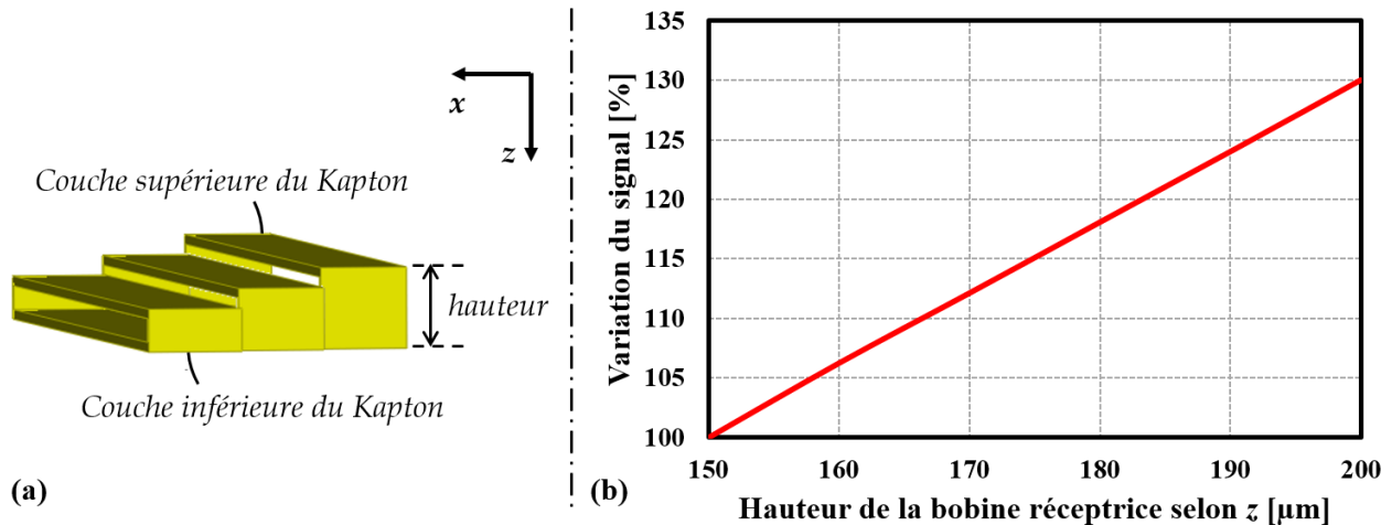
Figure 3.23 : (a) Représentation de l'augmentation de la hauteur d'une bobine réceptrice selon z (vue de profil). (b) Simulations à 1 MHz de la variation de l'amplitude du signal en fonction de la hauteur d'une bobine réceptrice lorsque le défaut est centré sur un élément de réception
