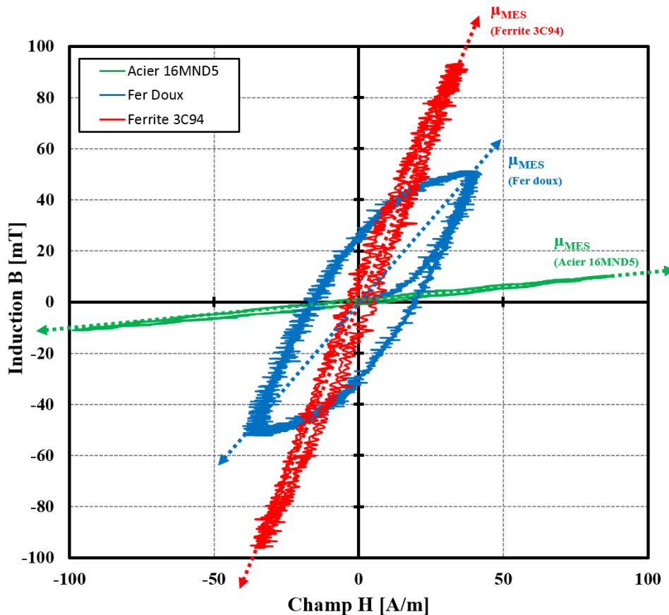
Figure 2.4 : Évaluation expérimentale de \mu_{MES}
