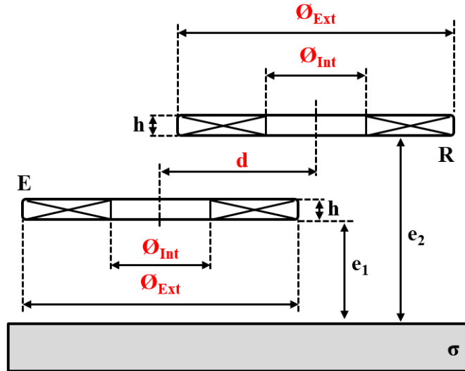
Figure 2.8 : Description des paramètres déterminés (en rouge) du capteur à fonctions séparées
