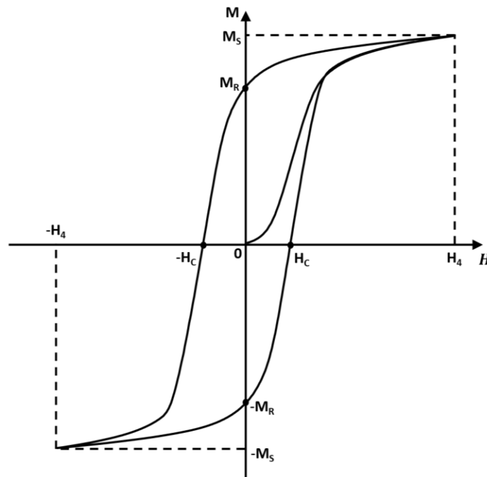
Figure 1.17 : Cycle d'hystérésis
