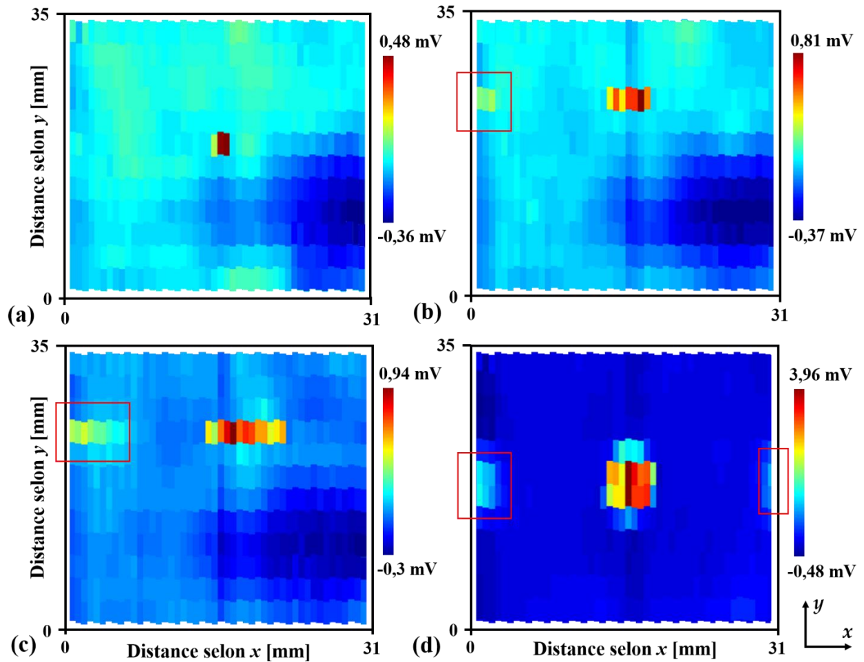
Figure 3.33 : Partie imaginaire du signal à 1 MHz lors de la détection d'entailles ( 2 \times 0,2 \times 0,5 \text{ mm}^3 (a), 5 \times 0,2 \times 0,5 \text{ mm}^3 (b) et 10 \times 0,2 \times 0,5 \text{ mm}^3 (c) et d'un trou traversant de diamètre 6 mm (d) (maquette en aluminium 2024T3)
