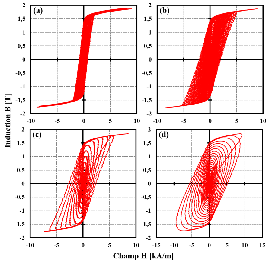
Figure A.1 : Cycles d'hystérésis du fer doux à une fréquence de : 0,05 Hz (a), 0,5 Hz (b), 1 Hz (c) et 5 Hz (d)
