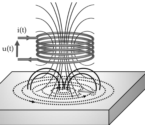
Figure 1.8 : Capteur à double fonction
