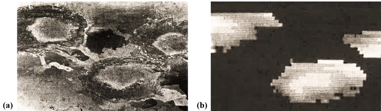
Figure 3.3 : (a) Photographie de l'échantillon d'aluminium corrodé. (b) Cartographie CF obtenue [Macecek_1991]
