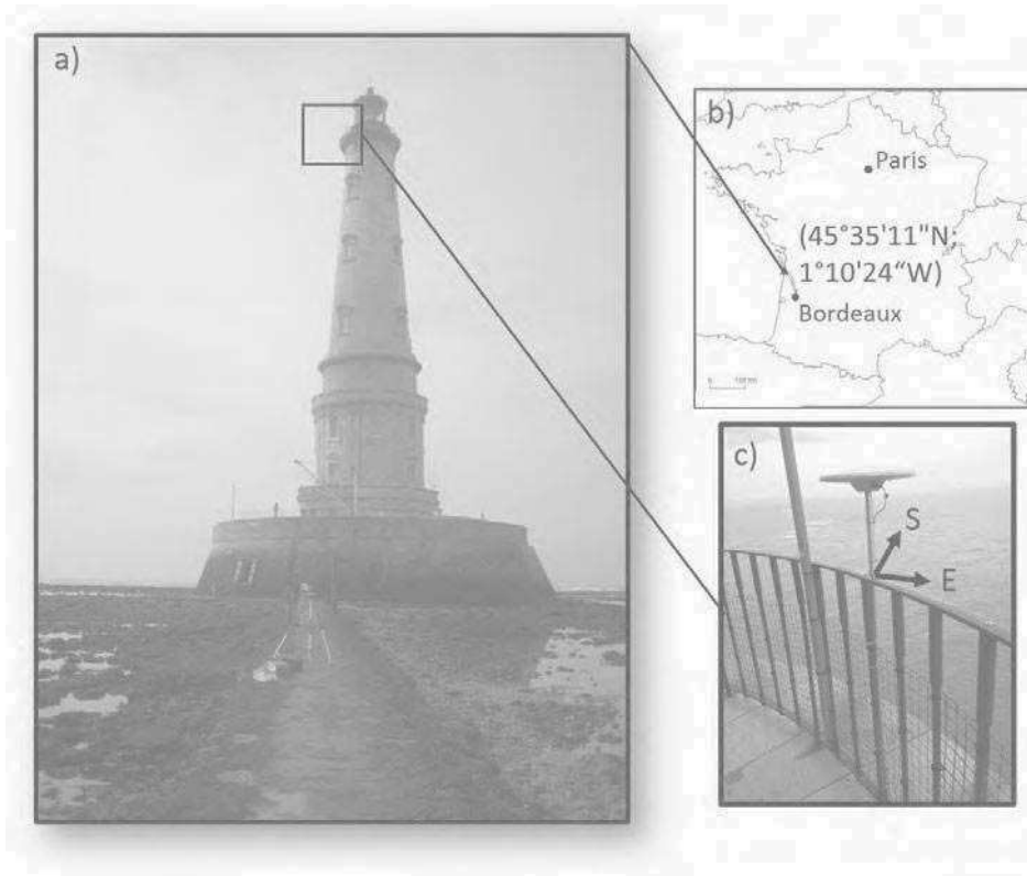
FIGURE 5.5 – Antenne Trimble Zephyr Geodetic 2 et récepteur Trimble NetR9 installés au sommet du phare de Cordouan, à environ 60 m au-dessus du niveau de la mer. Le phare de Cordouan ( 45^{\circ}35'11''\text{N} ; 1^{\circ}10'24''\text{O} ) est situé dans l'embouchure de l'estuaire de la Gironde, dans le Sud-Ouest de la France. Il culmine à \sim 60 m au-dessus du niveau de la mer.
