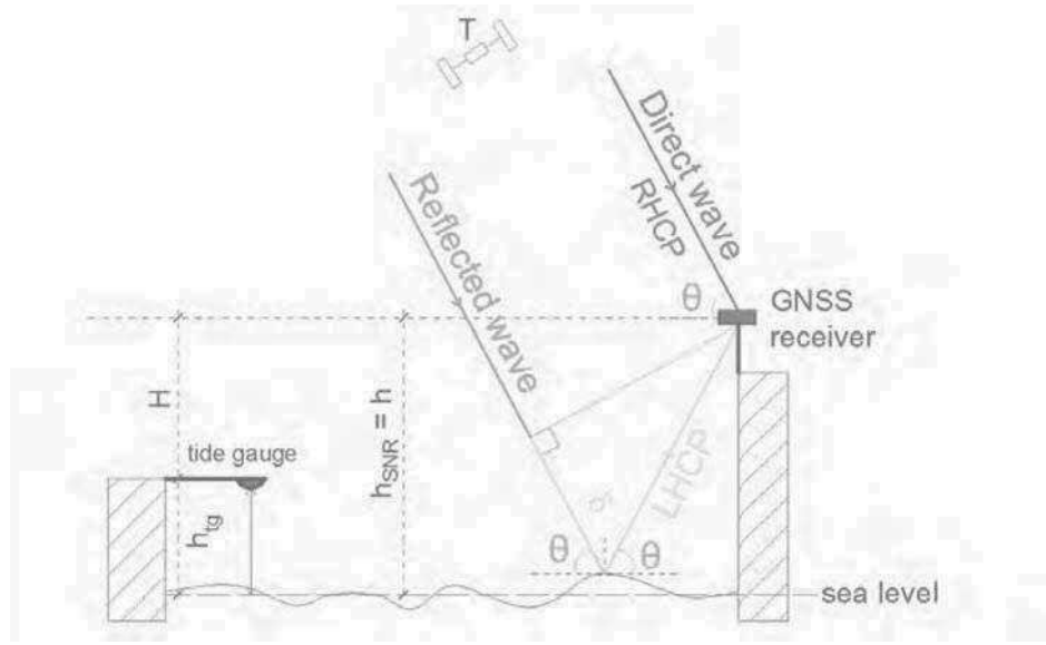
FIGURE 3.13 – Géométrie d'un réflectomètre GNSS à antenne unique.
