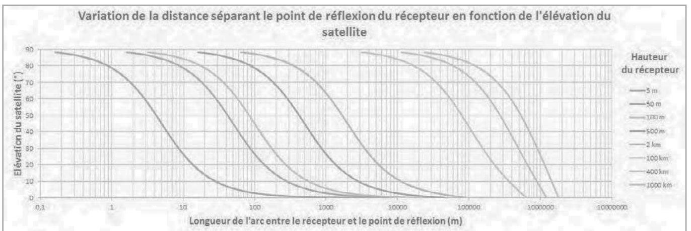
Figure 8. Eloignement des points de réflexion en fonction de l'élevation du satellite, pour différentes hauteurs du récepteur
