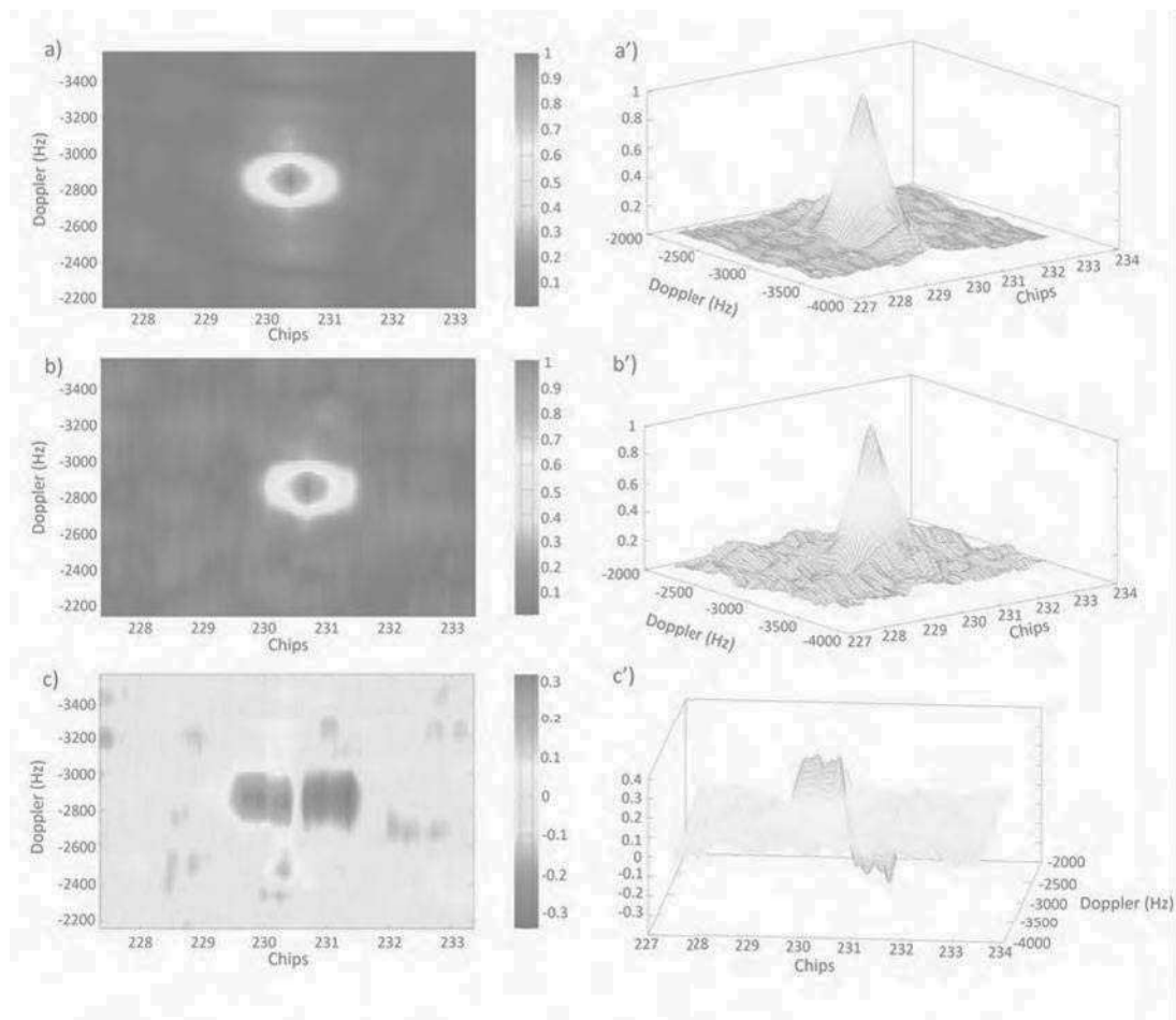
FIGURE 3.5 – Cartes de Délai-Doppler (DDM) obtenues pour un signal direct (a et a') et réfléchi (b et b'), et différence entre les deux (c et c').
