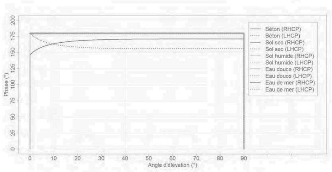
FIGURE 2.11 – Phase des coefficients de Fresnel pour la composante co-polarisée (RHCP) et cross-polarisée (LHCP) d'une onde électromagnétique (RHCP) se réfléchissant sur différents types de surface.
