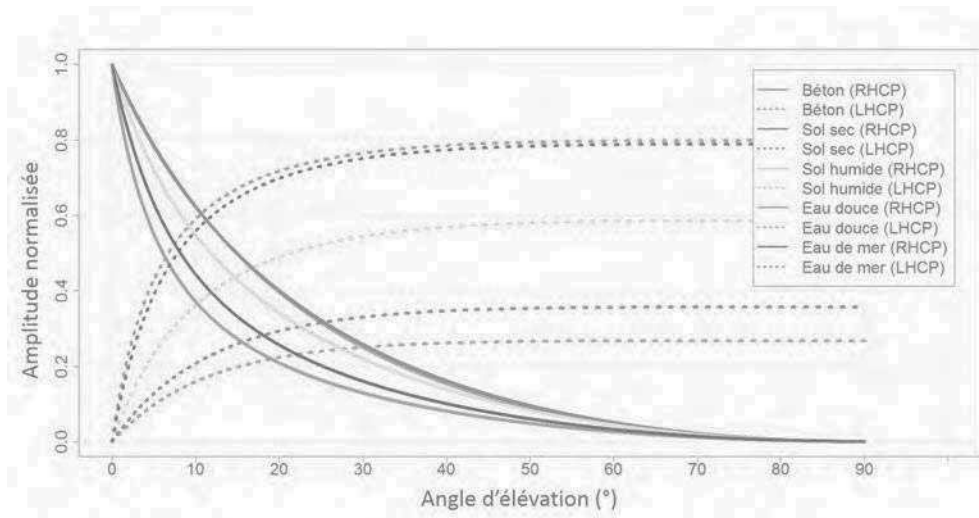
FIGURE 2.10 – Amplitude des coefficients de Fresnel pour la composante co-polarisée (RHCP) et cross-polarisée (LHCP) d'une onde électromagnétique (RHCP) incidente se réfléchissant sur différents types de surface.
