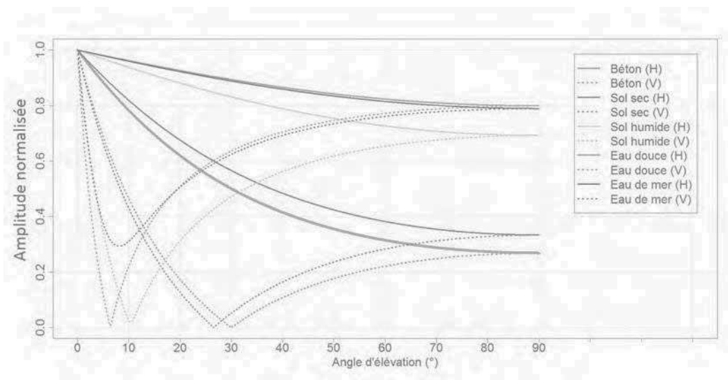
FIGURE 2.8 – Amplitude des coefficients de Fresnel pour la composante horizontale (H) et verticale (V) d'une onde électromagnétique se réfléchissant sur différents types de surface.
