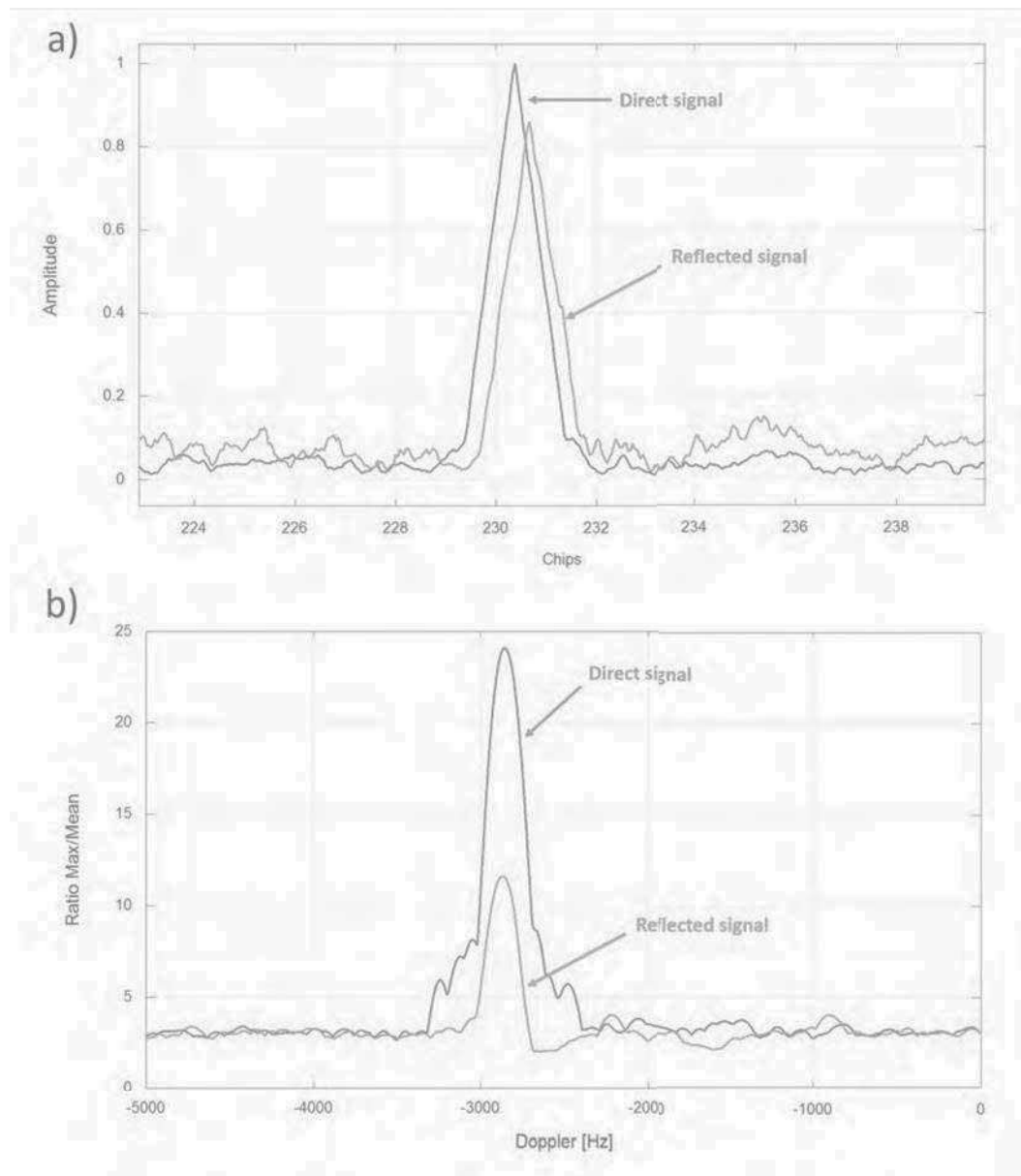
FIGURE 3.3 – Formes d’onde (a) et fréquences Doppler (b) des signaux direct et réfléchi. Les mesures ont été effectuées par une antenne ARINC743A GPS S67-1575 orientée vers le zenith et polarisée RHCP pour capter le signal direct, et une même deuxième antenne orientée vers le nadir et polarisée LCHP pour le signal réfléchi. Les deux antennes étaient placées sur un phare à 60 m au-dessus du niveau de la mer. Les mesures présentées dans cette figure ont été réalisées sur le satellite GPS PRN15, dans la situation d’une mer calme.
