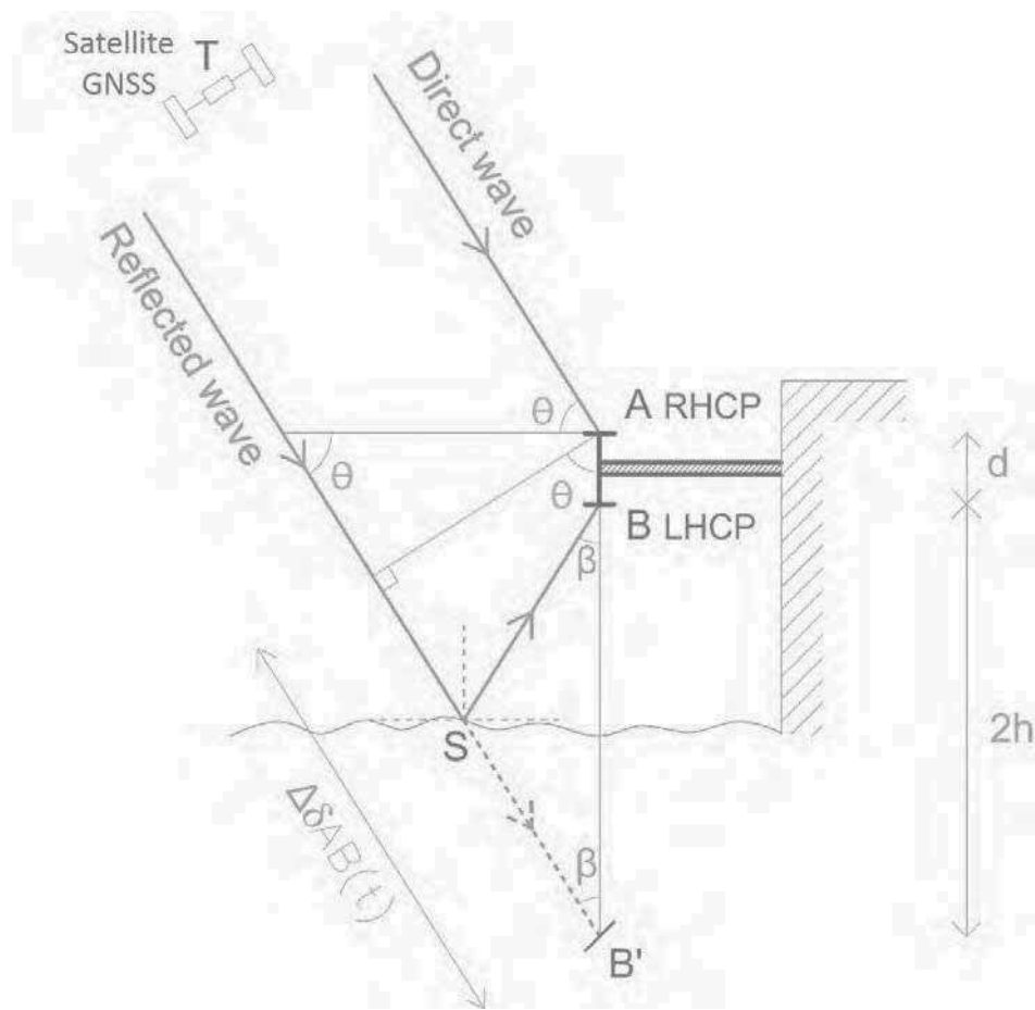
FIGURE 3.1 – Géométrie d'un réflectomètre GNSS à double antenne.
