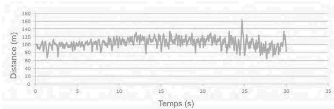
FIGURE 3.9 – Différence de trajet entre les signaux directs et réfléchis pour le satellite PRN12.
