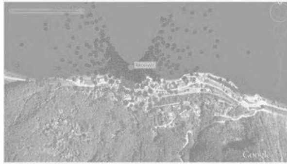
FIGURE 4.8 – Influence du relief - Points de réflexion spéculaires obtenus en intégrant un MNT (rouge) et en approximant la Terre en un ellipsoïde (orange). Par souci de clarté, les altitudes des points oranges (sans prendre en compte le MNT) ont été mises égales à celles du MNT pour qu'ils soient visibles. Les simulations ont été réalisées avec un récepteur placé à 50 m du sol, au bord du lac de Genève (46°24'30"N ; 6°43'06"E).
