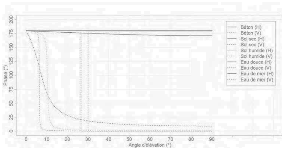
FIGURE 2.9 – Phase des coefficients de Fresnel pour la composante horizontale (H) et verticale (V) d'une onde électromagnétique se réfléchissant sur différents types de surface.
