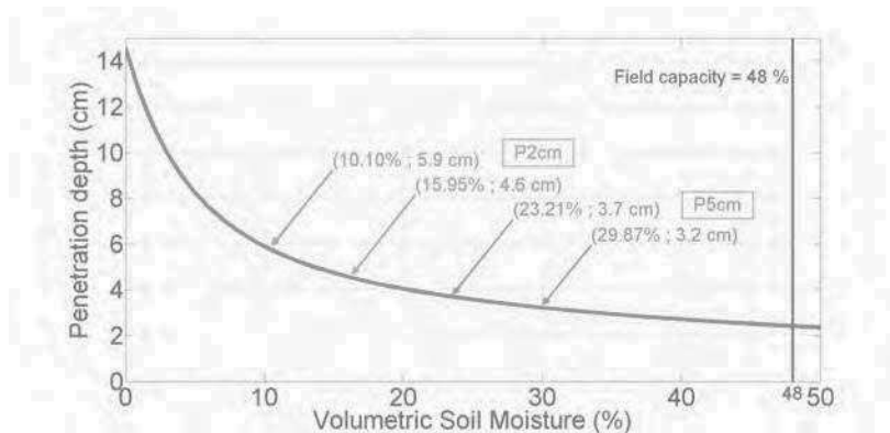
FIGURE 6.4 – Profondeur de pénétration théorique des ondes GNSS dans le sol autour de l'antenne géodésique.
