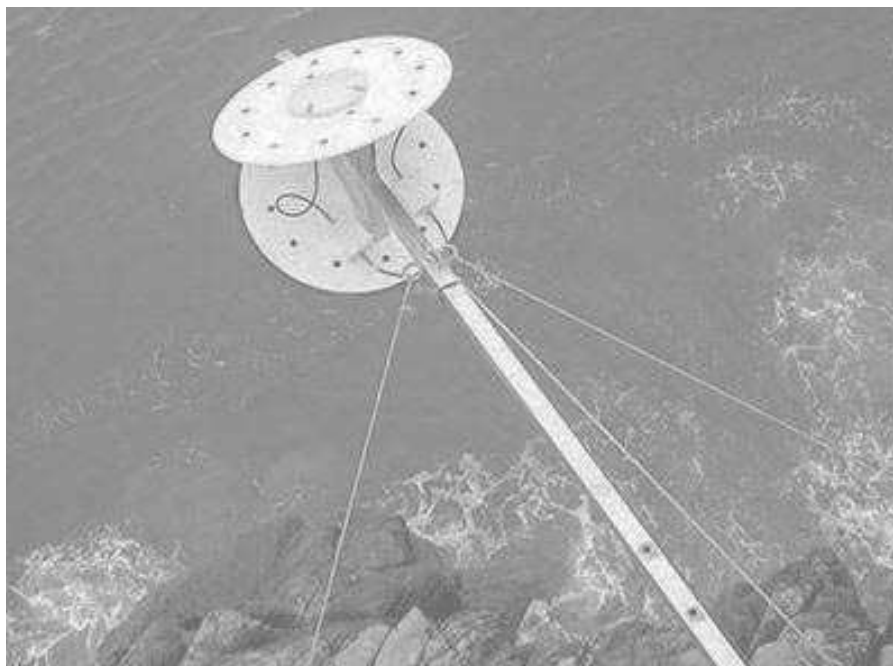
Figure 2. Réflectomètre Oceanpal de Starlab
