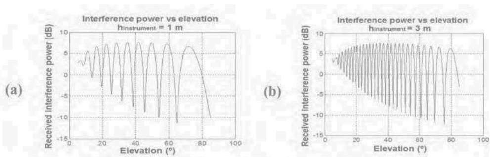
FIGURE 3.12 – Puissance théorique reçue par un réflectomètre de type IPT pour une réflexion sur la mer, en fonction de l’angle d’élévation du satellite pour une hauteur d’instrument de 1 m (a) et 3 m (b).
