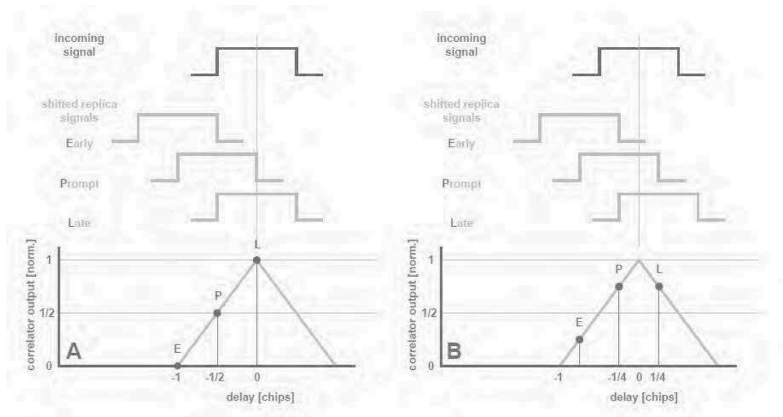
FIGURE 3.2 – Décomposition de la fonction de corrélation du signal direct. Source : Helm (2008) (adapté)
