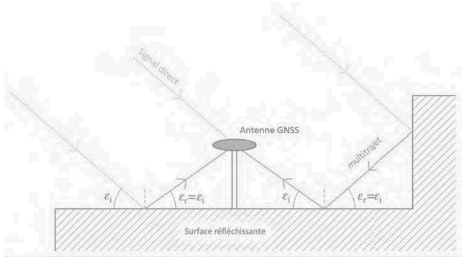
FIGURE 2.1 – Le phénomène de multi-trajet sur les signaux GNSS. \epsilon_i : angle d'incidence. \epsilon_r : angle de réflexion.
