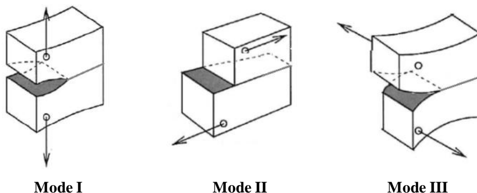
Figure I. 9 : Différents modes de rupture
