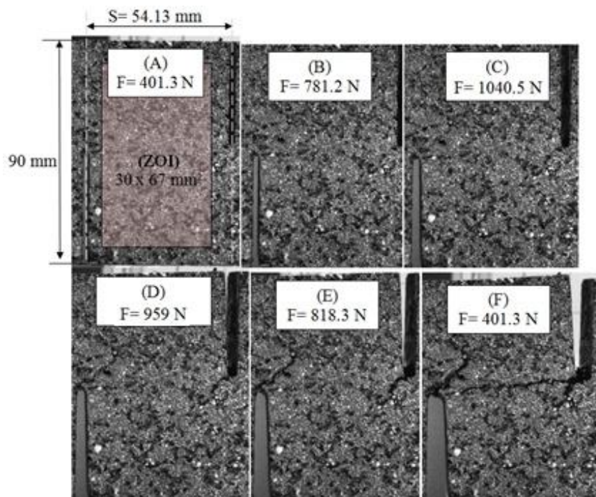
Figure II. 41: Fissurations macroscopiques au voisinage de l'interface.
