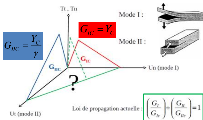
Figure III. 2 : Description des paramètres physiques liés à l'amorçage et à la propagation (Vandellos, 2009)
