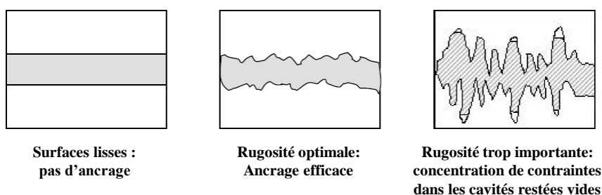
Figure I.6 : Effet de la rugosité et du mouillage sur l'ancrage mécanique (Monternot et al., 1978)
