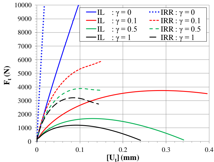
Figure III. 37 : Effet du paramètre de couplage avec Y_c = 30 \text{ J/m}^2
