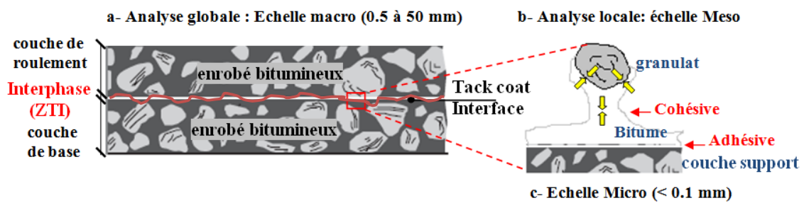
Figure I. 25 : Représentation multi-échelle de la Zone de Transition Interfaciale (ZTI)
