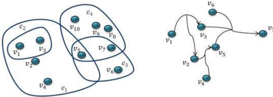
FIGURE 3.6 : Exemples d'hypergraphe.
