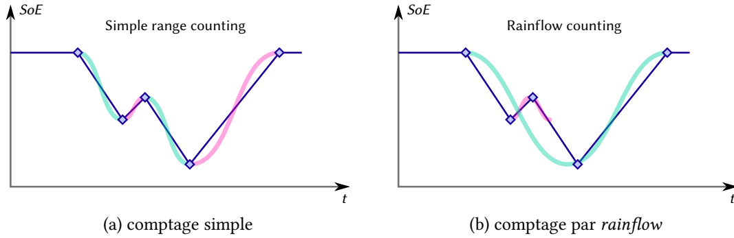
FIGURE 2.16 – Comparaison entre une détection des cycles par extrema locaux et une détection par rainflow [94, 188]
