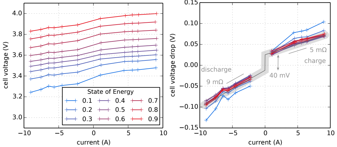
FIGURE 2.14 – Tension aux bornes d’une cellule Lithium Ion NCA, en fonction du courant échangé et pour différentes valeurs de l’état d’énergie. À droite, la chute de tension en est déduite afin de déterminer sa dépendance par rapport au courant [94].
