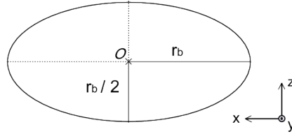
Figure 2.3 – Condensat au fond du piège habillé. L'ellipse représente schématiquement une coupe dans le plan vertical de la surface équipotentielle sur laquelle est contraint le nuage. Elle présente un petit axe de demi-longueur r_b/2 selon la direction z et un axe dans le plan horizontal de longueur r_b . Les atomes condensés, en présence de la gravité, se réunissent au fond de la bulle, à une altitude d'environ z = -r_b/2 .
