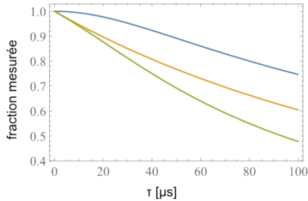
Figure A.5 — Évolution simulée de la fraction d’atomes détectée (rapport entre le nombre d’atomes détectés et le nombre d’atomes réellement présents) en fonction de la durée d’une impulsion sonde d’intensité 9I_{sat} non polarisée. En bleu-haut seulement l’effet Doppler est pris en compte. En jaune-milieu seulement le dépompage est pris en compte. En vert-bas les deux effets sont combinés.
