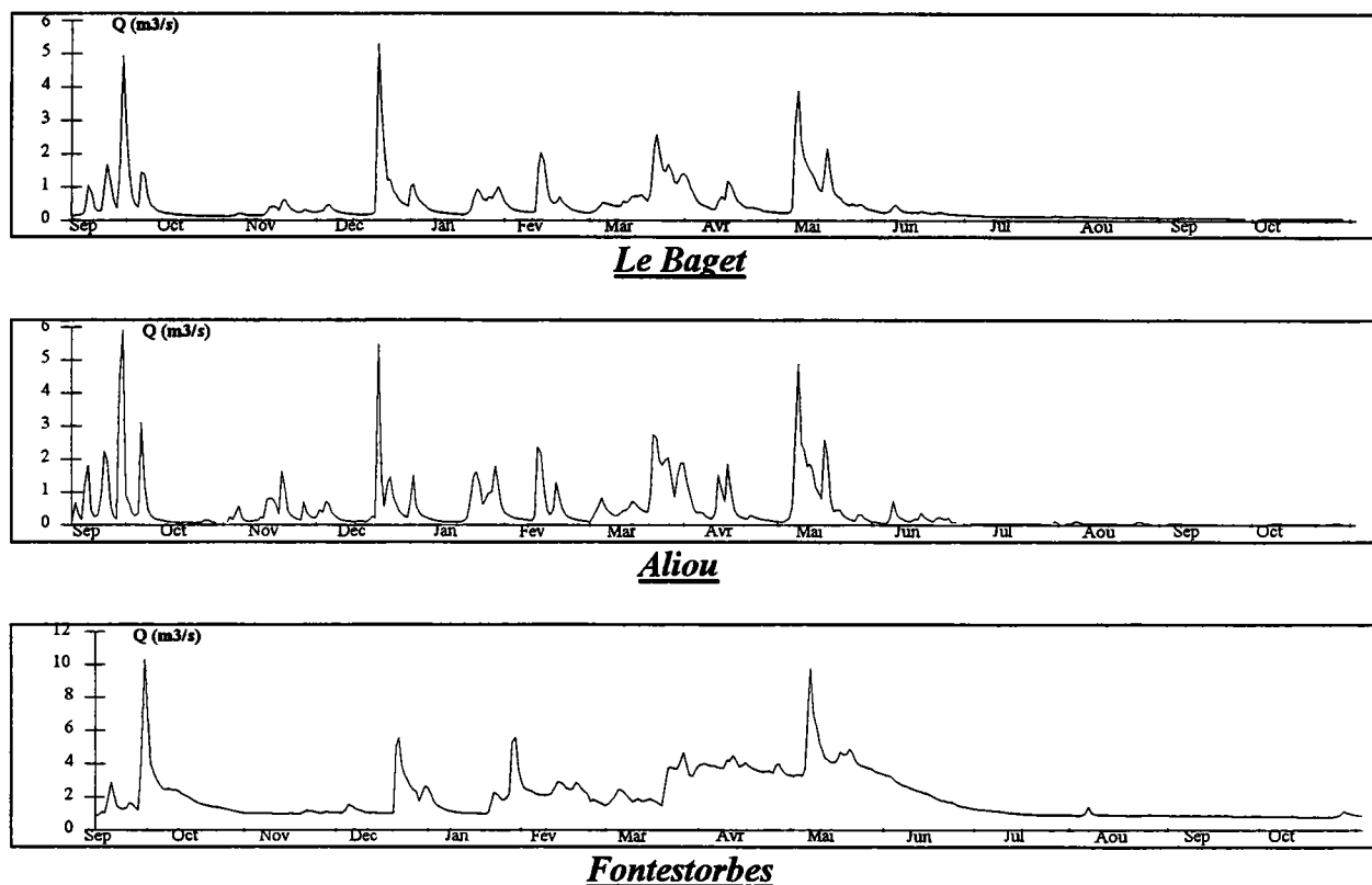
Graphique 3 - 46. Hydrogrammes des aquifères karstiques du Baget, d'Aliou et de Fontestorbes, cycle 1985
