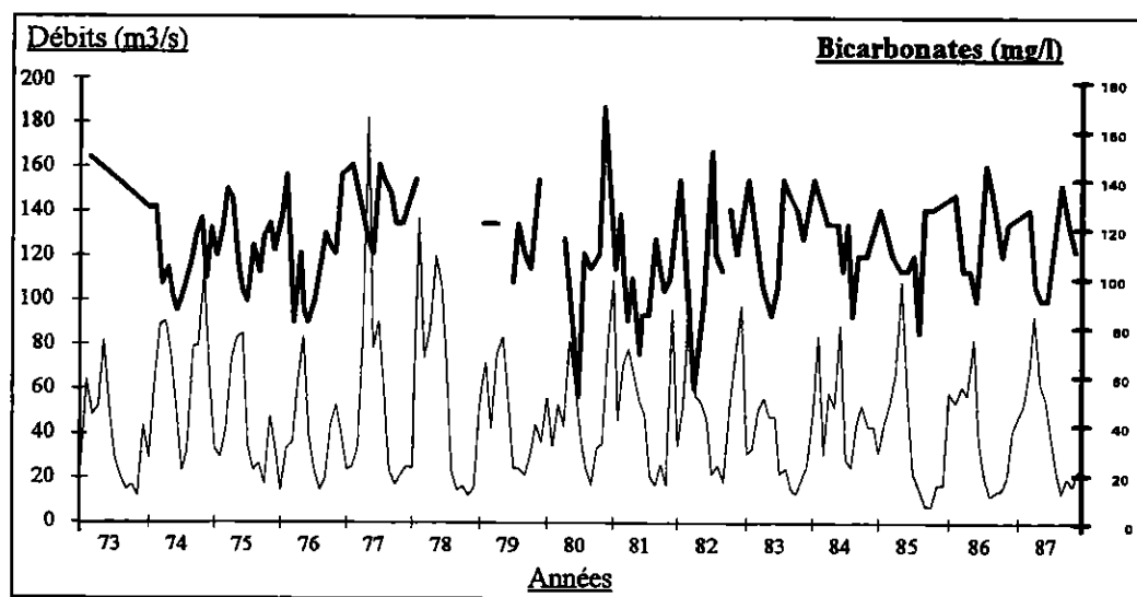
Graphique 4 - 59. Evolution des teneurs en bicarbonates et des débits à la station de Roquefort/Garonne sur le Salat, période 1973 à 1987
