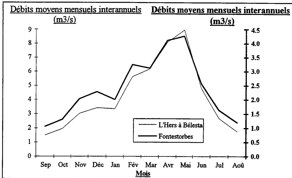
Graphique 3 - 14. Courbes des débits moyens mensuels interannuels de l'Hers à Bélesta et de Fontestorbes, cycles 1973 à 1979
