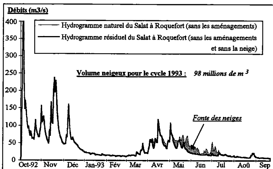
Graphique 3 - 76. Hydrogramme résiduel du Salat (sans les aménagements et sans la neige), cycle 1993
