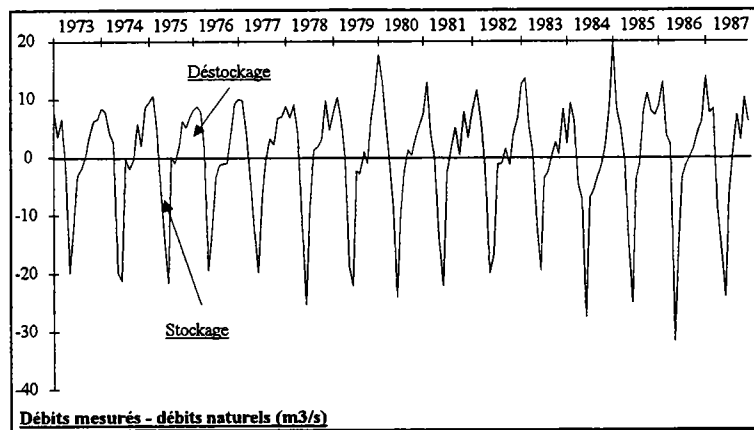
Graphique 3 - 63. Mise en évidence des stockages et déstockages des barrages à vocation énergétique à Auterive (Ariège), période 1973-1987
