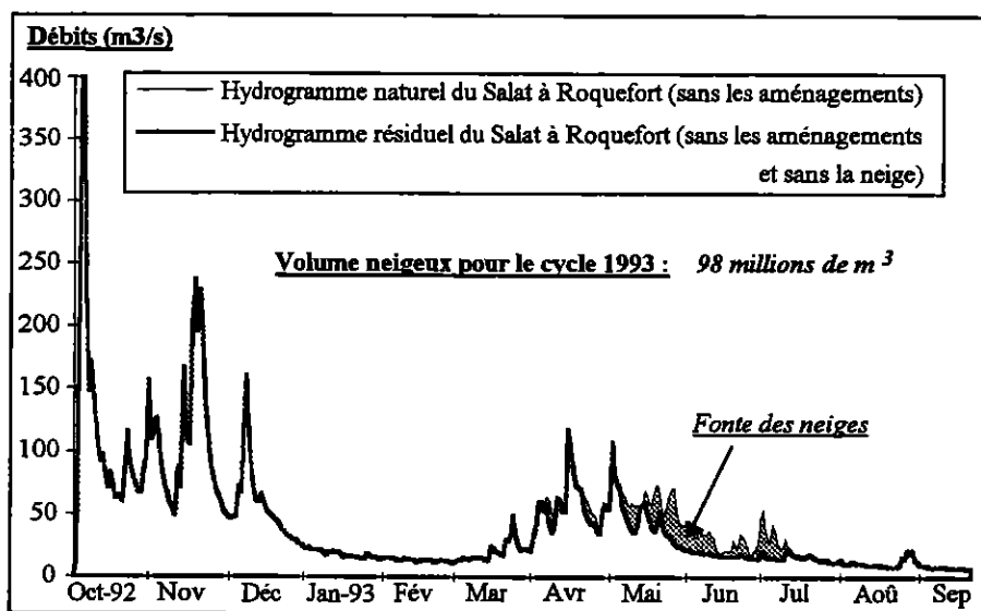
Graphique 3 - 76. Hydrogramme résiduel du Salat (sans les aménagements et sans la neige), cycle 1993
