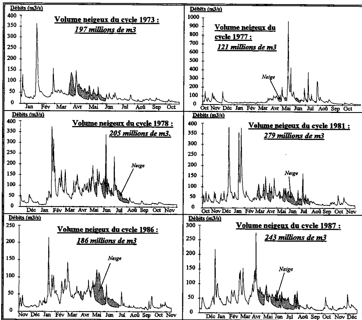
Graphique 3 - 67. Volumes d'écoulement neigeux et hydrogrammes du Salat à Roquefort, sans l'influence neigeuse, pour les cycles 73, 77, 78, 81, 86, et 87
