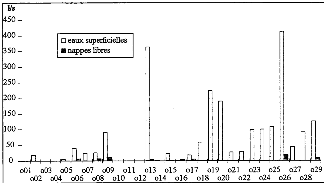
Graphique 14. Répartition des débits prélevés pour l'irrigation par sous-secteurs en 1991 (prélèvements totaux = 2.2 m 3 /s)
