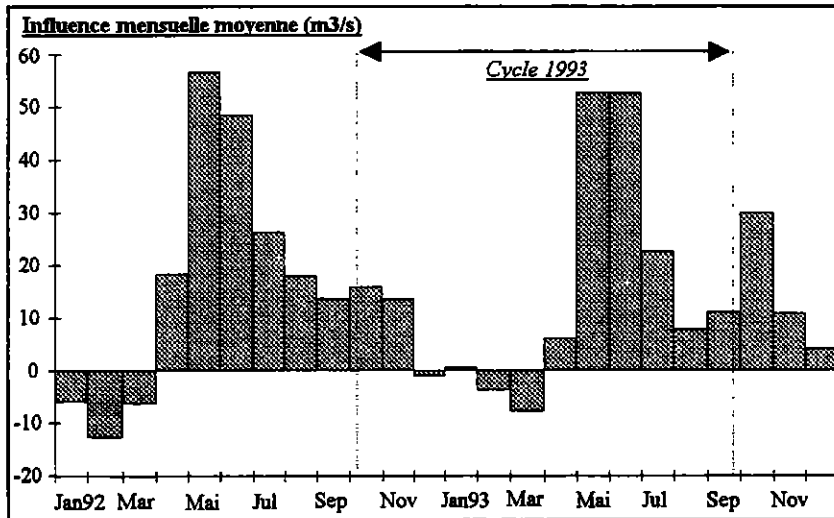
Graphique 3 - 78. Influence mensuelle des aménagements (m 3 /s) sur la Garonne à Portet, cycle 1993
