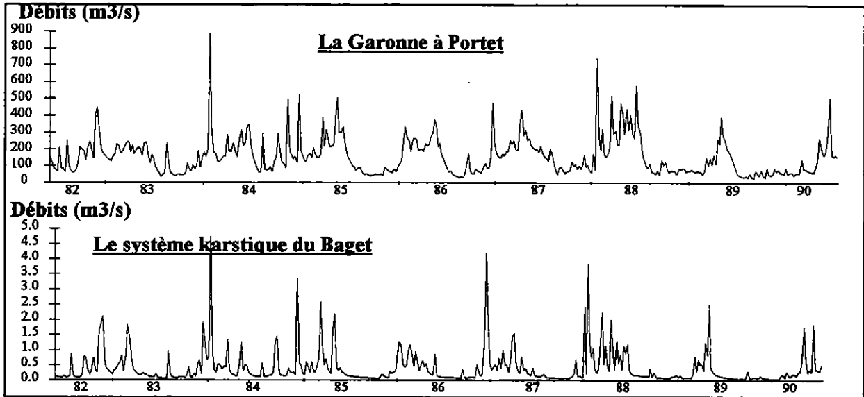
Graphique 3 - 71. Débit de la Garonne et du système karstique du Baget pour la période 1982-1990
