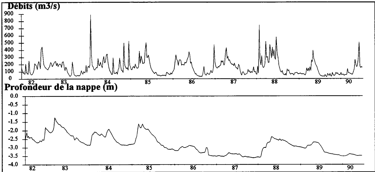
Graphique 3 - 69. Débit de la Garonne (en haut) et piézométrie à Saint-Porquier (en bas) pour la période 1982-1990
