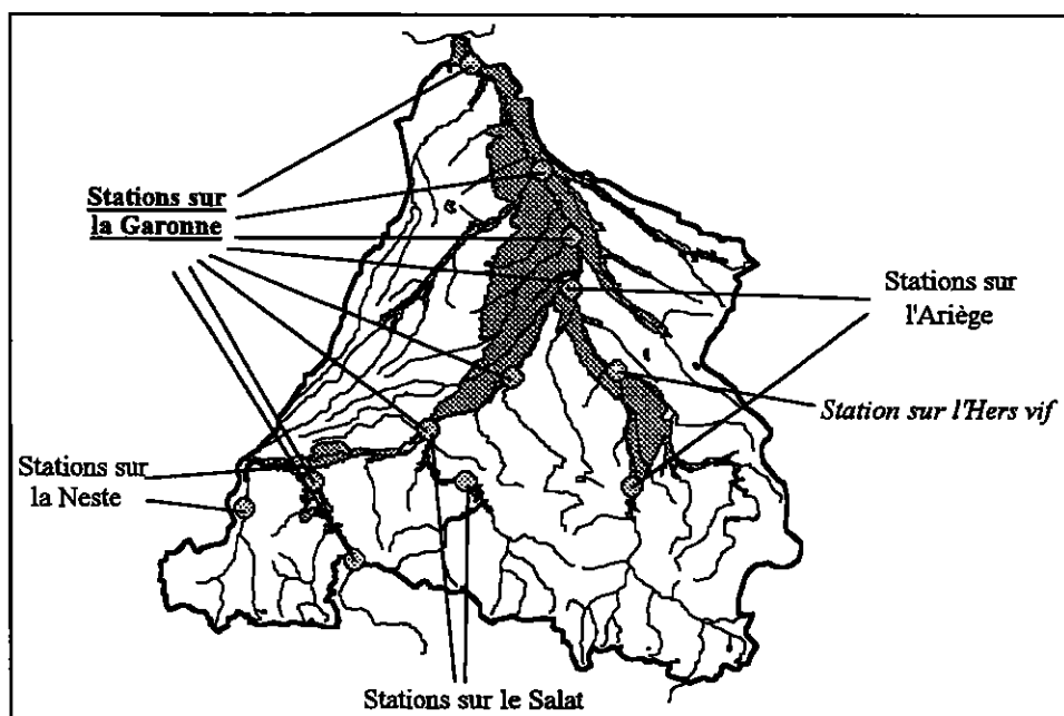
Carte 5 - 1. Stations de prélèvements isotopiques de la campagne d'été du cycle 1993
