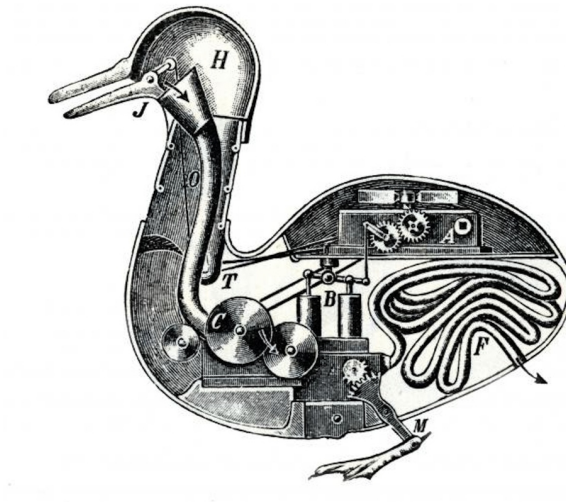
FIGURE 1.2 – Croquis du canard créé par Jacques de Vaucanson en 1738.
