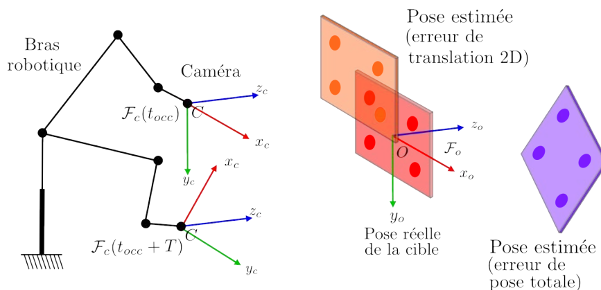
FIGURE 2.8 – Les deux positions de la caméra au début et à la fin de son mouvement, à t = t_{occ} et à t = t_{occ} + T sont représentées. La pose réelle de la cible est représentée en rouge. L'erreur de pose de translation 2D est représentée en orange (Sect. 2.4.1). L'erreur de pose complète est représentée en violet (Sect. 2.4.2).
