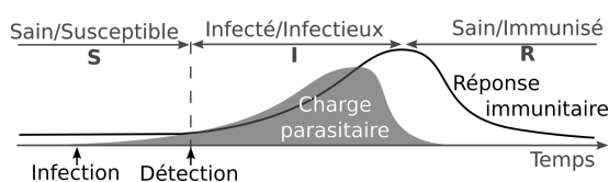
Figure 3.3: Dynamique de la charge parasitaire (surface grisée) et de la réponse immunitaire (courbe noire) chez un individu, avec les phases Sain (et Susceptible d'être infecté), Infecté et Immunité (qui peut redevenir Susceptible après la perte de "mémoire" immunitaire). Adapté de Keeling et Rohani, (2008).
