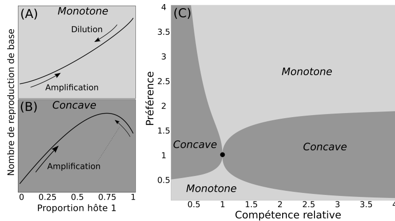
Figure 6.3: Modélisation du \mathcal{R}_0 en fonction des préférences et compétences relatives ( transmission ratio ) pour les maladies vectorielles (adapté de Miller et Huppert, (2013)). (A) Fonction monotone et (B) fonction concave hump-shaped . (C) Forme du \mathcal{R}_0 : monotone en claire et concave en foncée, le point noir (1, 1) est une fonction de \mathcal{R}_0 constante en fonction de la proportion des hôtes.
