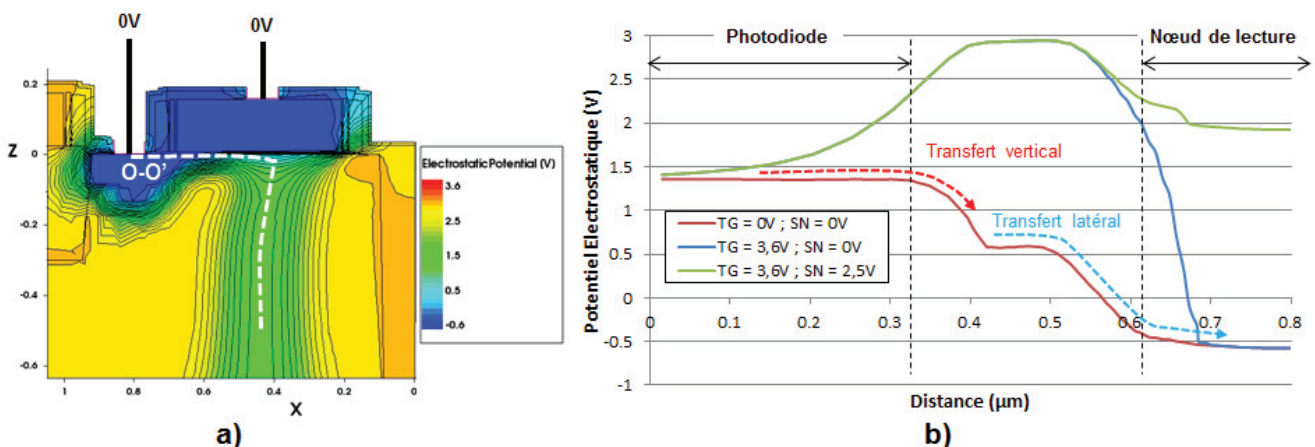
Figure 48 : a) Coupe 2D d'une simulation TCAD en trois dimensions du potentiel électrostatique régnant dans la partie supérieure de la photodiode lors du transfert. La figure b) représente le profil de potentiel électrostatique selon la courbe O-O' lors du transfert des charges (rouge), après remise à zéro de la photodiode (bleu) et une fois la ligne bloquée au début de l'intégration (vert). La direction de transfert des charges est indiquée par les flèches rouges et bleues.
