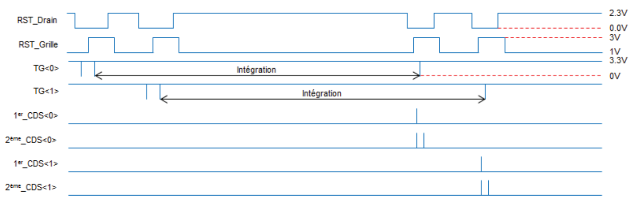
Figure 55: Timing et tensions de mise en œuvre de l'architecture partagée à 2-transistors sur un pixel de type P.
