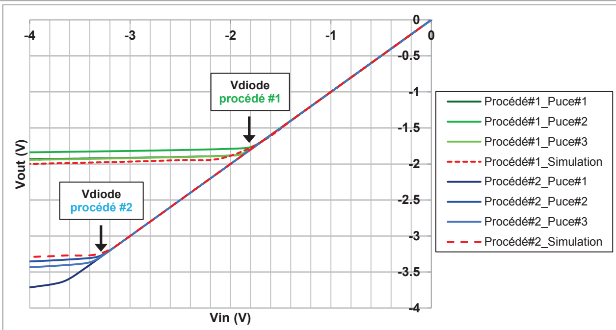
Figure 41 : Mesures de potentiel de diode sur la structure présentée en figure 40 et fabriquée avec deux procédés de fabrication différents : un dopage d'épitaxie faible (vert) et un autre élevé (bleu). Les courbes ont été obtenues en mesurant trois puces par plaque de silicium. La différence de V_{diode} entre chaque puce provient de la variabilité naturelle du procédé de fabrication. Les deux procédés ont été simulés avec les mêmes paramètres de calibration et les structures virtuellement testées pour donner les courbes en pointillés rouges.
