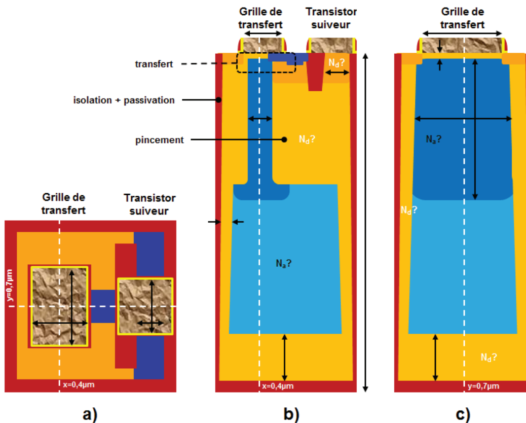
Figure 29 : Schéma présentant les principaux paramètres à optimiser pendant la fabrication du pixel de type P. a) vue du dessus et b) et c) vue en coupe selon y = 0,7\mu\text{m} et x = 0,4\mu\text{m} . Sont notamment à définir les différentes concentrations de dopants des caissons N et P ( N_d et N_a ), le type d'isolation inter pixels, la passivation des interfaces Si/SiO 2 , la profondeur de la photodiode et enfin la zone de transfert des charges de la photodiode vers le nœud de lecture.
