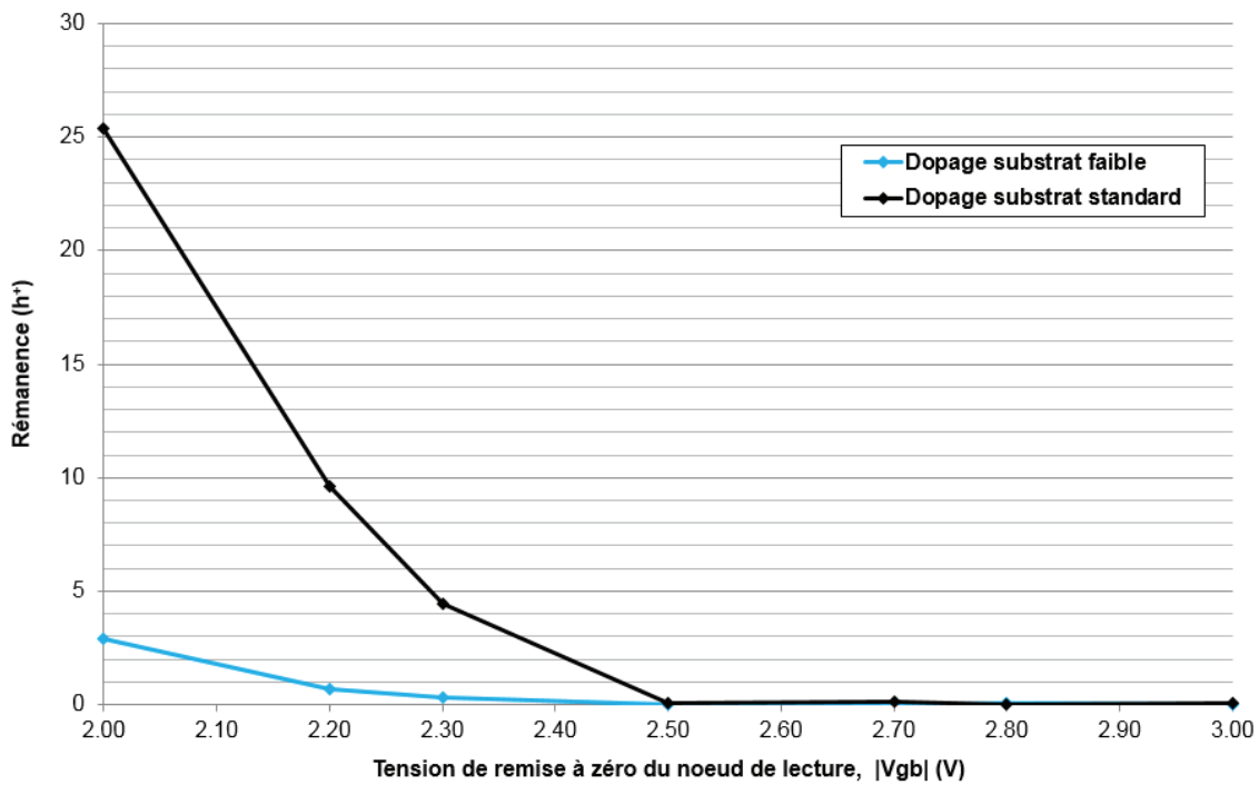
Figure 98 : Mesure de la rémanence moyenne, pour un niveau de signal sous éclairnement d'environ 300 h + , en fonction de la tension de réinitialisation du nœud de lecture pour deux capteurs de type P possédant un dopage substrat différent : dopage standard (noir) et dopage faible (bleu)
