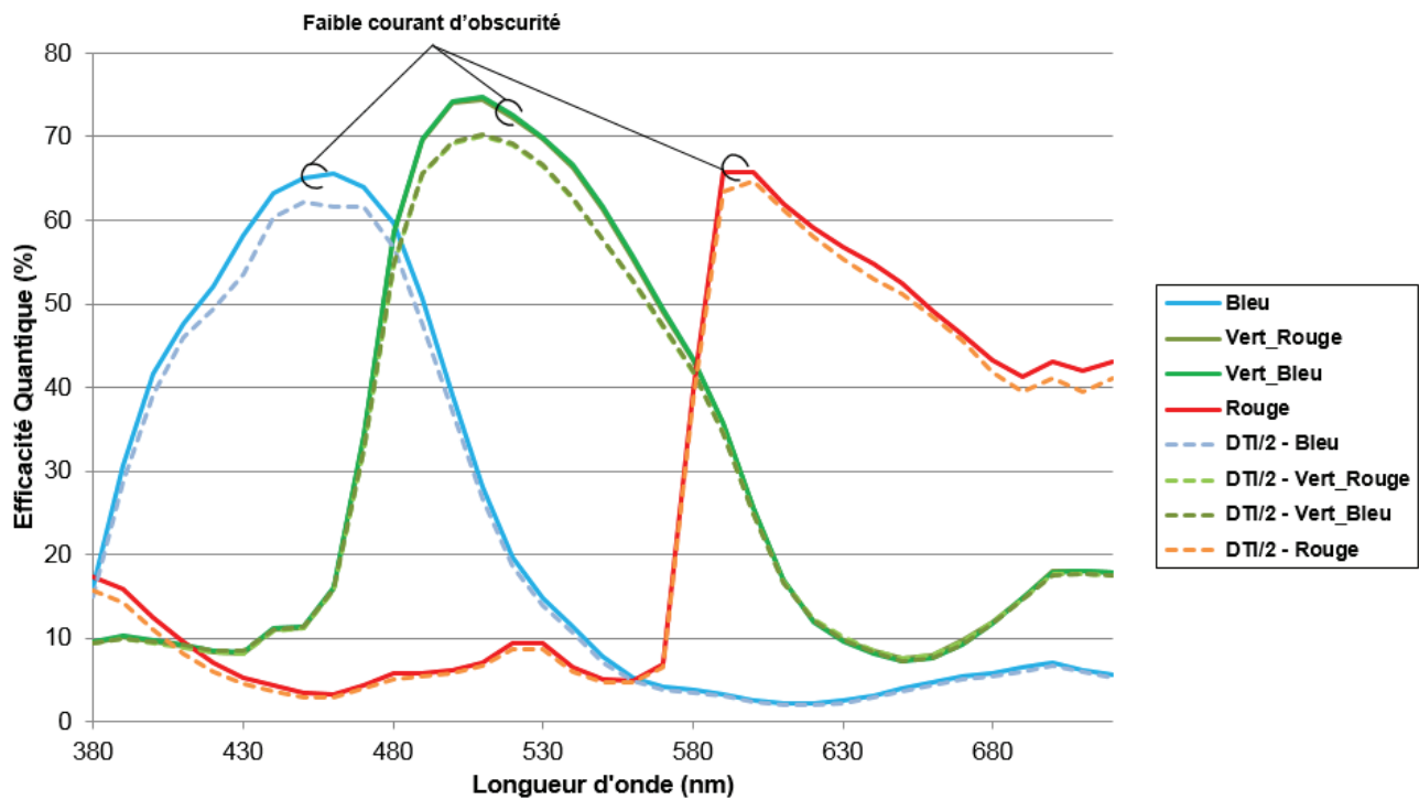
Figure 104 : Comparaison de l'efficacité quantique mesurée sur les trois plans couleur entre 380nm et 720nm pour deux capteurs de type P différents : l'un ayant subi une dose d'implantation standard pour passer l'interface des DTI (trait plein) et l'autre ayant subi une dose divisée par deux (trait pointillé).
