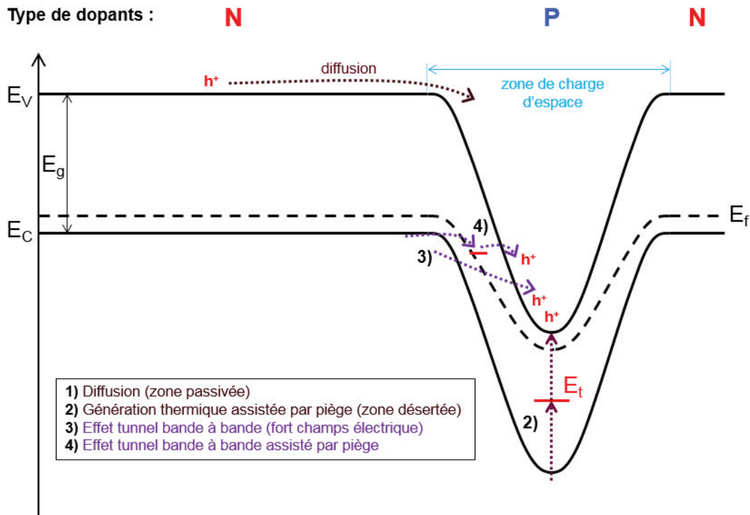
Figure 62 : Diagramme de bandes présentant les principaux mécanismes de génération du courant d'obscurité dans une photodiode pincée de type P : la diffusion (1), la génération thermique (2) et l'effet tunnel bande à bande et celui assisté par piège (3 et 4).
