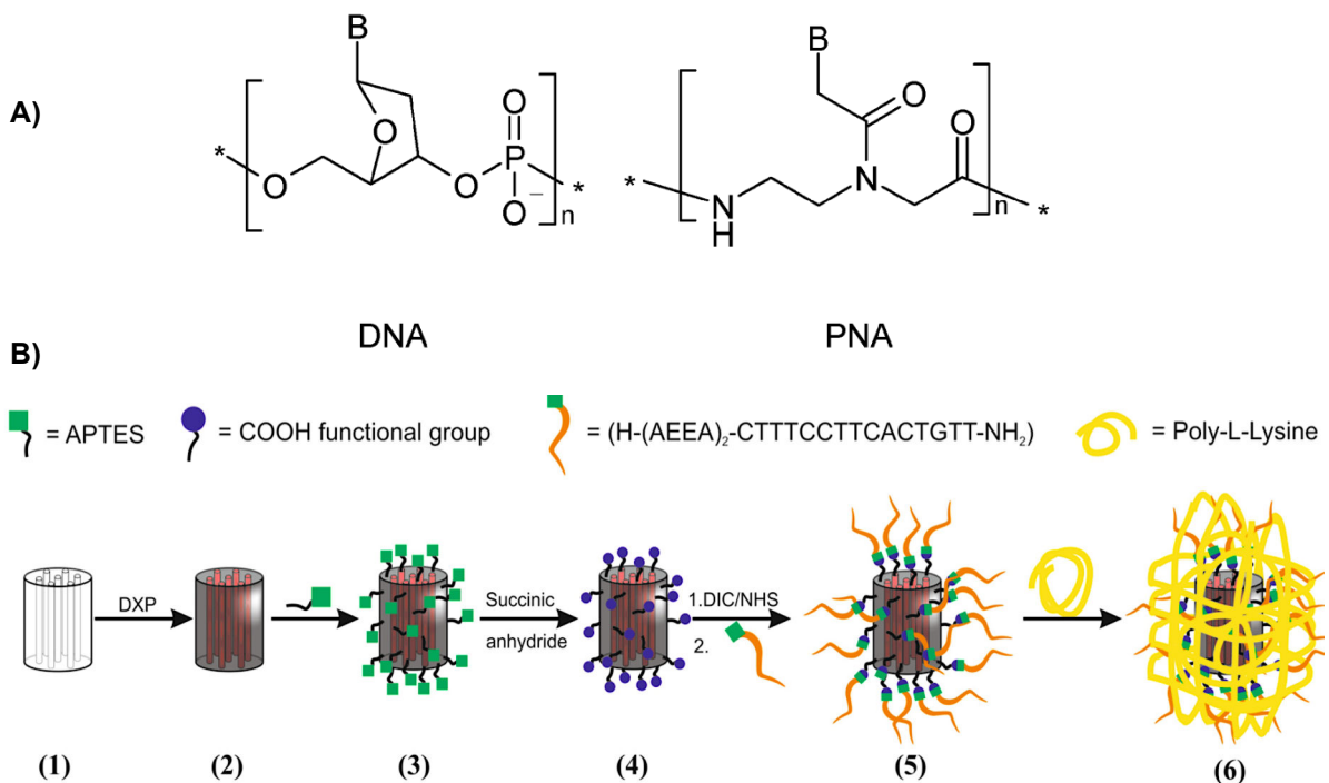
Fig. 3 A) Comparaison entre les structures de l'ANP et de l'ADN; b) Plan représentant les étapes de fonctionnalisation pour obtenir le matériaux zéolite final rempli de molécule fluorescente, modifié par de l'APN sur la surface et couvert avec une fine couche de poly-L-lysine.
