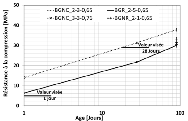
Figure 48 : Evolution des résistances des bétons non adjuvés
