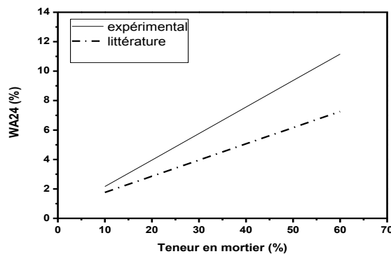
Figure 17 : Influence de la teneur en mortier sur le coefficient d'absorption (Mefteh et al., 2013) ; (Meftah and Arabi, 2011)
