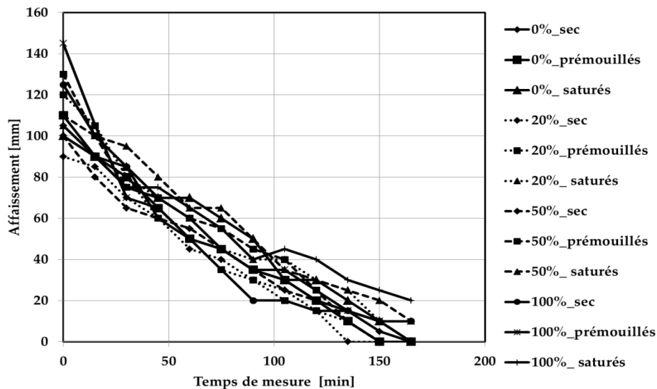
Figure 21 : L'influence du taux de substitution des granulats recyclés à l'état séché à l'air, séché à l'étuve et saturé surfaces sèches sur la maniabilité (Poon et al., 2004)
