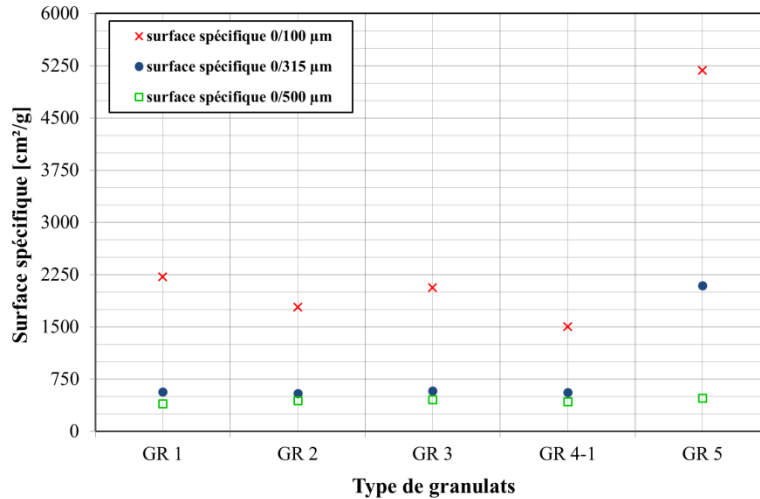
Figure 40 Surfaces spécifiques Blaine des éléments fins
