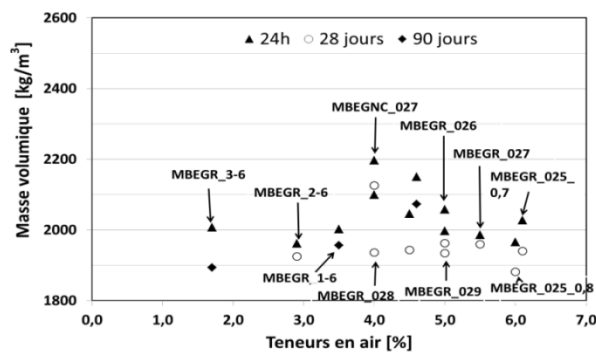
Figure 164 : Evolution de la masse volumique aux différentes échéances avec la teneur en air
