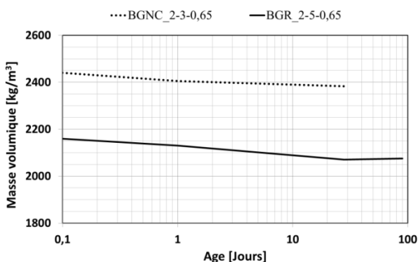
Figure 45 : Evolution de la masse volumique des bétons non adjuvés
