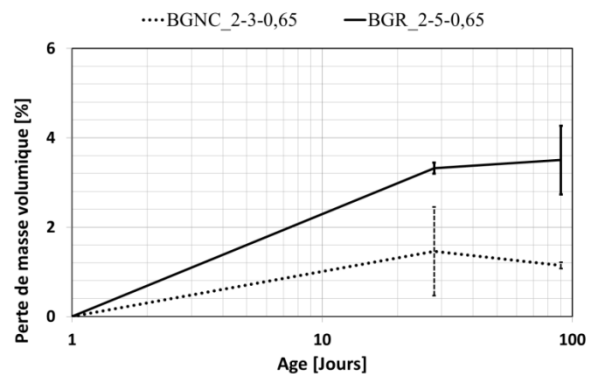
Figure 47 : Perte de masse volumique des bétons non adjuvés par rapport à la valeur à 1 jour
