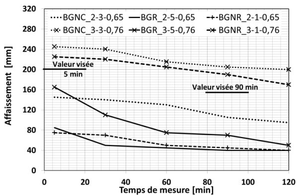
Figure 44 : Evolution de l'ouvrabilité des bétons BGNR, BGNC et BGR non adjuvés
