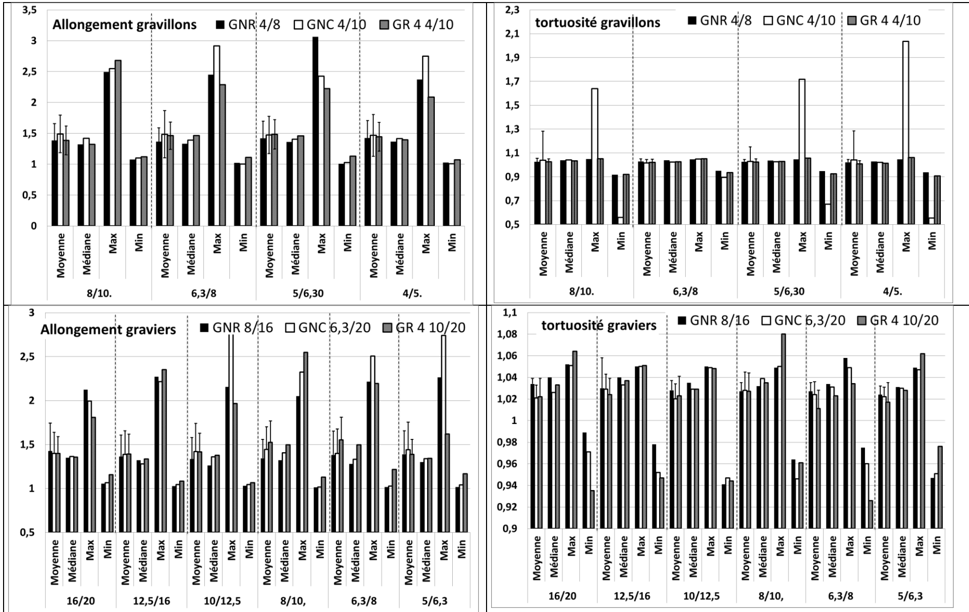
Figure 51 Critères allongement et tortuosité par analyse d'images
