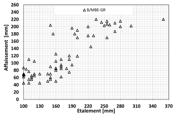
Figure 149 : corrélation des bétons et MBE de GR adjuvantés
