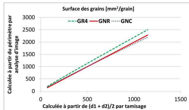
Figure 77 Ecart d'estimation des surfaces spécifiques
