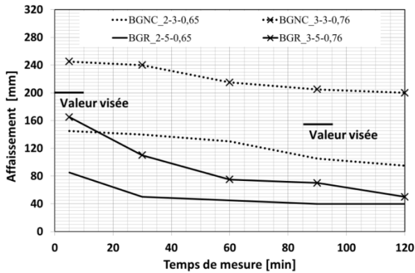
Figure 43 : Evolution de l'ouvrabilité des bétons non adjuvés
