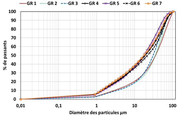
Figure 33 Granulométrie laser, Fraction 0/100µm
