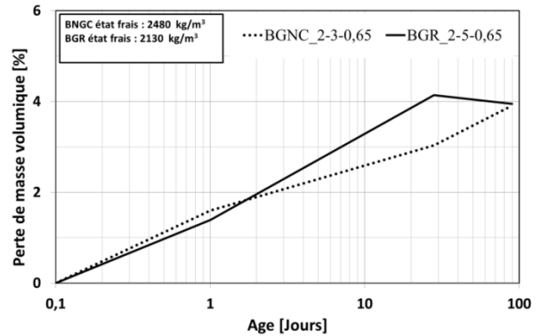
Figure 46 : Perte de masse volumique des bétons non adjuvés par rapport à la valeur à l'état frais
