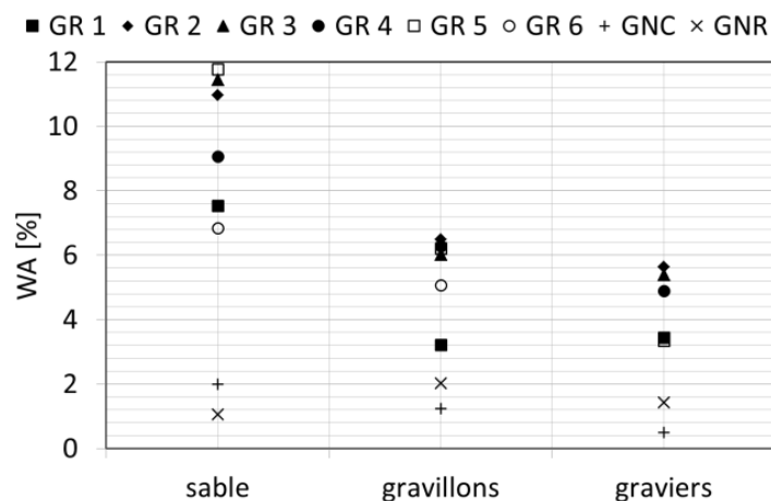
Figure 58 Coefficients d'absorption
