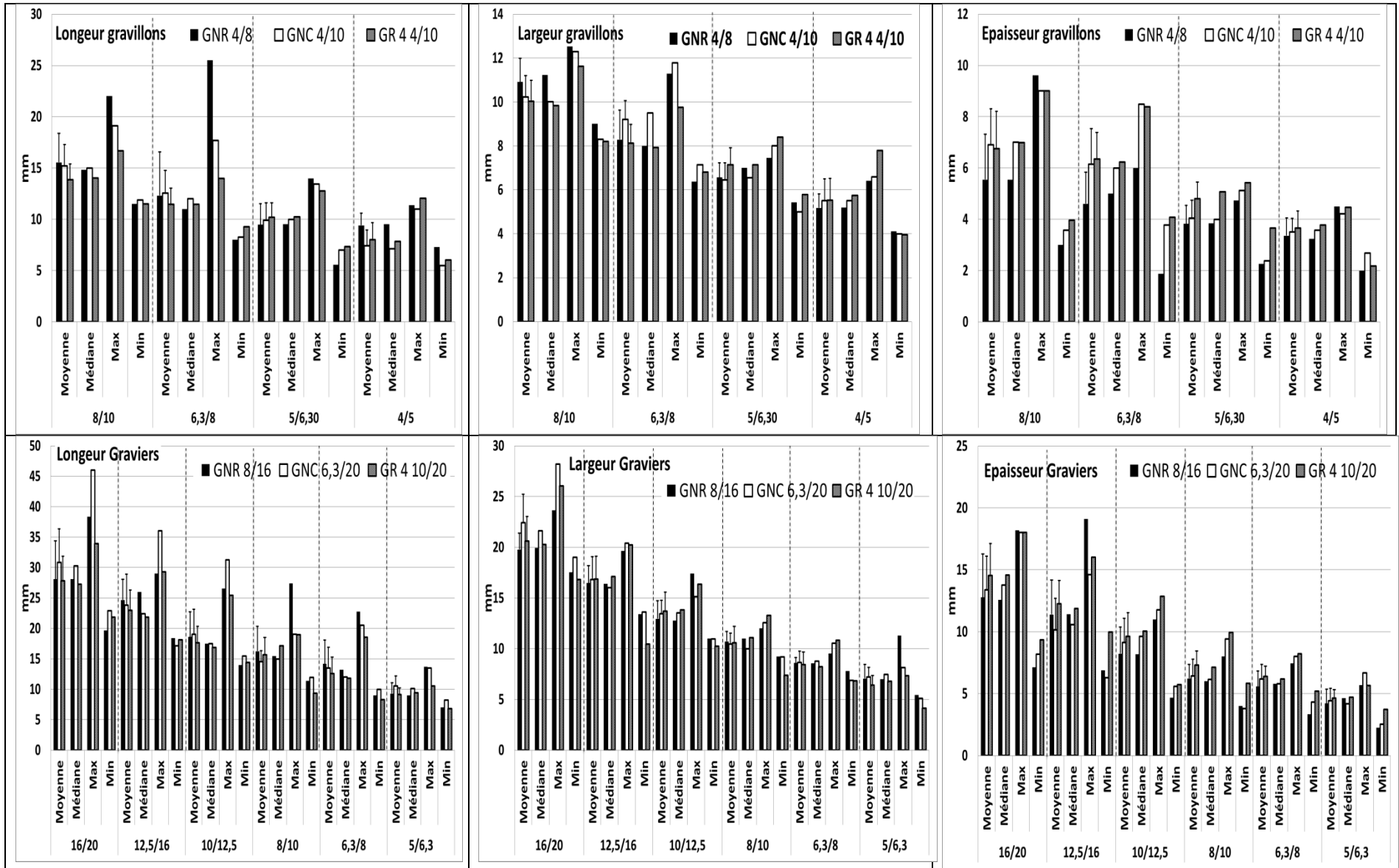
Figure 46 Longueurs, largeurs et épaisseurs par mesure au pied à coulisse
