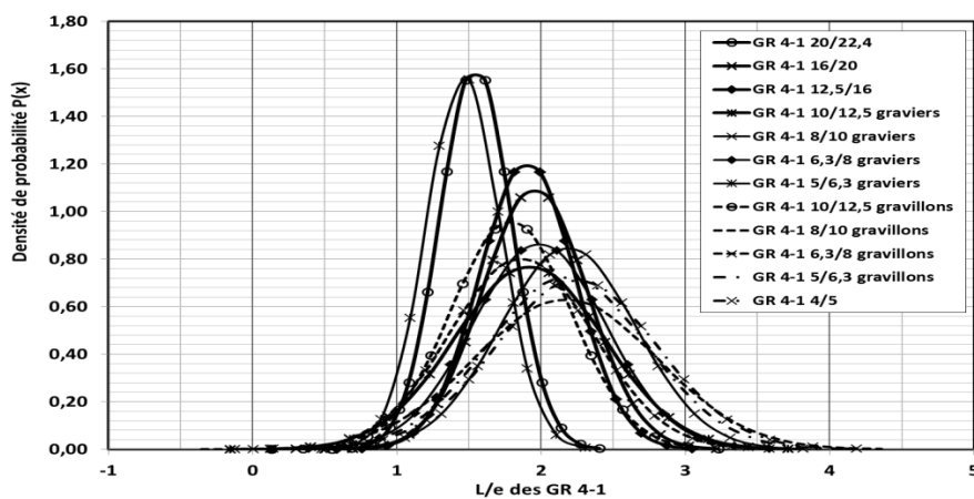
Figure 24: Courbes de Gauss du rapport L/e des GR 4-1 obtenues au pied à coulisse
