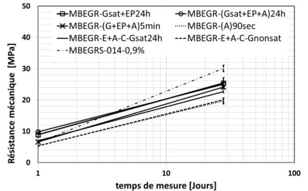
Figure 138 : Résistance mécanique des MBE dont le mode de malaxage a été modifié
