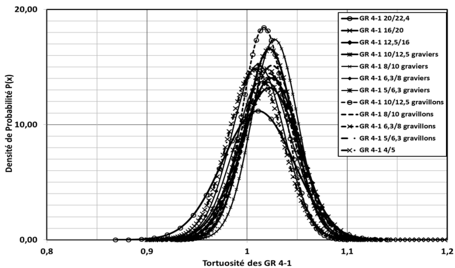
Figure 30: Courbes de Gauss de la tortuosité des GR 4-1 obtenues par analyse d'images
