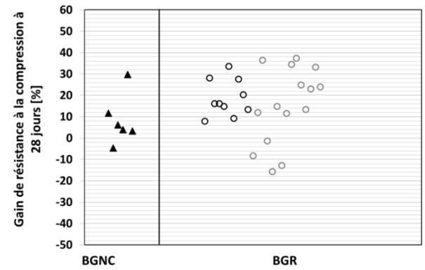
Figure 74 : Gain de résistance mécanique des bétons adjuvantés à 28 jours
