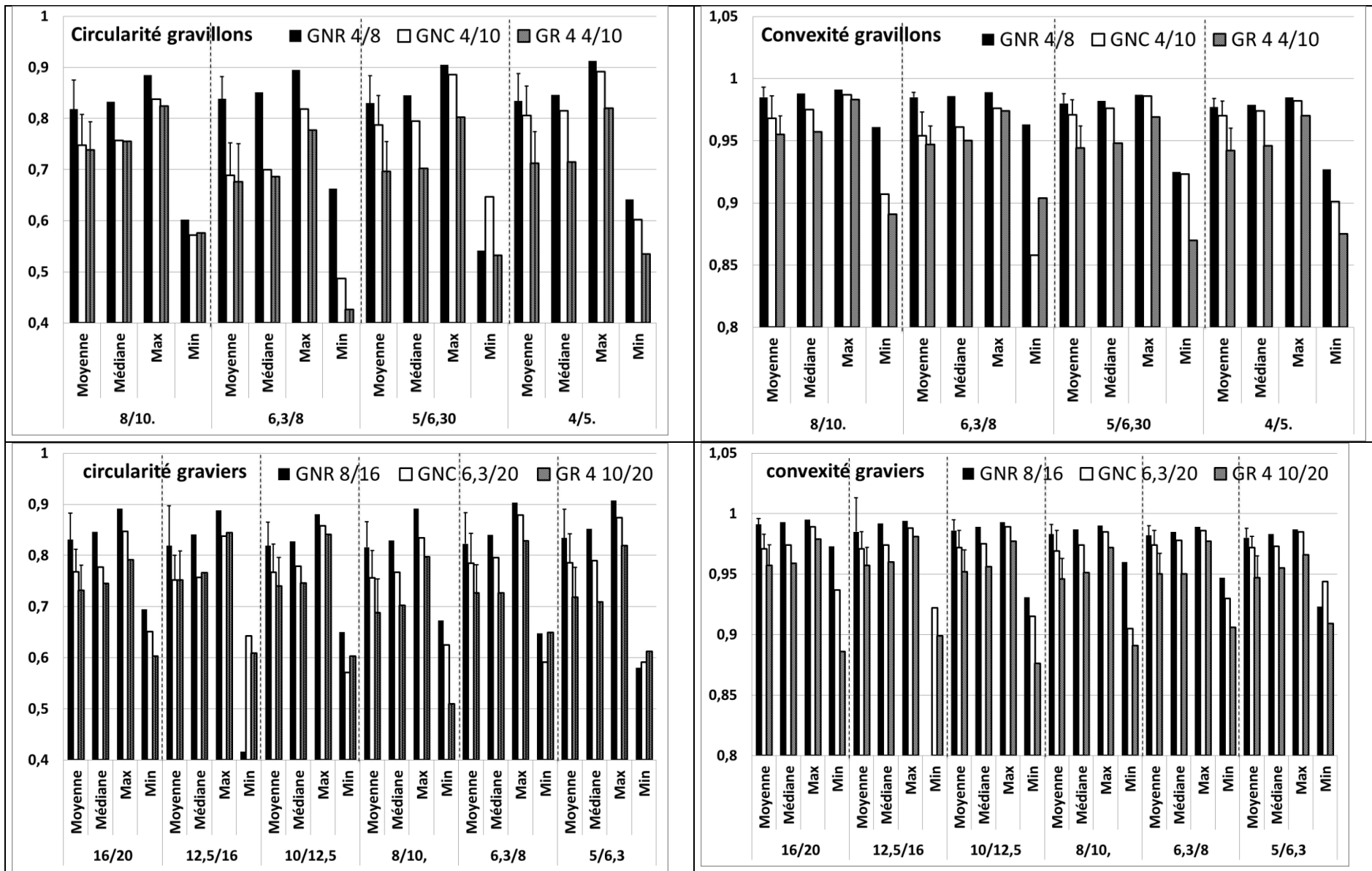
Figure 56 Circularité et convexité par analyse d'images
