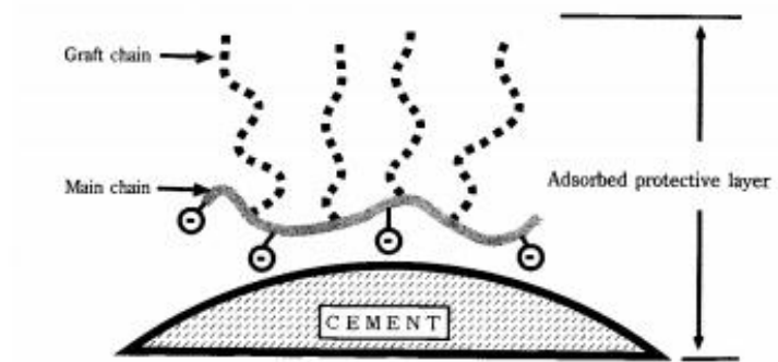
Figure 3 : Représentation schématique d'un polymère dispersant les grains de ciment par effet stérique (d'après Kinoshita et al (1997) dans Martin Cyr, 1999) (Cyr, 1999)
