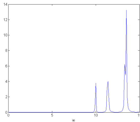
(d) error\_T_{10} for k = 3, h = 0.05
