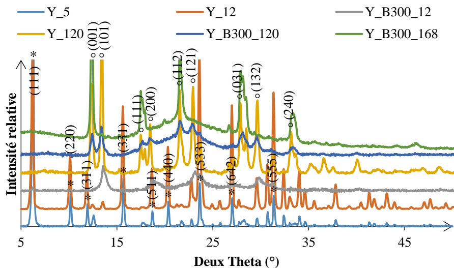
Figure 46 : DRX Y synthétisées dans différentes conditions
