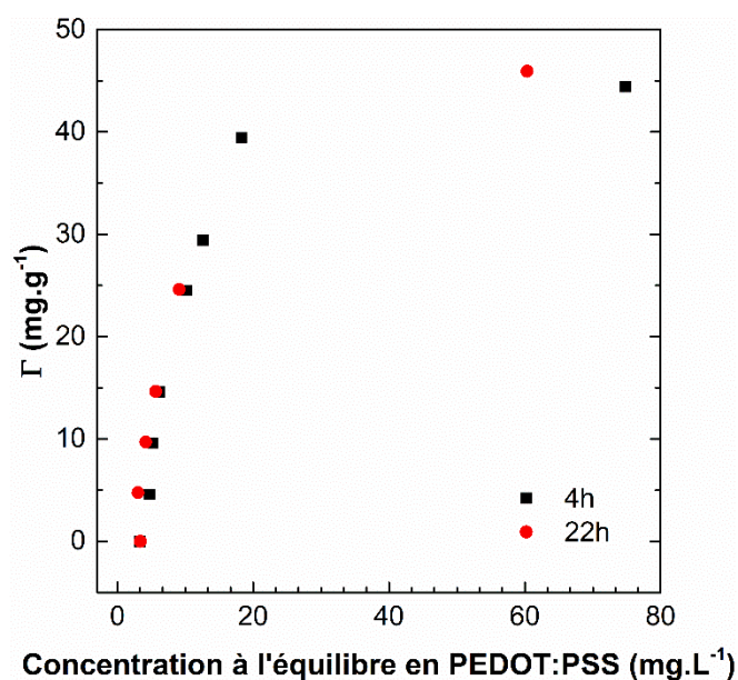
Figure IV-5 : Isothermes d'adsorption du PEDOT:PSS PH sur les particules d'alumine en fonction du temps d'adsorption, pH 3, NaCl 3.10 -3 M.
