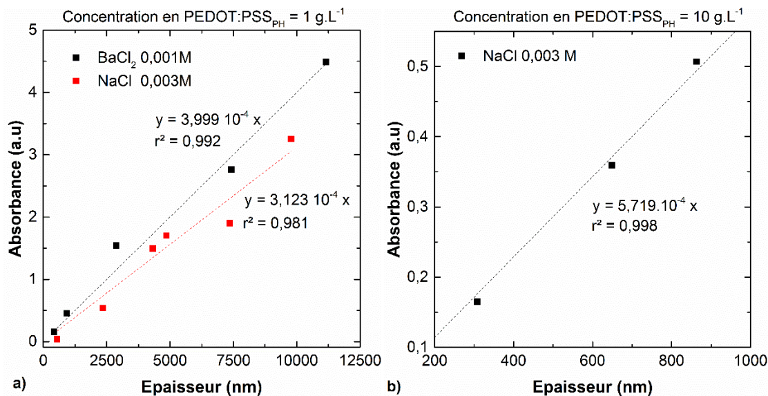
Figure III-11 : Mesure d'absorbance à 930 nm en fonction de l'épaisseur des films multicouches (PDDA/PEDOT:PSS PH ) n , a) films réalisés par dip-coating, b) films réalisés par spin-coating. C PEDOT:PSS 1-10 g.L -1 , C PDDA 1 g.L -1 , pH 5,5.
