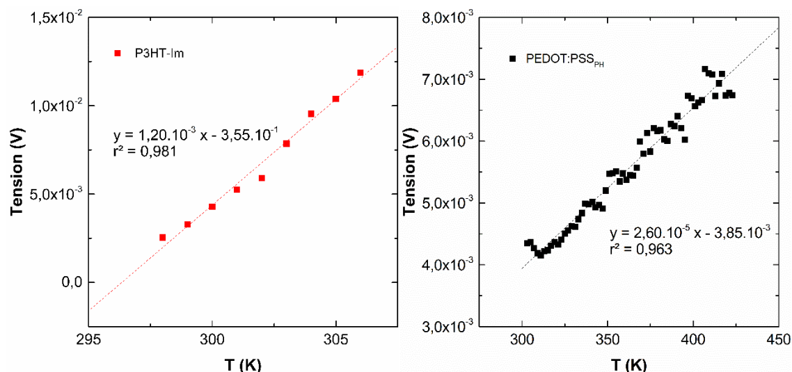
Figure V-11 : Evolution de la tension en fonction d'un gradient de température pour : a) un film drop-casté de P3HT-Im et b) un film drop-casté de PEDOT:PSS PH .
