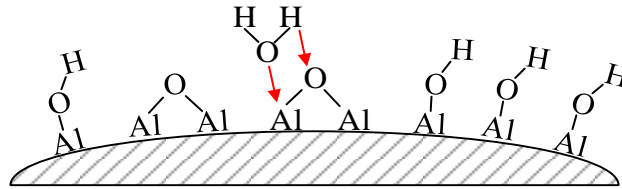
Figure IV-1 : Représentation schématique de la formation de groupements Al-OH.
