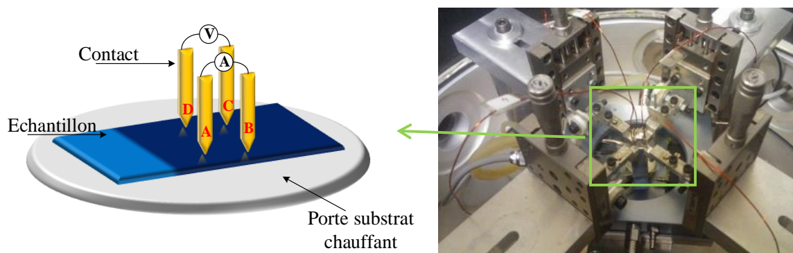
Figure II-15 : L'appareil de mesure de conductivité.
