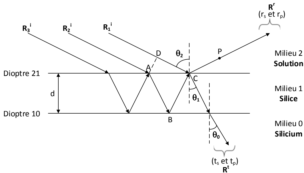
Figure II-9 : Réflexion de la lumière pour un système à deux dioptries.
