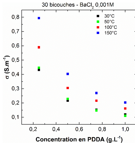
Figure III-23 : Evolution de la conductivité en fonction de la concentration en PDDA pour des films (PDDA/PEDOT:PSS PH ) 30 de 30 bicouches. C_{PEDOT:PSS} 1 \text{ g.L}^{-1} , C_{PDDA} 0,25 - 1 \text{ g.L}^{-1} , BaCl_2 10^{-3} \text{ M} , pH 5,5
