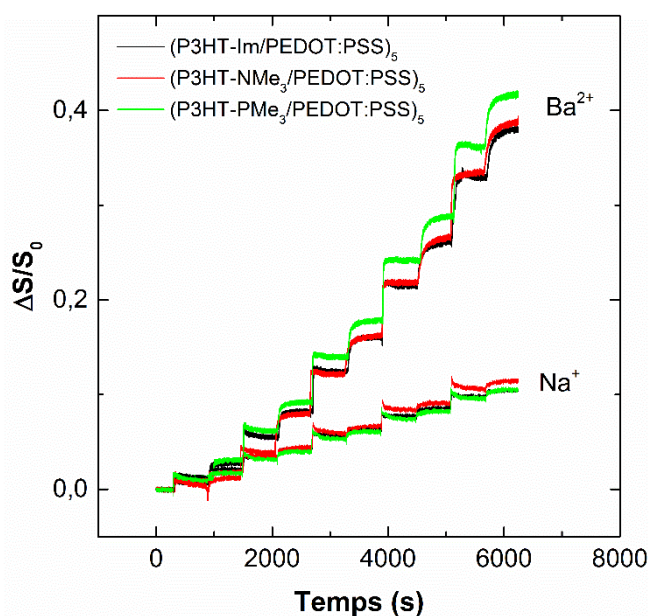
Figure V-2 : Courbes réflectométriques des films (P3HT-R/PEDOT:PSS PH ) 5 en fonction de la nature du sel. NaCl 3.10 -3 M - BaCl 2 1.10 -3 M, Cp 0,01g.L -1 , pH 5,5.
