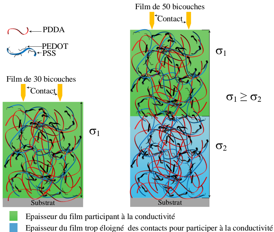
Figure III-20 : Représentation schématique de l'effet de l'augmentation du nombre de bicouches adsorbées sur la conductivité de films multicouches (PDDA/PEDOT:PSS) PH ) n .
