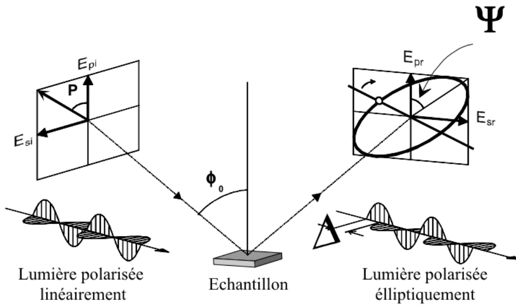
Figure II-10 : Représentation schématique des angles ellipsométriques \Delta et \Psi .
