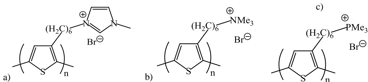
Figure I-7 : Structures des P3HT-R utilisés : a) le P3HT-Im, b) P3HT-NMe 3 , c) le P3HT-PMe 3 .
