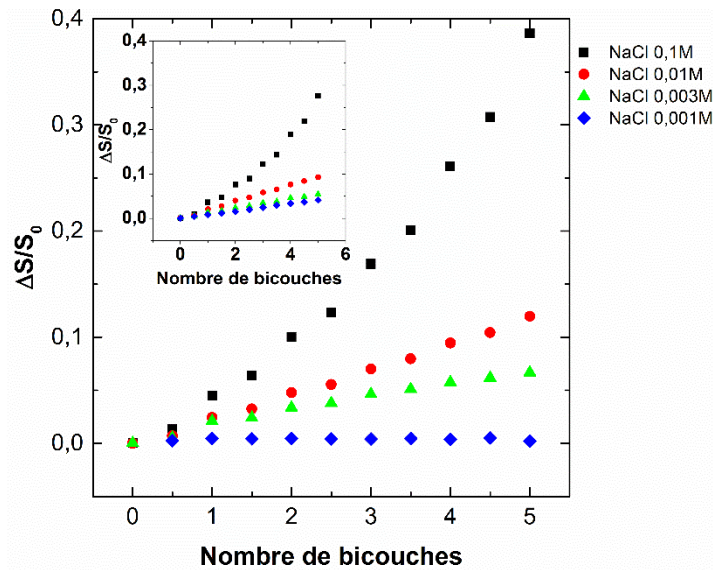
Figure III-3 : Effet de la force ionique sur la croissance d'un film multicouche (PDDA/PEDOT:PSS PH ) 5 et en encadré (PDDA/PEDOT:PSS 8000 ) 5 . Concentration en NaCl : ♦:10 -3 , ▲:3.10 -3 , ●:10 -2 et ■:10 -1 M, Cp 0,01 g.L -1 , pH 5,5.
