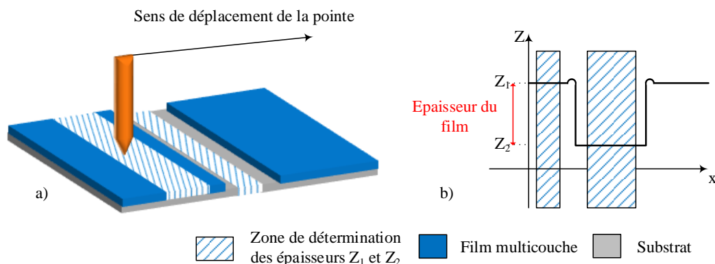
Figure II-11 : a) Représentation schématique de la mesure d'épaisseur par profilométrie, b) profil type de mesure obtenu après passage de la pointe.
