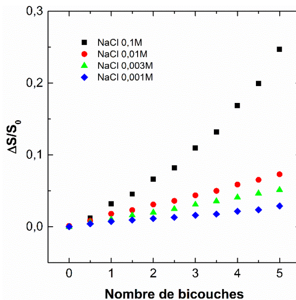
Figure III-4 : Effet de la force ionique sur la croissance d'un film multicouche (PDDA/PSS) 5 . Concentration en NaCl : ♦:10 -3 , ▲:3.10 -3 , ●:10 -2 et ■:10 -1 M, Cp 0,01g.L -1 , pH 5,5.
