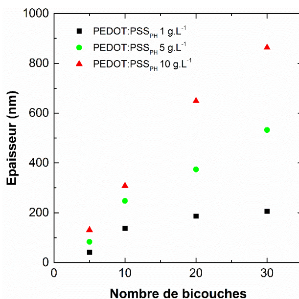
Figure III-10 : Epaisseurs des films de (PDDA/PEDOT:PSS PH ) n mesurées par profilométrie en fonction du nombre de bicouches réalisées par spin-coating, C_{\text{PEDOT:PSS}} 1, 5 et 10 g.L -1 , C_{\text{PDDA}} 1 g.L -1 , pH 5,5, NaCl 3.10 -3 M.
