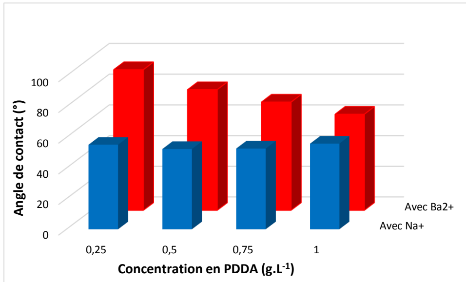
Figure III-26 : Variation des angles de contact en fonction de la concentration en PDDA pour des films de 50 bicouches.
