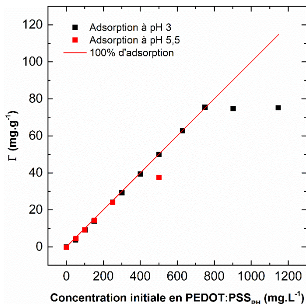
Figure IV-8 : Evolution de la quantité de PEDOT:PSS PH adsorbé par gramme d' Al_2O_3 en fonction de la quantité initiale introduite, pH 3, NaCl 3.10^{-3} M.
