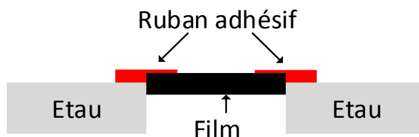
Figure V-7 : Représentation schématique du système de fixation du substrat souple recouvert par le film multicouche.
