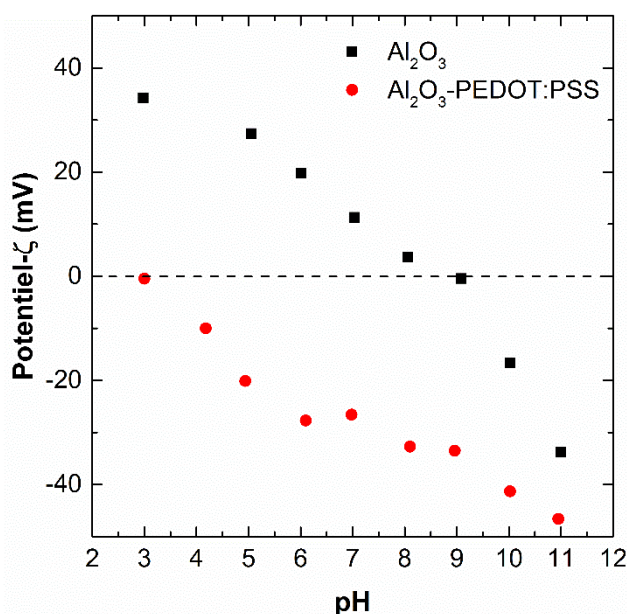
Figure IV-9 : Potentiel- \zeta des particules d'alumine avant et après adsorption du PEDOT:PSS PH , NaCl 3.10 -3 M.
