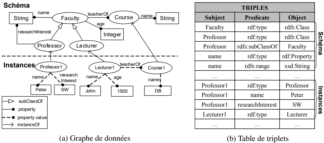
FIGURE 5.1 – Schéma et données utilisés pour les exemples
