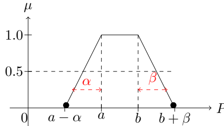
FIGURE 4.3 – Exemple de relaxation de prédicat
