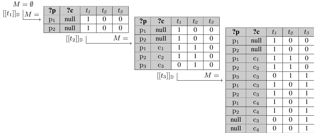
FIGURE 5.8 – Exécution de l'algorithme 3 qui calcule la matrice de relaxation
