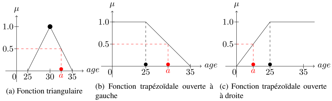
FIGURE 4.2 – Différentes fonctions d'appartenance
