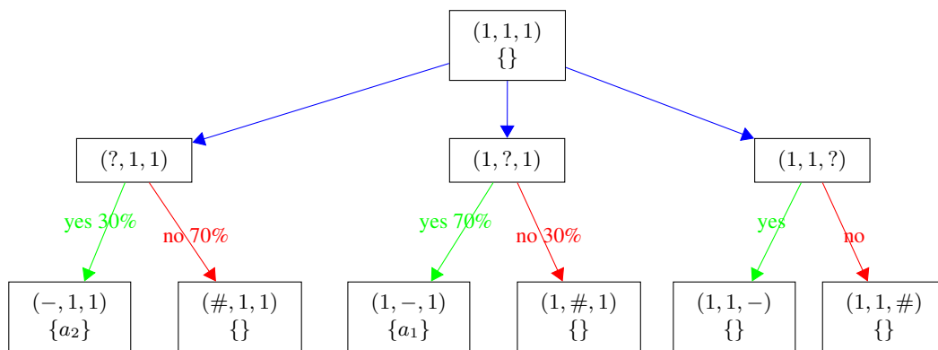
FIGURE 3.5 – Treillis de requêtes relaxées par suppression
