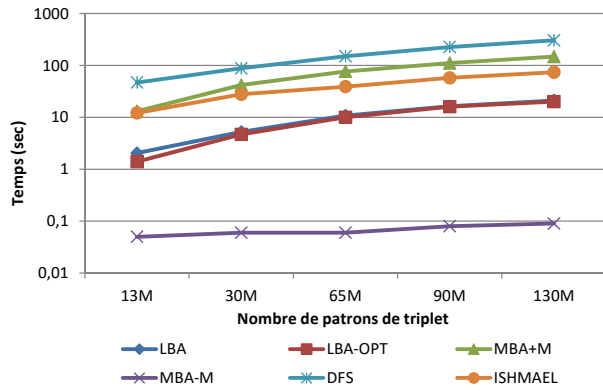
FIGURE 5.13 – Temps de réponse vs taille du jeu de données, requête 15PT
