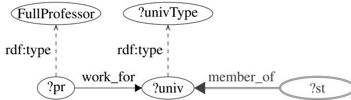
FIGURE 1.10 – Exemple de requête SELECT
