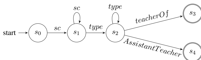
FIGURE 3.11 – Requête SPARQL avec chemin sous forme d'automate fini non-déterministe
