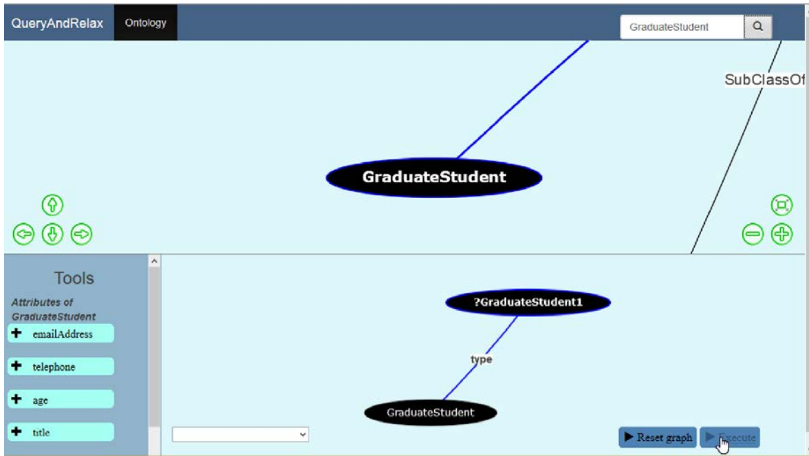
FIGURE 4.5 – Construction d'une requête SPARQL
