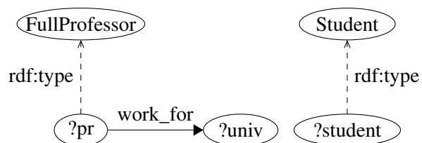
FIGURE 1.8 – Produit cartésien entre patrons de triplets
