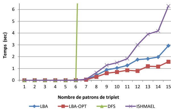
FIGURE 5.16 – Temps de réponse vs taille des requêtes, LUBM100
