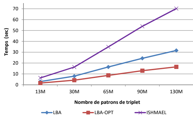
FIGURE 5.17 – Temps de réponse vs taille du jeu de données, requête 15 PT
