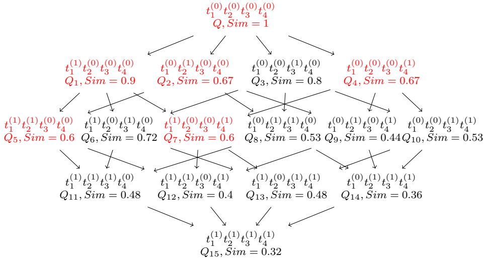
FIGURE 6.4 – Exemple de graphe de relaxations
