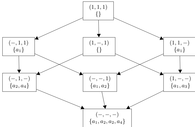
FIGURE 3.4 – Treillis de requêtes relaxées par suppression
