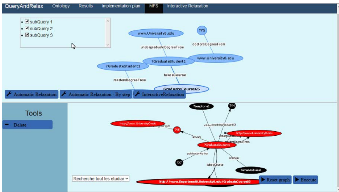
FIGURE 5.11 – Recherche des MFSs dans QaRS
