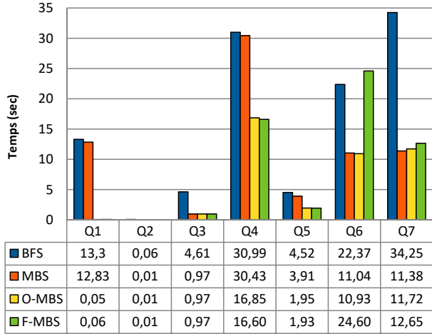
FIGURE 6.7 – Coût en temps sur Jena TDB
