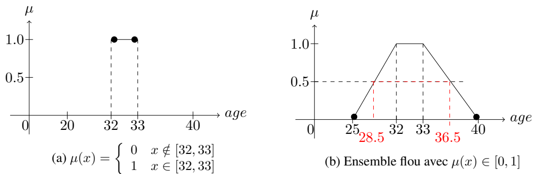
FIGURE 3.1 – Fonction d'appartenance pour un ensemble classique (a) et flou (b)
