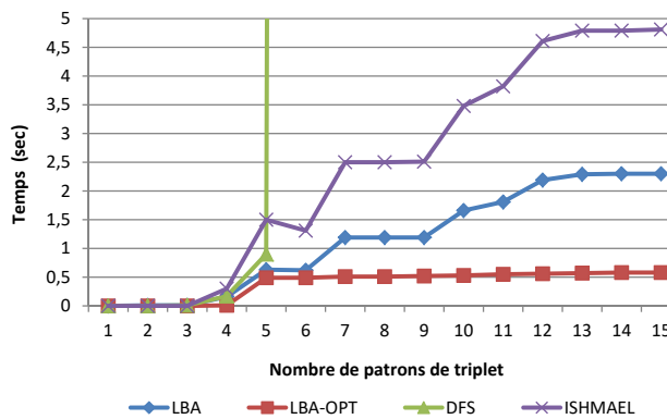
FIGURE 5.14 – Temps de réponse vs taille des requêtes, LUBM100
