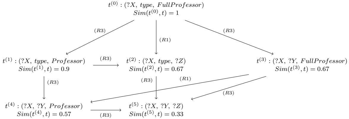
FIGURE 6.2 – Relaxation d'un patron de triplet
