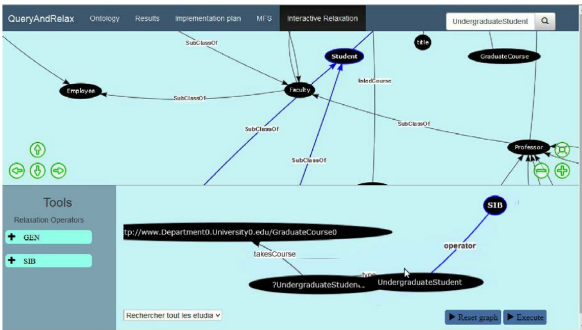
FIGURE 4.6 – Construction d’une requête relaxée
