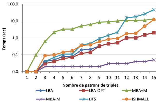
FIGURE 5.12 – Temps de réponse vs taille des requêtes, LUBM100
