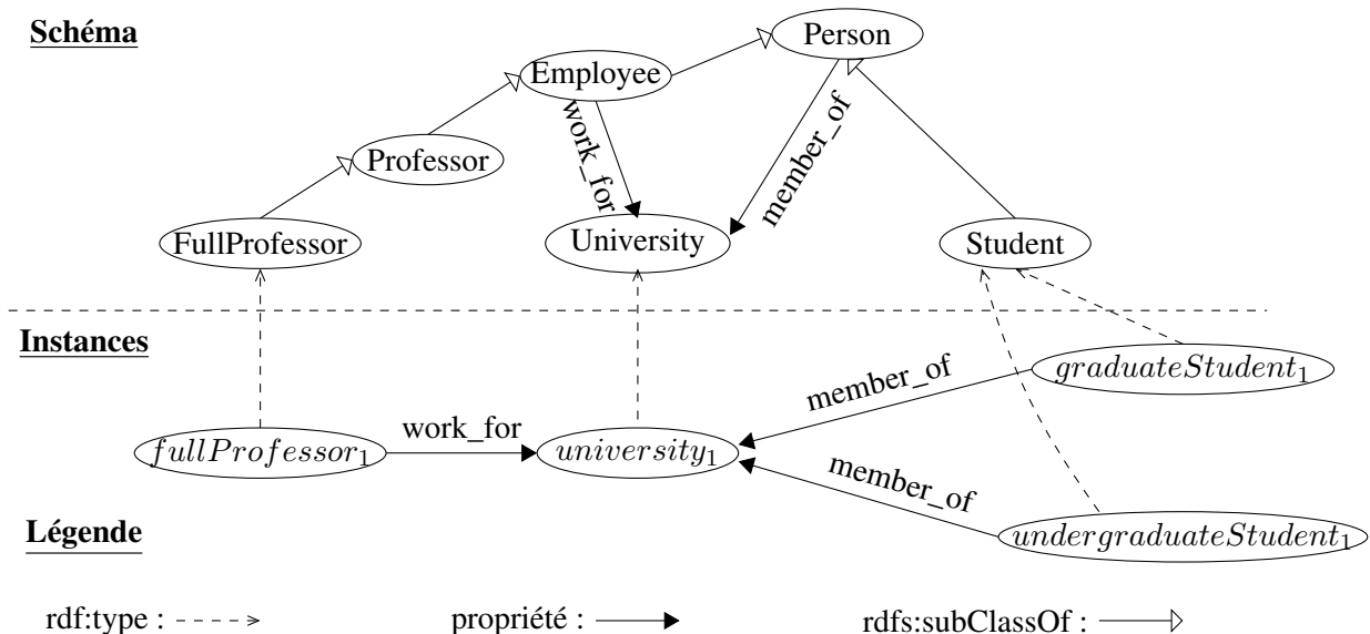
FIGURE 1.2 – Graphe RDF des données et du schéma RDFS associé
