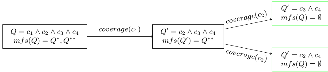
FIGURE 3.9 – Recherche de requêtes relaxées de Q avec Recover
