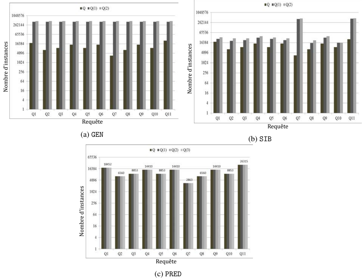
FIGURE 4.10 – Nombre d’instances filtrées pour chaque opérateur de relaxation
