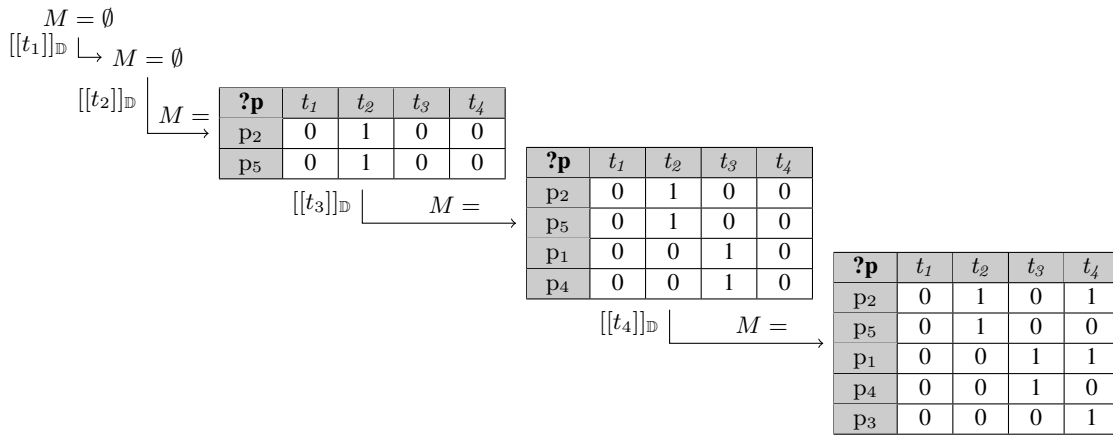
FIGURE 5.10 – Un exemple d'exécution de l'algorithme 4
