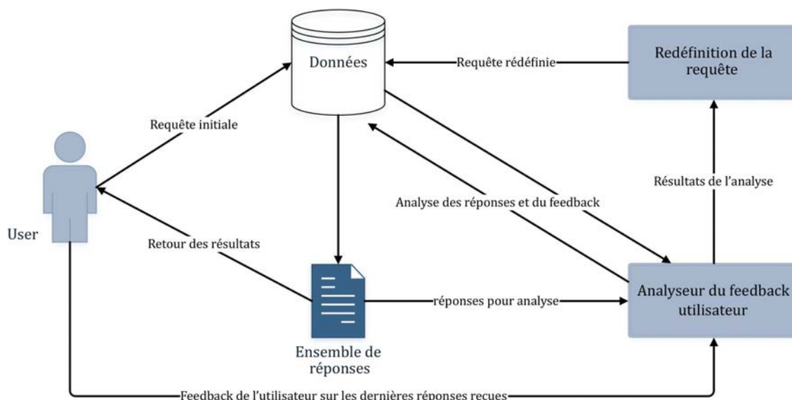
FIGURE 2.2 – Architecture de l'approche coopérative avec Feedbacks utilisateur (inspirée de [148])
