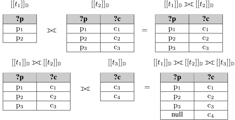
FIGURE 5.7 – Opérateur de jointure externe entre des ensembles de mappings
