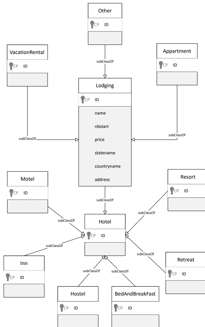
FIGURE 4.8 – Ontologie de logement
