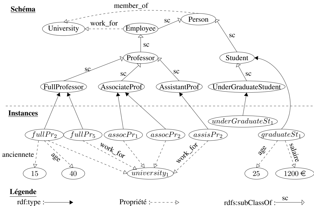
FIGURE 3.10 – Graphe de données
