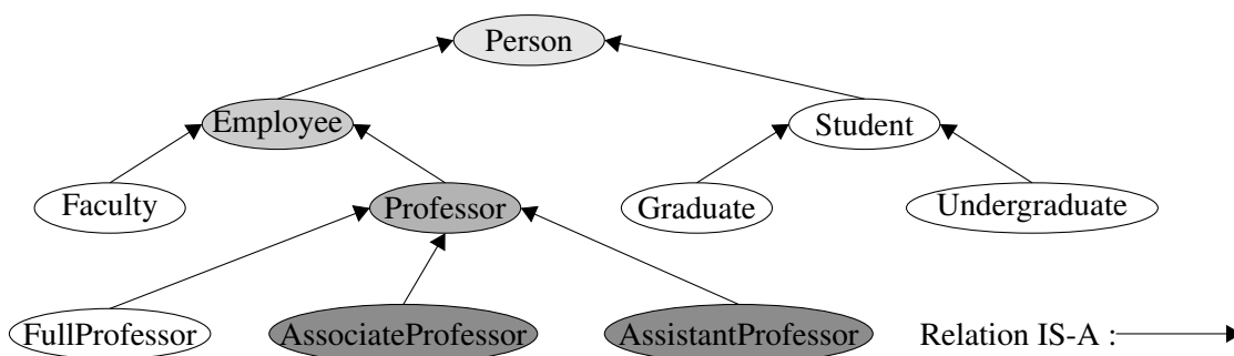
FIGURE 3.6 – Hiérarchie abstraite de types (TAH)
