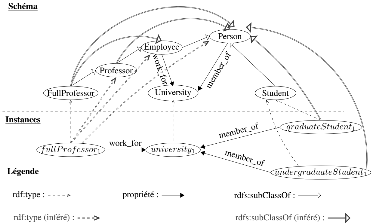
FIGURE 1.6 – Graphe RDF des données RDF saturées
