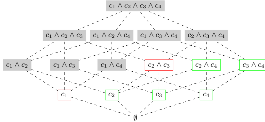
FIGURE 3.8 – Treillis des sous-requêtes de Q
