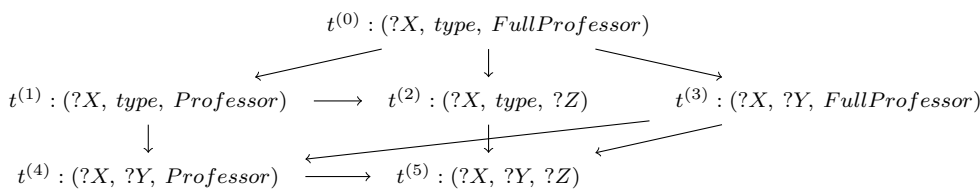
FIGURE 3.12 – Relaxation d'un patron de triplet
