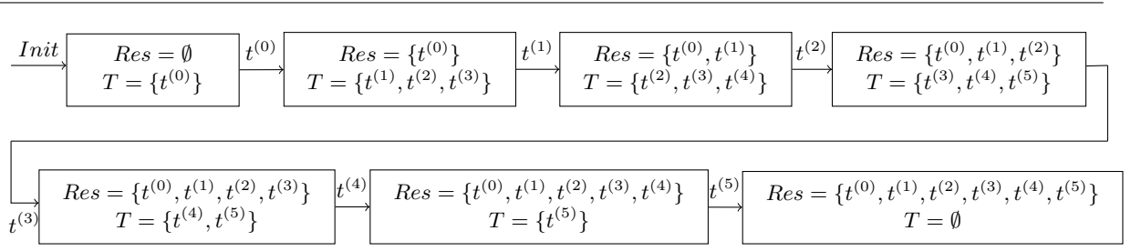
FIGURE 6.3 – Exemple d'exécution de l'algorithme 5 sur un patron de triplet t
