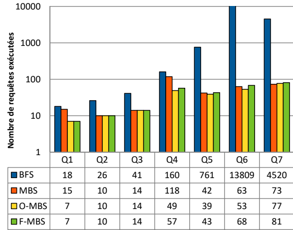
FIGURE 6.8 – Coût en nombre de requêtes
