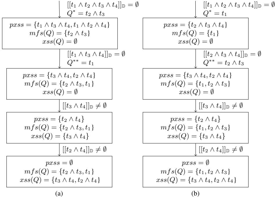
FIGURE 5.5 – Un exemple d'exécution de l'algorithme 2 pour trouver les MFS et XSS de Q
