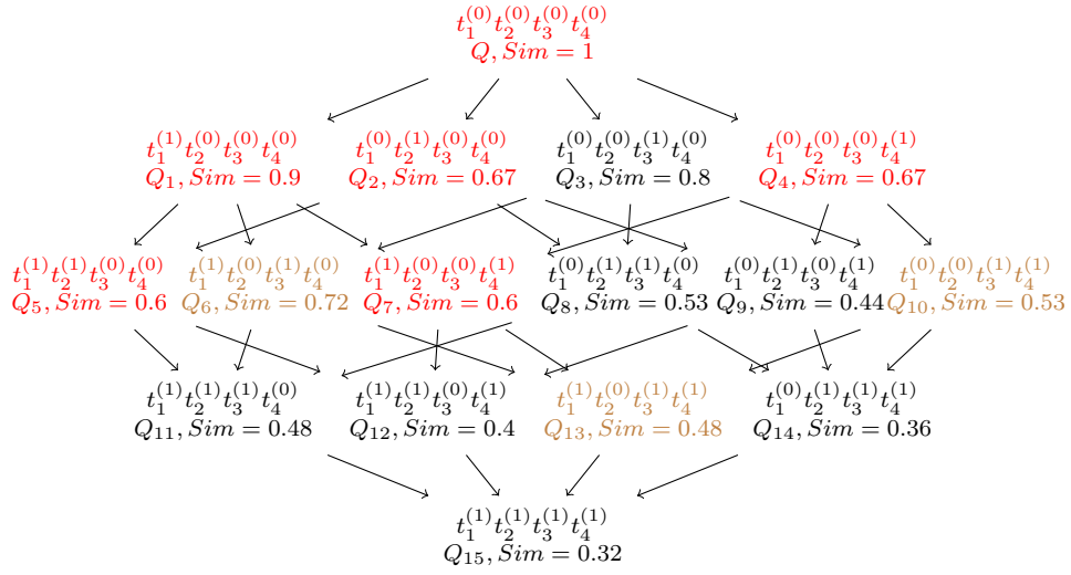
FIGURE 6.6 – Graphe de relaxation exploré avec O-MBS
