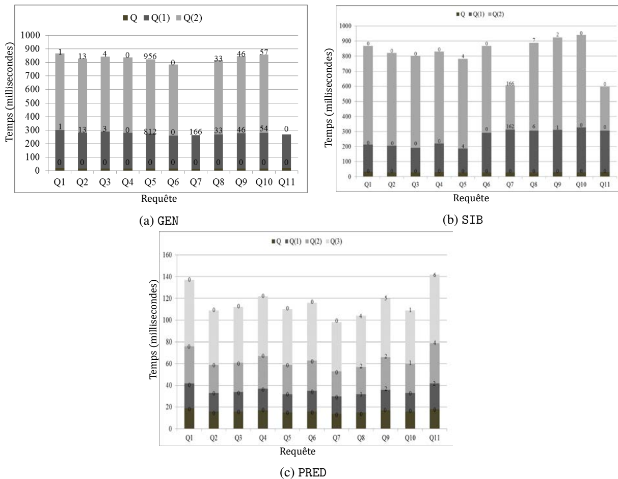
FIGURE 4.9 – Temps d'exécution de la relaxation et nombre des réponses alternatives retournées
