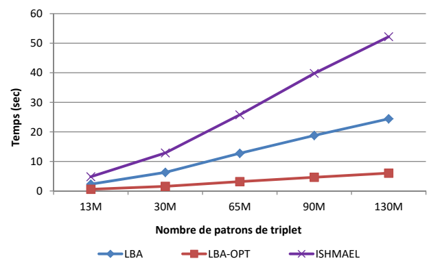
FIGURE 5.15 – Temps de réponse vs taille du jeu de données, requête 15 PT
