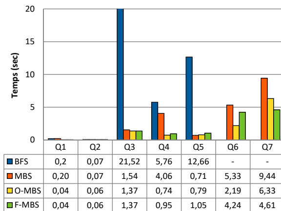
FIGURE 6.9 – Coût en temps sur Virtuoso
