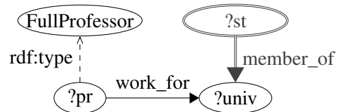
FIGURE 1.9 – Patron de graphe avec OPTIONAL
