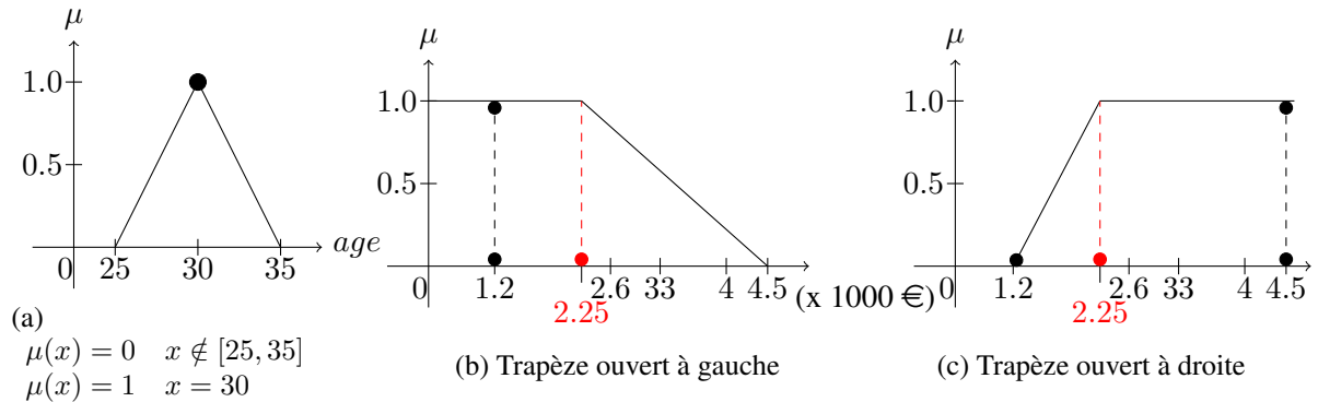
FIGURE 3.2 – Autres formes de fonctions d'appartenance
