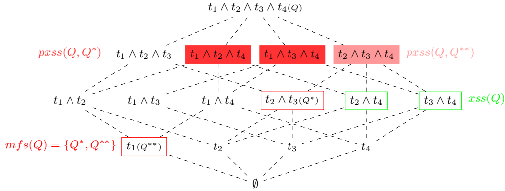
FIGURE 5.4 – Le treillis des sous-requêtes de Q avec ses MFS et XSS
