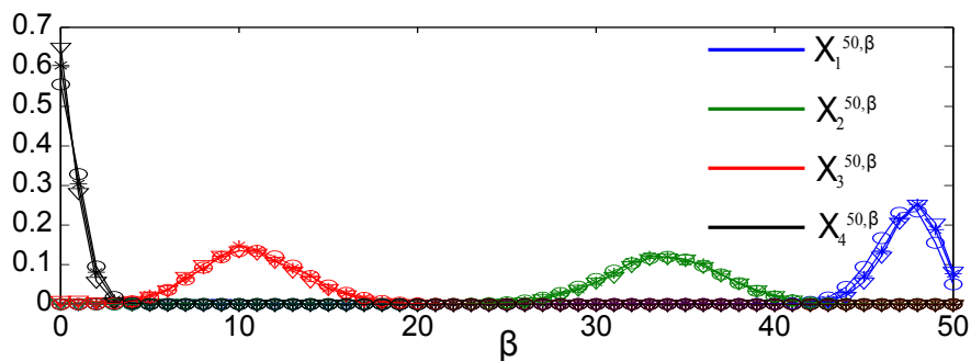
FIGURE 8: Valeurs de \bar{X}_{\theta}^{50, \beta} à la fin de la simulation: les cercles sont les valeurs théoriques obtenues à partir de ((13)), les triangles sont les résultats de la simulation à l'aide du Reality , et les croix sont des résultats de simulation à l'aide du Infocom05 .
