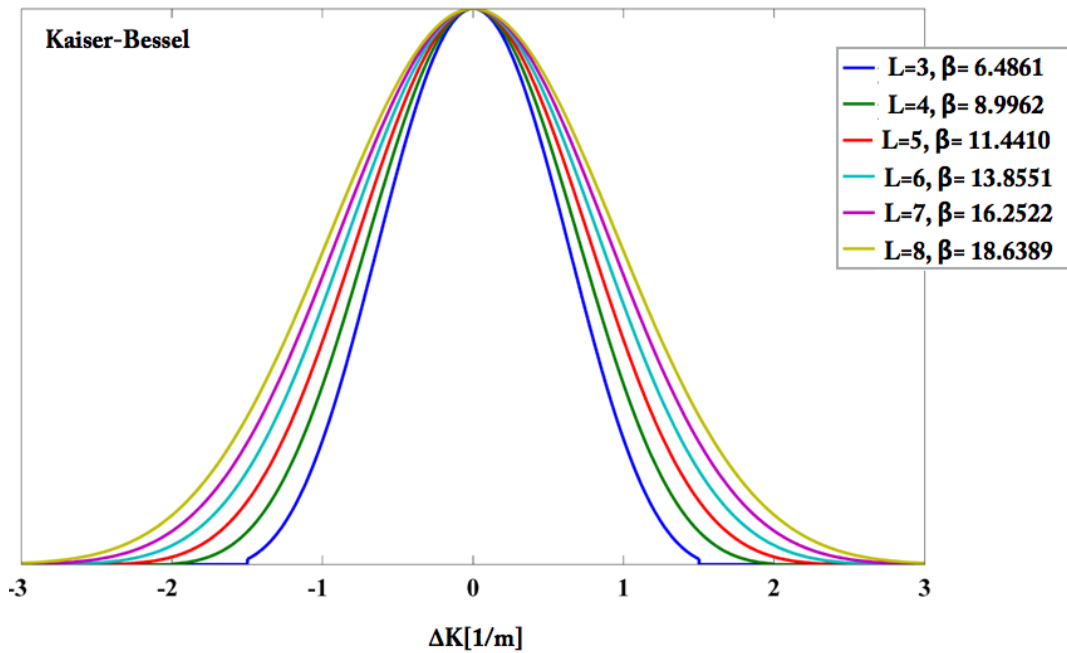
Figure 2.10. Kernel de Kaiser-Bessel avec différentes combinaisons de taille ( L ) et de forme ( \beta ).
