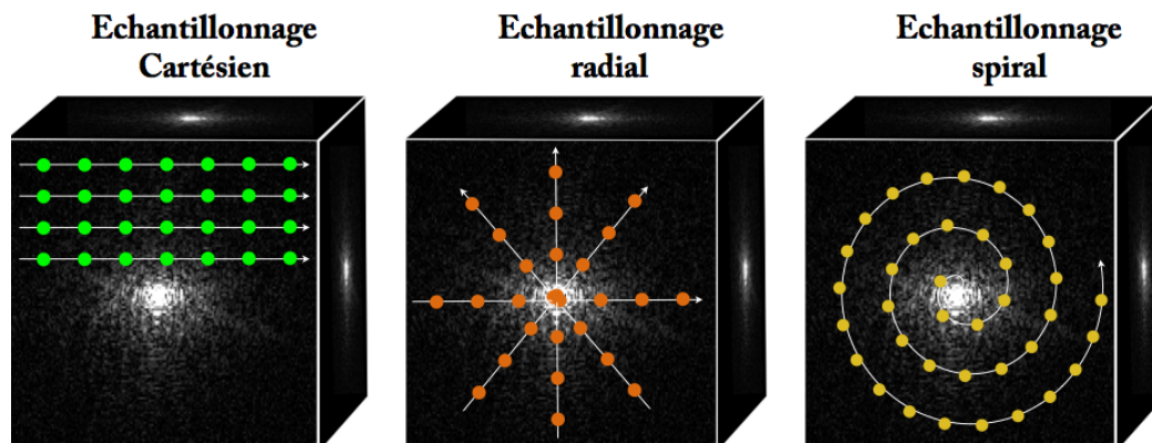
Figure 2.5. Les trois méthodes principales d'échantillonnage de l'espace de Fourier.
