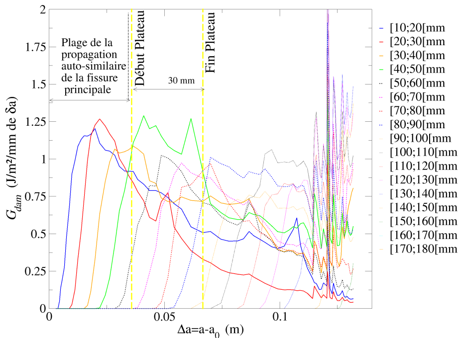
FIGURE 4.32 – Évolution du taux local de restitution d'énergie G_{dam} dans chaque bande h_{tr}=10 \text{ mm} - WST 300 #4
