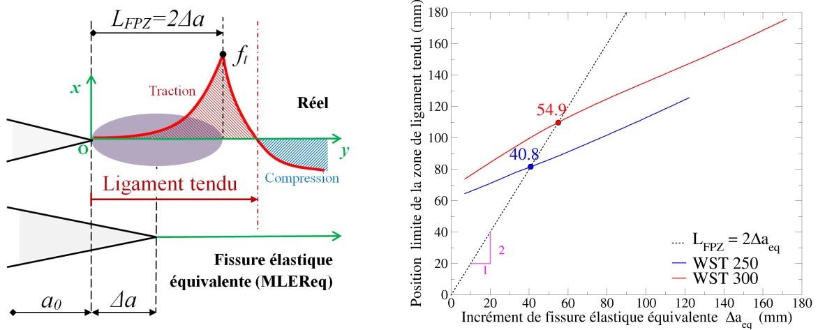
(a) Répartition théorique de la contrainte \sigma_{xx} le long du ligament (étude EF élastique cf Figure 3.13)
