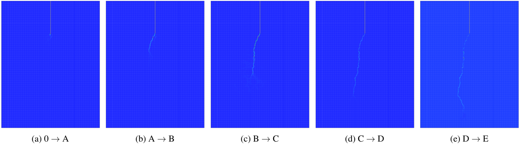
FIGURE 3.23 – Champs des énergies restitué à différents moments de la simulation
