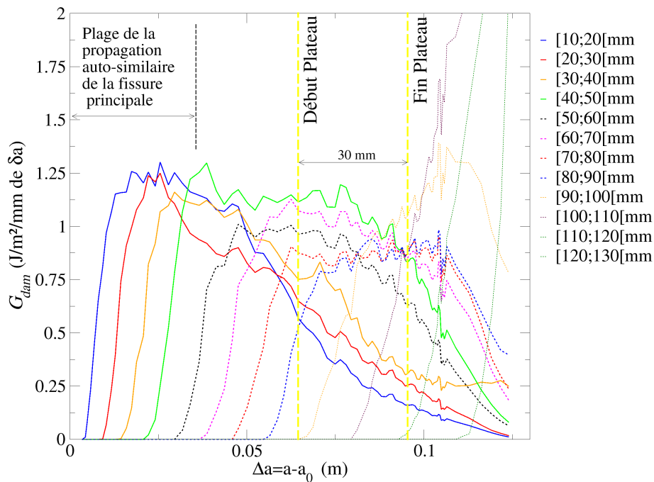
FIGURE 4.31 – Évolution du taux local de restitution d'énergie G_{dam} dans chaque bande h_{tr}=10 \text{ mm} - WST 250 #2
