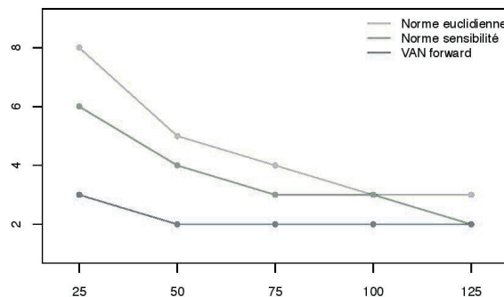
FIGURE 4.11 – Vitesses des convergences (en nombre d'itérations de l'algorithme par valeur de M fixée), pour différents critères d'adversité
