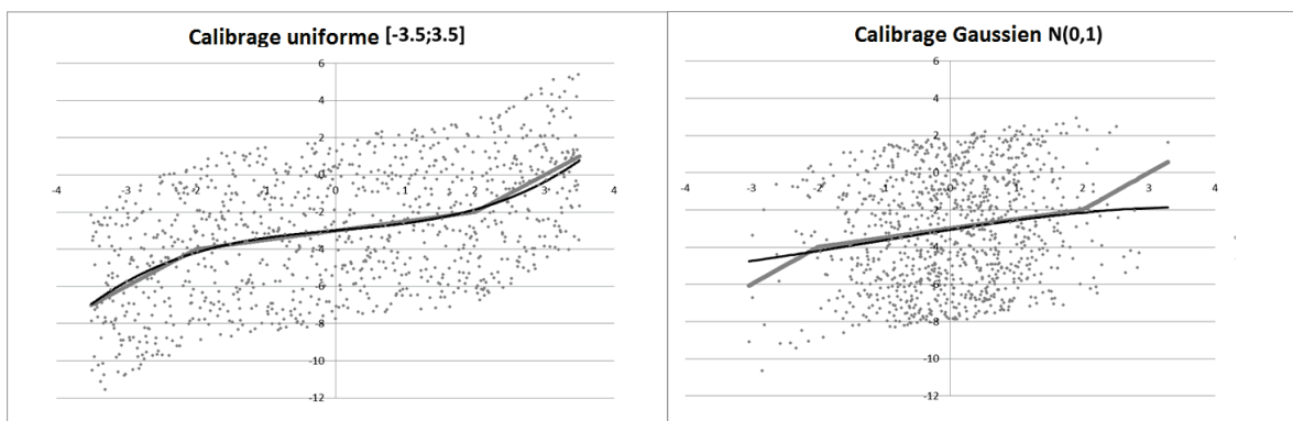
FIGURE 11 – Exemple où x est scalaire, cadre homoscedastique sous exogénéité faible - calibrage du proxy Gaussien (vraie distribution) vs. calibrage uniforme sur [-3,5;3,5] (VAN : points gris, vraie fonction FP : courbe grise épaisse, proxy : ligne noire)
