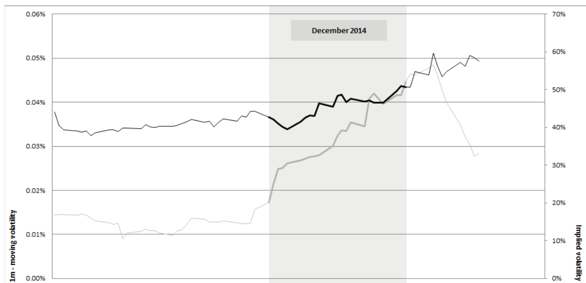
FIGURE 16 – Statistiques observées sur la volatilité implicite de swaption maturité 5 / ténor 5 - noir : volatilité mobile 1 mois entre le 15/10/14 et le 15/01/15 - gris : volatilité implicite entre le 15/10/14 et le 15/01/15
